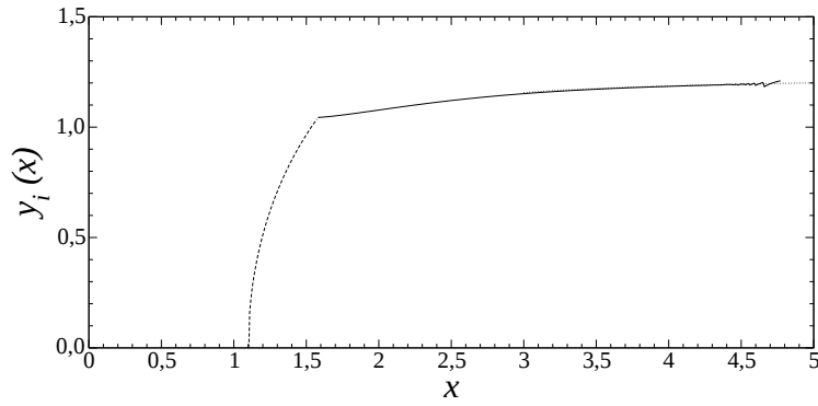
FIG. B.3 – Tracé des points d'inversion y_i(x) en fonction de x . La courbe en trait plein est résultat de l'évaluation numérique de l'équation (B.72), qui montre quelques fluctuations dûes aux erreurs d'arrondi au voisinage de x \sim 4.7 , la courbe pointillée est le prolongement asymptotique (B.76) pour 3 < x < 5 , et la courbe en traits pointillés représente (B.73).
