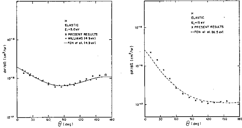
FIG. A.1 – Sections efficaces différentielles de collision électron-atomes neutres expérimentales. Elle sont issues de Shyn et al. [104]. La figure de gauche est typique pour les énergies E < 10 \text{ eV} , et la figure de droite est typique des énergies E > 10 \text{ eV} .
