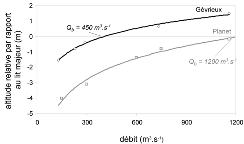
Figure 2.38 – Exemple de courbe hauteur/débit et d'estimation du débit de connexion pour les placettes de Planet et Gévrioux, Q_b = débit de débordement
