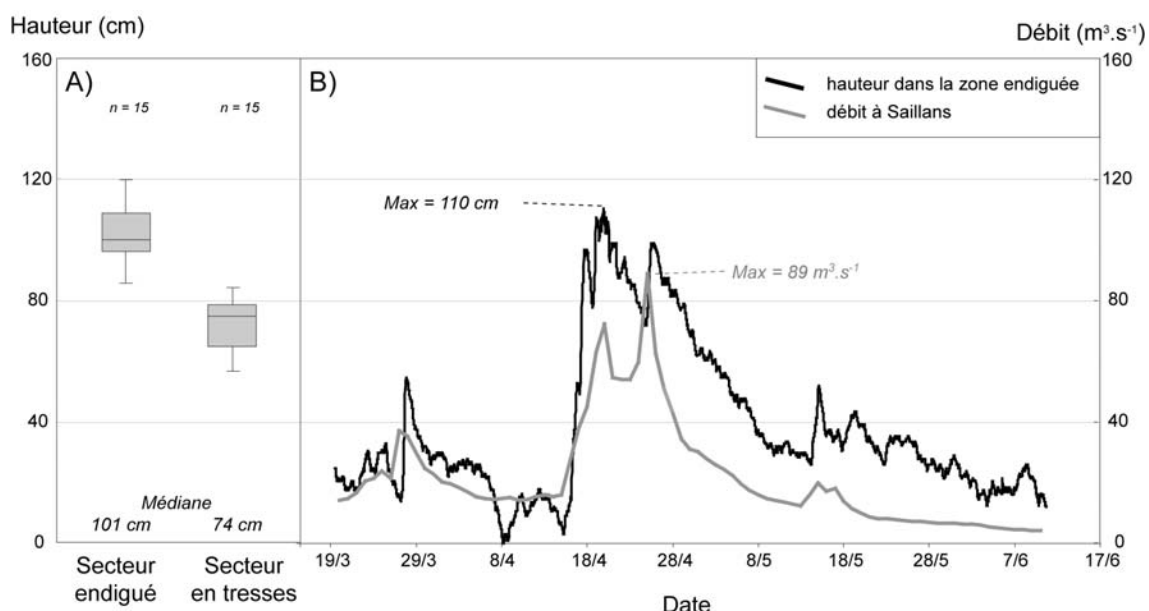
Figure 3.18 – Comparaison hydrologique entre le secteur en tresses et le secteur endigué pour un événement, A) hauteur des laisses de crue, B) suivi hydrologique en continu
