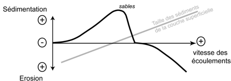
Figure 3.10 – Variabilité des processus de sédimentation et d'érosion des sédiments sableux en fonction de la vitesse du courant
