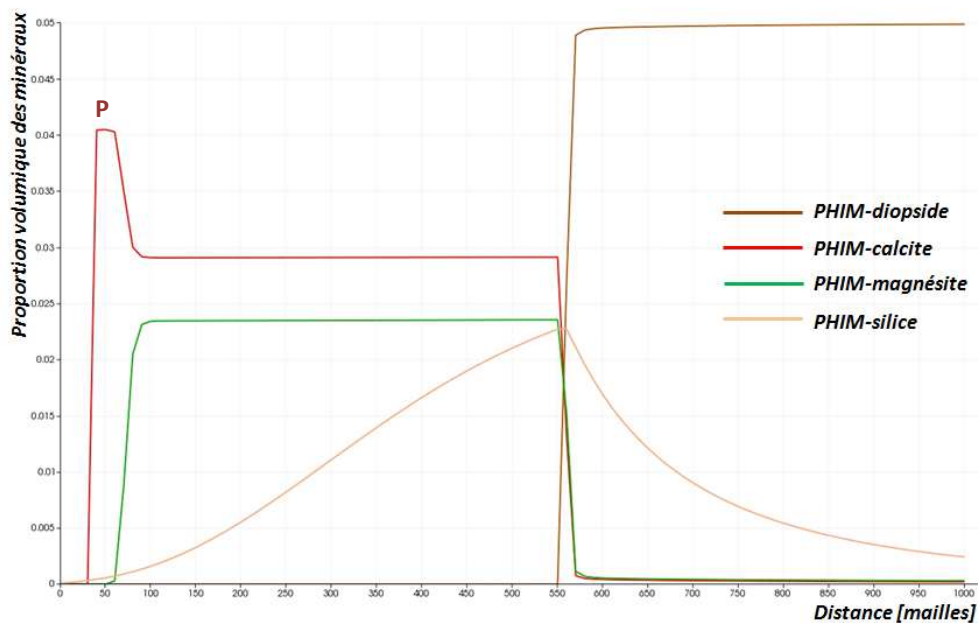
Figure 8: Profil de dissolution/précipitation des minéraux dans le cas homogène (à 180000 jours). La vitesse du fluide vaut 5 m.an -1
