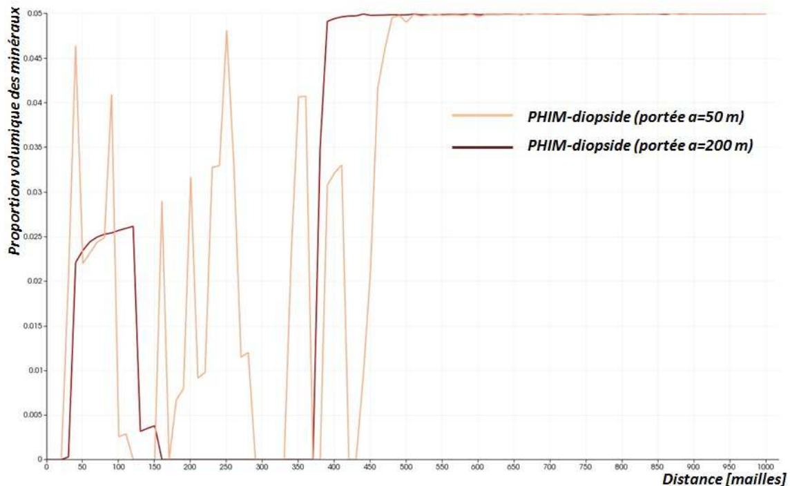
Figure 23: Comparaison des profils de dissolution du diopside à 108000 jours dans le cas de perturbation de kS , avec des portées a_1=50 m et a_2=200 m et de même variance \sigma^2=0.44 . La vitesse du fluide est égale à 5 \text{ m.an}^{-1} .
