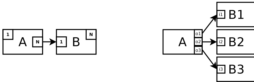
FIGURE 5.9 – Cas N1-1N. À droite la représentation de l’assemblage générique, à gauche un exemple d’assemblage à l’exécution avec trois noeuds clonés. '1'=Simple. 'N'=Répliqué.
