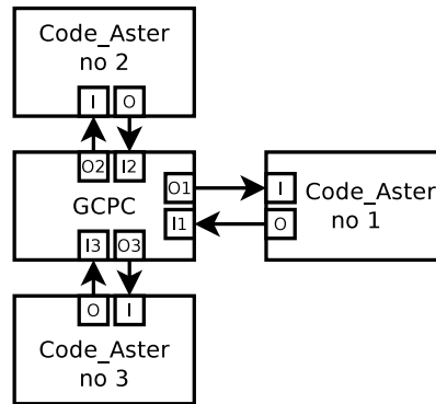
FIGURE 5.6 – Architecture de l’application FETI dans YACS avec trois sous-domaines. I/O : input/output datastream port.
