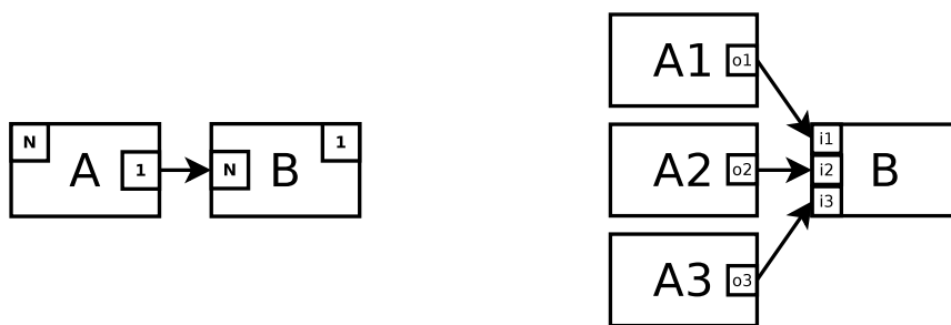
FIGURE 5.10 – Cas 1N-N1. À droite la représentation de l’assemblage générique, à gauche un exemple d’assemblage à l’exécution avec trois noeuds clonés. '1'=Simple. 'N'=Répliqué.
