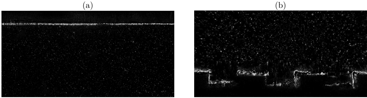
FIGURE 5.22 – Images de PIV après soustraction de l'arrière-plan au voisinage (a) de la plaque lisse et (b) de la zone creux-obstacle. Contraste et luminosité ont été artificiellement augmentés pour une meilleure lisibilité.
