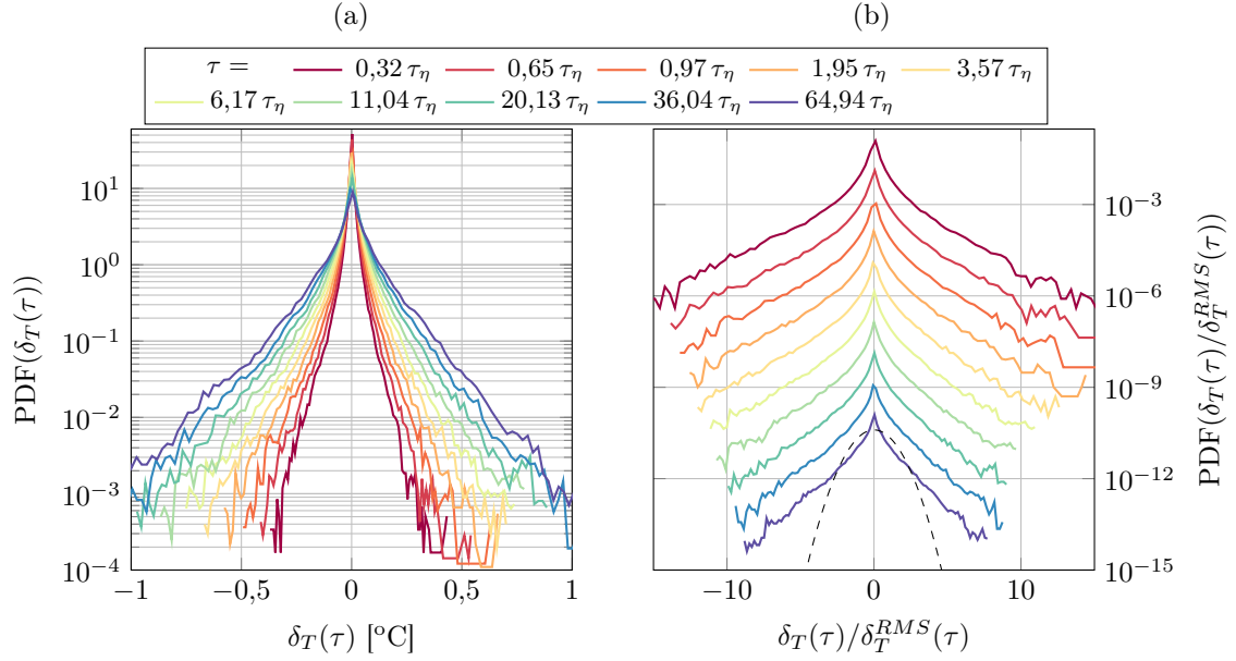
FIGURE 2.21 – PDF des incréments de (a) température et (b) de température normalisée par la moyenne quadratique. Ra = 5,0 \times 10^{10} . La ligne pointillée noire correspond à une gaussienne. Les courbes normalisées sont décalées pour une meilleure lisibilité.
