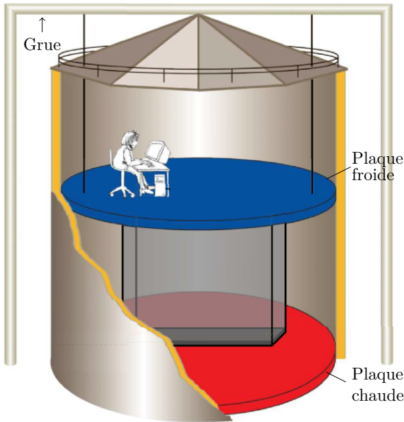
FIGURE 4.10 – Schéma du Barrel of Ilmenau et de la cellule parallélépipédique insérée dedans. Image courtoisement fournie par R. du Puits.
