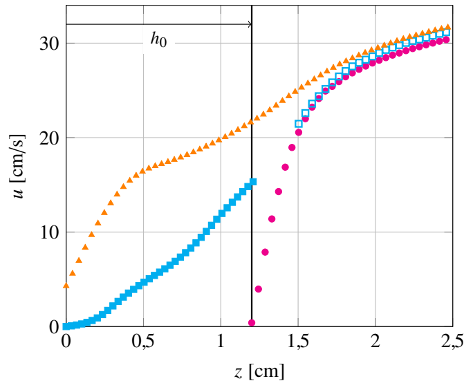
FIGURE 4.18 – Profils de vitesse près de la plaque rugueuse à Ra = 4,04 \times 10^{10} , au-dessus d'un obstacle (cercles magenta), dans le sillon (triangles orange) et dans le creux (carrés cyans pleins pour l'acquisition dans le creux à basse vitesse et vides pour l'acquisition au-dessus du creux à haute vitesse).
