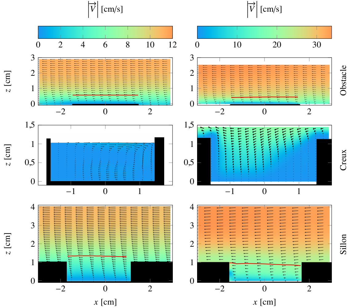
FIGURE 4.16 – Champs moyens de vitesse à Ra = 4,66 \times 10^9 (gauche) et Ra = 4,04 \times 10^{10} (droite). Les trois positions sont représentées de haut en bas : au-dessus d'un obstacle, dans le creux et dans le sillon. L'échelle des flèches est arbitraire de façon à permettre une meilleure visualisation. Les lignes rouges représentent l'épaisseur de déplacement \delta_{déplacement} (voir equation 4.22).
