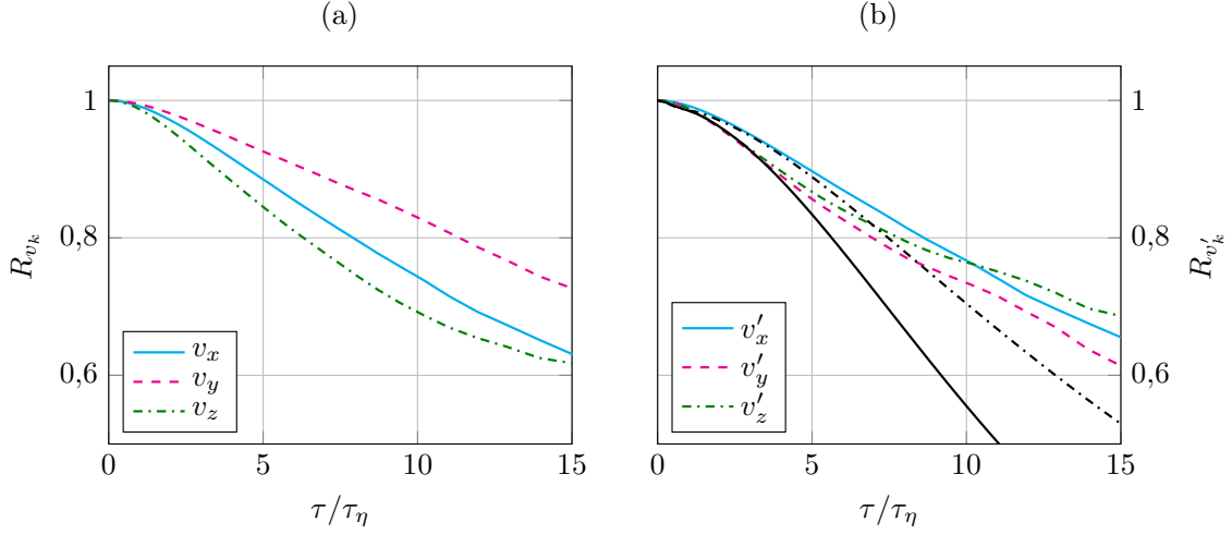
FIGURE 3.22 – Fonctions d'autocorrélation (a) des composantes de la vitesse et (b) des fluctuations correspondantes. La ligne pointillée noire représente la fonction d'autocorrélation des fluctuations de vitesse horizontale obtenue avec le particule instrumentée (chapitre 2), la ligne pleine noire celle pour les fluctuations de vitesse verticale.
