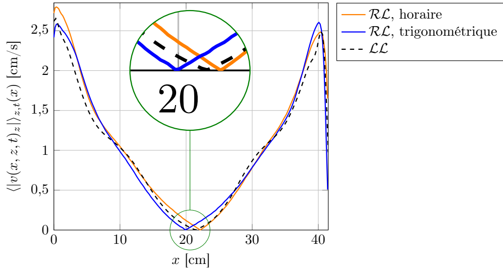
FIGURE 5.3 – Profils des valeurs absolues de la vitesse verticale moyennés dans une bande horizontale centrée de 10 cm de hauteur pour la \mathcal{RL} ( Ra = 7,0 \times 10^{10} ) dans les deux sens de rotation et pour la cellule \mathcal{LL} ( Ra = 6,9 \times 10^{10} ) dans le sens trigonométrique. Les barres d'incertitude n'excèdent pas \pm 0,02 cm/s.
