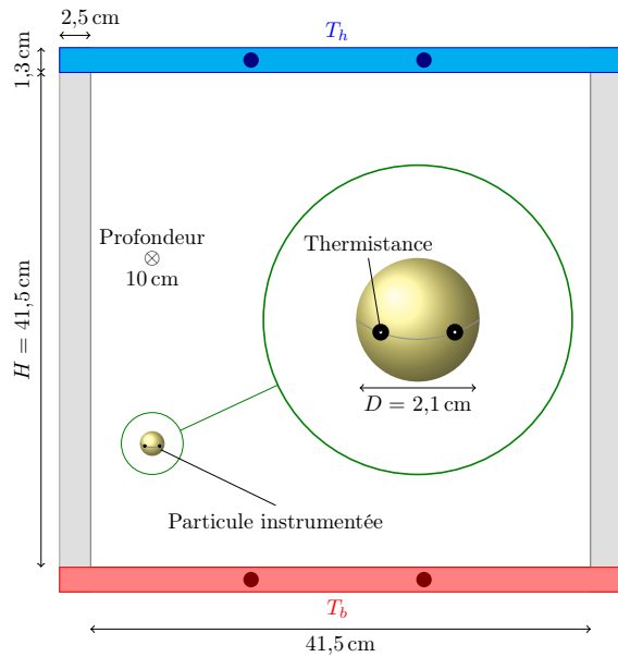
FIGURE 2.1 – Gauche : schéma de principe de la cellule de convection utilisée. Les cercles plus foncés représentent les Pt100 utilisées pour contrôler la température des plaques. La particule instrumentée est représentée à l'échelle de la cellule. Sur le zoom, les points blancs entourés de noir représentent les thermistances entourées de Stycast . Droite : photographie de la particule ouverte. On voit l'emplacement et les contacts qui accueillent les piles.
