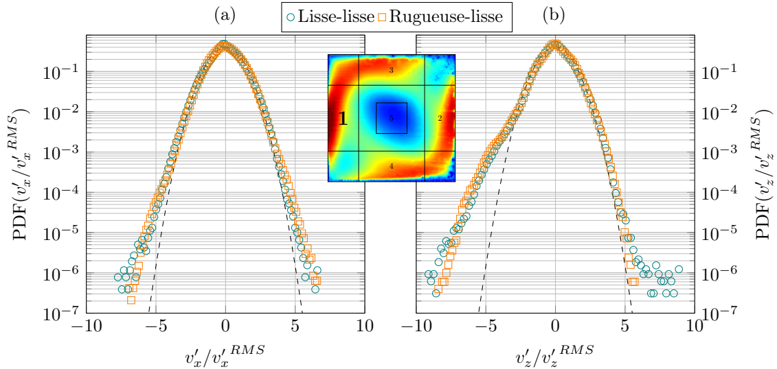
FIGURE 5.11 — Zone 1 — Comparaison des densités de probabilité (PDF) des fluctuations de vitesse (a) horizontale et (b) verticale entre les cellules \mathcal{RL} et \mathcal{LL} pour des nombres de Rayleigh respectifs de 7,0 \times 10^{10} et 6,9 \times 10^{10} . La ligne pointillée représente une distribution gaussienne.
