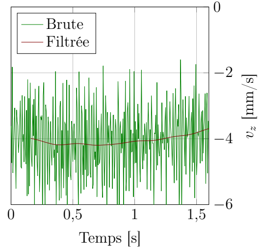
FIGURE 3.10 – Comparaison entre la vitesse calculée par différence finie de la position et celles calculée avec filtrage.
