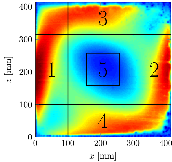
FIGURE 5.8 – Définition des zones pour l'analyse statistique.
