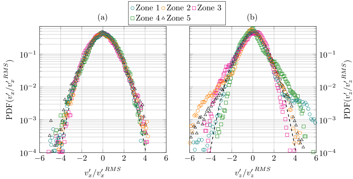
FIGURE 2.33 – Fonctions densité de probabilités des fluctuations des vitesses (a) horizontale et (b) verticale dans chacune des zones, normalisées par la moyenne quadratique correspondante. En pointillé : une distribution gaussienne d'écart-type 1 et de moyenne nulle.
