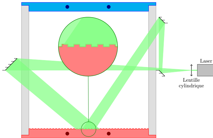
FIGURE 5.20 – Schéma du montage pour l'illumination des différentes zones à proximité des rugosités par la nappe laser.
