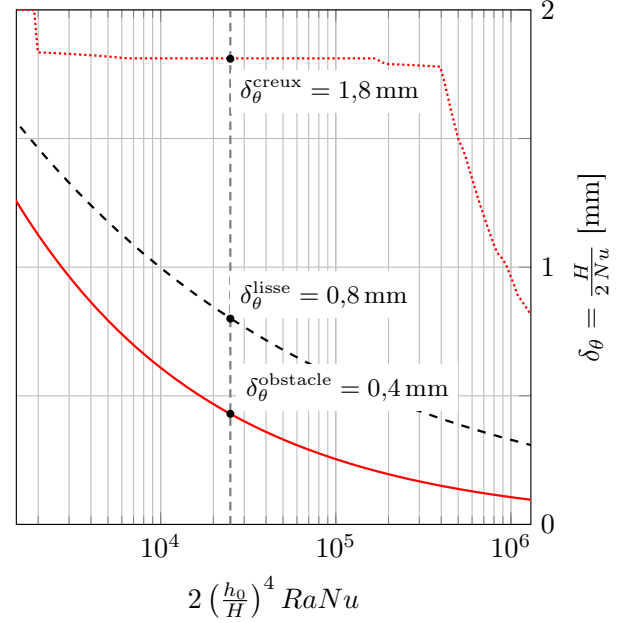
FIGURE 4.9 – Épaisseur de la couche limite thermique au-dessus de l'obstacle (trait plein rouge), dans le creux (pointillés rouge) et près de la plaque lisse (ligne pointillée noire). Ces épaisseurs sont tracées à partir de l'équation 4.12, de l'équation 4.18 et du modèle de Grossmann-Lohse, respectivement.
