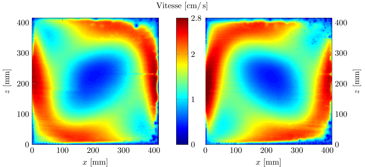
FIGURE 5.1 – Comparaison du champ moyen des modules de vitesse pour les deux sens de rotation de la circulation grande échelle. Cellule \mathcal{RL} , Ra = 7,0 \times 10^{10} .
