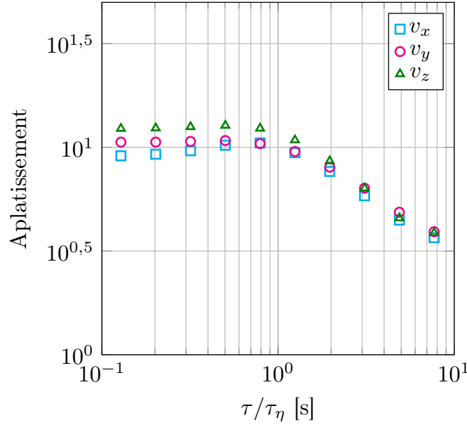
FIGURE 3.27 – Moment d'ordre quatre des distributions d'incrments de vitesse en fonction de l'incrment temporel associ.
