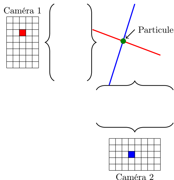
FIGURE 3.6 – Schéma de la correspondance tridimensionnelle d'une particule avec deux caméras. Le principe est extensible à un plus grand nombre de caméras.
