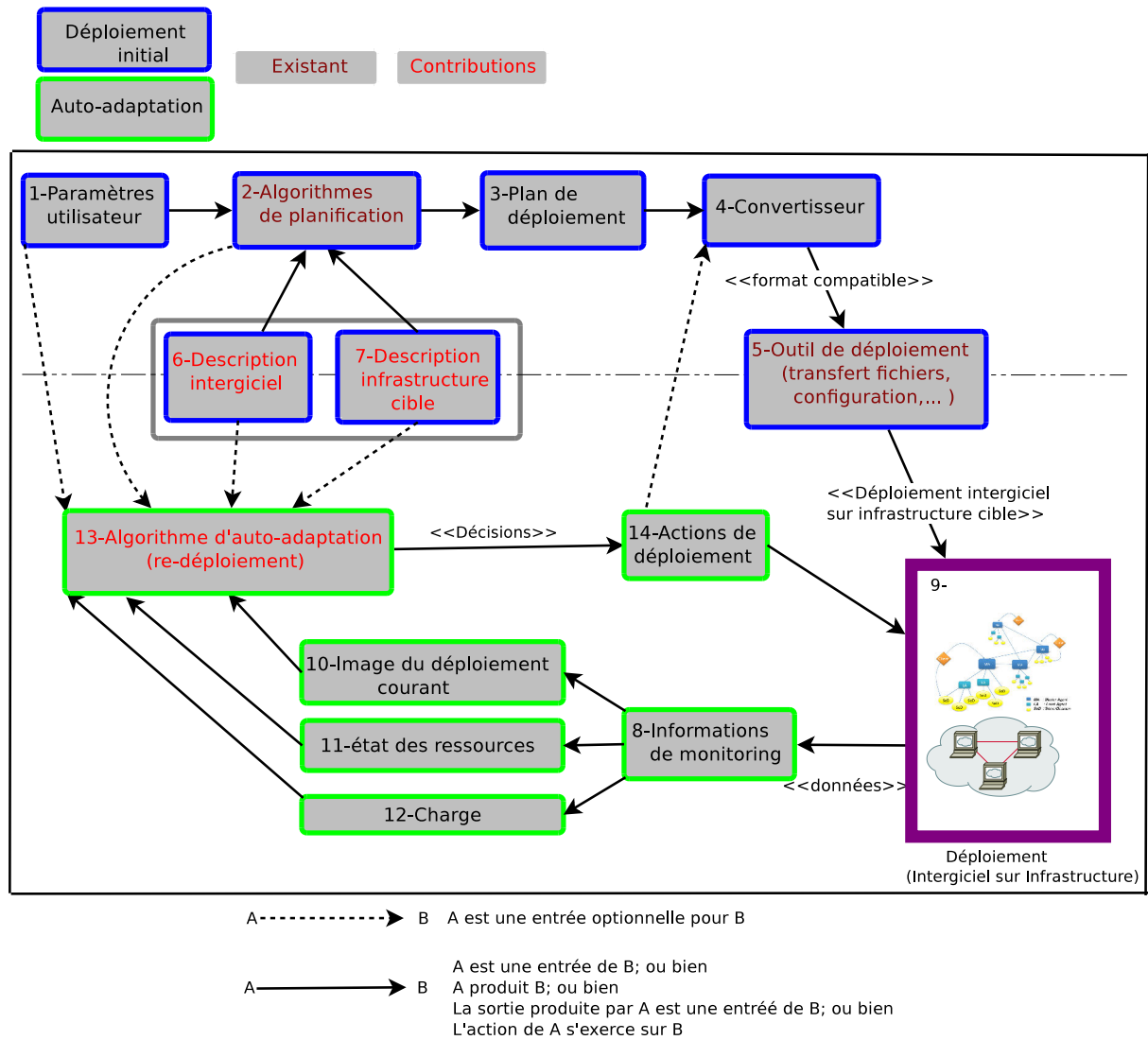
Figure 3.1: Architecture pour le déploiement auto-adaptatif d'intergiciel
