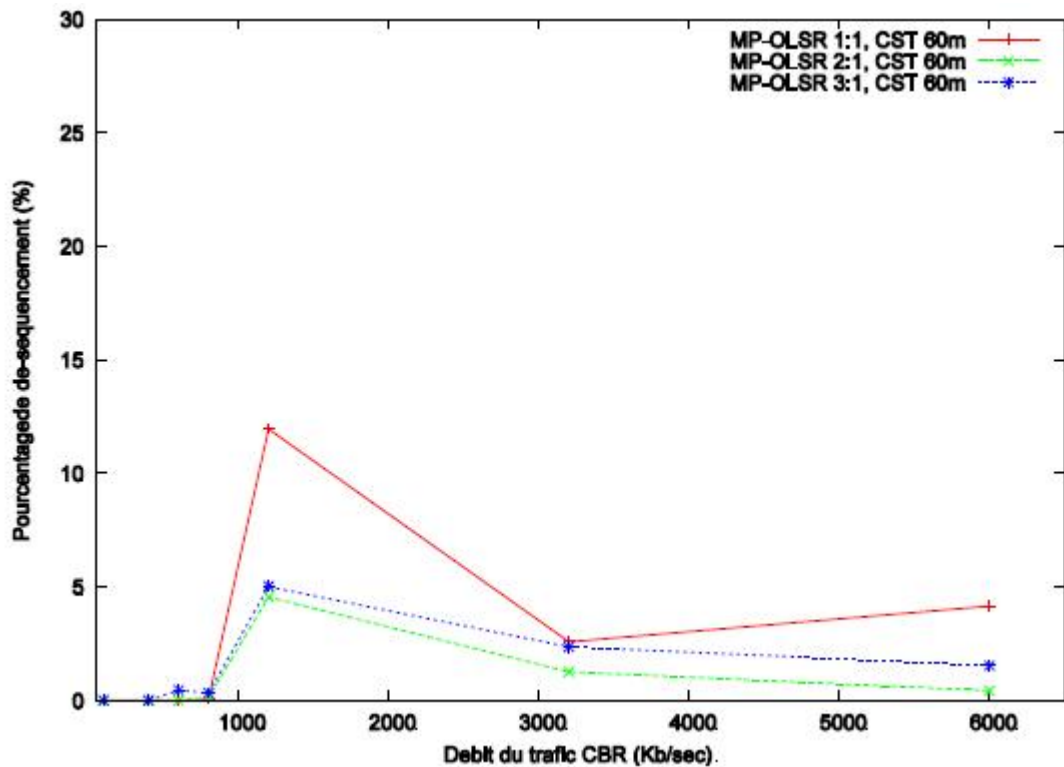
Figure 3.17 — Scénario 2 : taux de déséquence pour MP-OLSR avec les répartitions 1 :1, 2 :1 et 3 :1 en fonction du débit du flux CBR.
