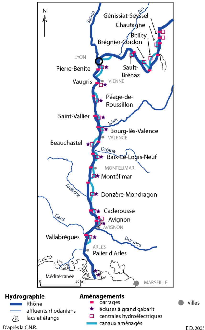
Figure 49. Carte des aménagements de la Compagnie Nationale du Rhône
