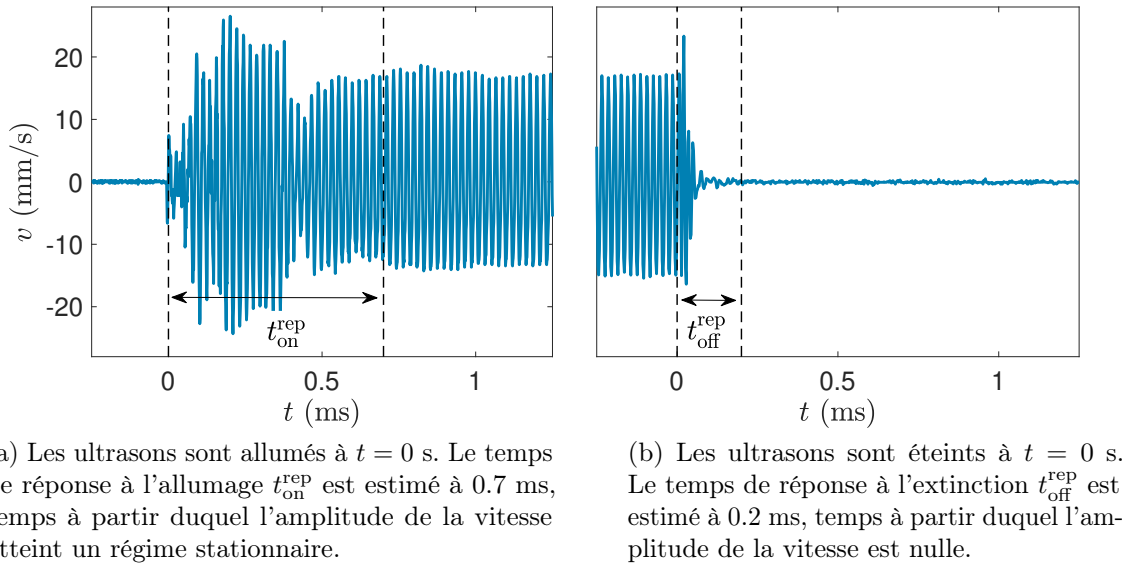
FIGURE 1.5 Réponse temporelle du transducteur piézoélectrique alimenté par un signal sinusoïdal de fréquence f_{\text{US}} = 45 kHz et d'amplitude 50 mV. La vitesse d'oscillation est mesurée au centre du transducteur piézoélectrique avec un vibromètre laser.
