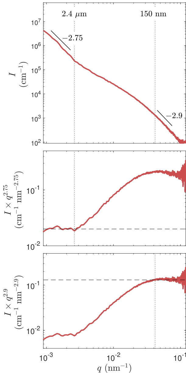
FIGURE 2.3 Analyse du spectre d'intensité d'un gel de noir de carbone (Cabot® Vulcan XC72R dans de l'huile minérale de viscosité \eta = 0.025 \text{ Pa.s} à 25^\circ\text{C} ) au repos et de concentration massique C = 6\% .
