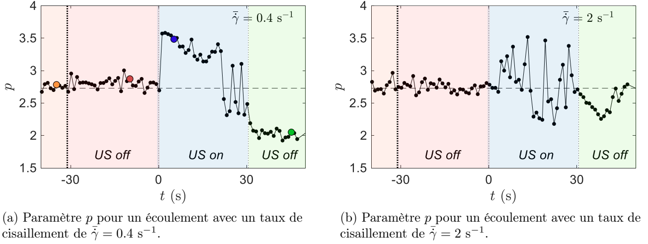
FIGURE 2.28 Évolution de l'exposant p en fonction du temps lorsque le gel de noir de carbone, en écoulement dans la cellule, est soumis à des ultrasons de pression acoustique P_{US} = 240 kPa. L'écoulement débute à t = -30 s, les ultrasons sont allumés à t = 0 s et éteints à t = 30 s.
