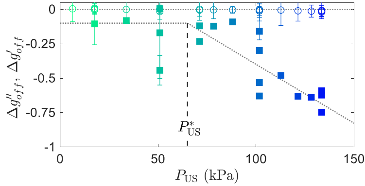
FIGURE 4.10 Variations relatives \Delta g'_{off} ( \square ) et \Delta g''_{off} ( \circ ) en fonction de la pression acoustique P_{US} . Les pointillés fins (...) servent de guides pour les yeux en mettant en évidence la tendance de \Delta g'_{off} et \Delta g''_{off} . À partir de la pression acoustique critique P_{US}^* , l'élasticité de la suspension est fortement diminuée par l'application d'ultrasons.
