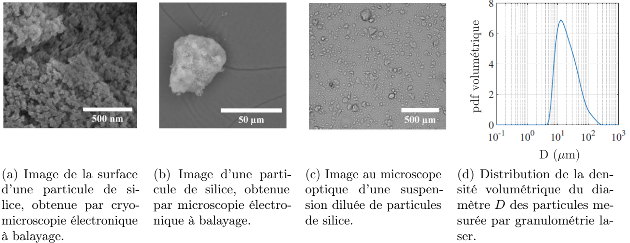
FIGURE 4.1 Caractérisation microscopique des particules de silice. Données issues d'une communication privée de C. Garat et G. Ovarlez.
