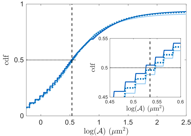
FIGURE 4.22 Influence du choix de l'intensité seuil sur la distribution cumulée normalisée pour une solution ayant été exposée à des ultrasons de puissance avec une pression acoustique P_{US} = 135 \text{ kPa} pendant 300 s. La cdf du logarithme des aires \log(\mathcal{A}) obtenue avec une intensité seuil minimale (●) diffère légèrement de celle obtenue avec l'intensité seuil maximale (●). Les pointillés représentent la cdf avec une intensité seuil choisie par l'oeil de l'expérimentateur de manière à optimiser la mesure des aires des particules.
