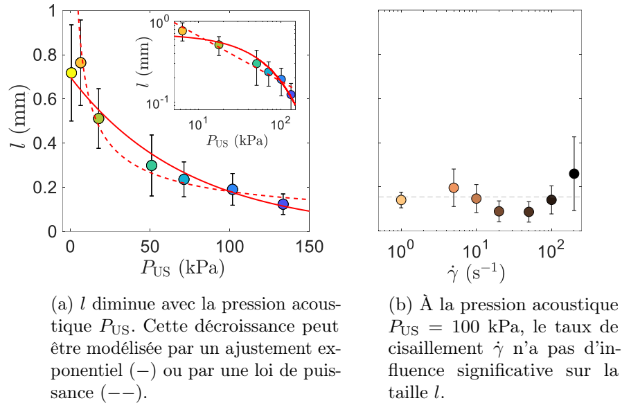
FIGURE 3.28 Évolution de la taille des domaines biréfringents l en fonction de la pression acoustique P_{US} et du taux de cisaillement \dot{\gamma} .
