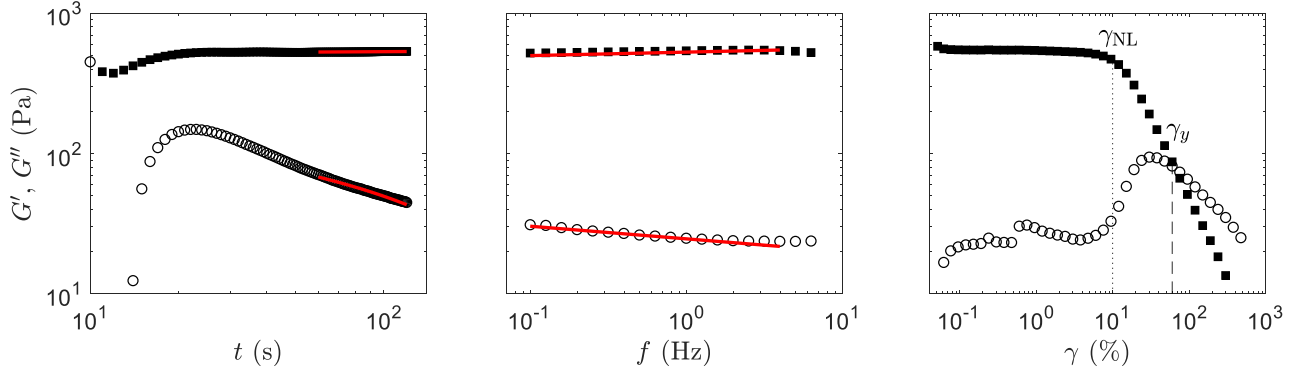
(a) Reprise des modules élastique G' (□) et visqueux G'' (○) après pré-cisaillement avec une déformation \gamma = 0.5 % et à la fréquence f = 1 Hz. Les courbes rouges représentent les ajustements du vieillissement logarithmique.
