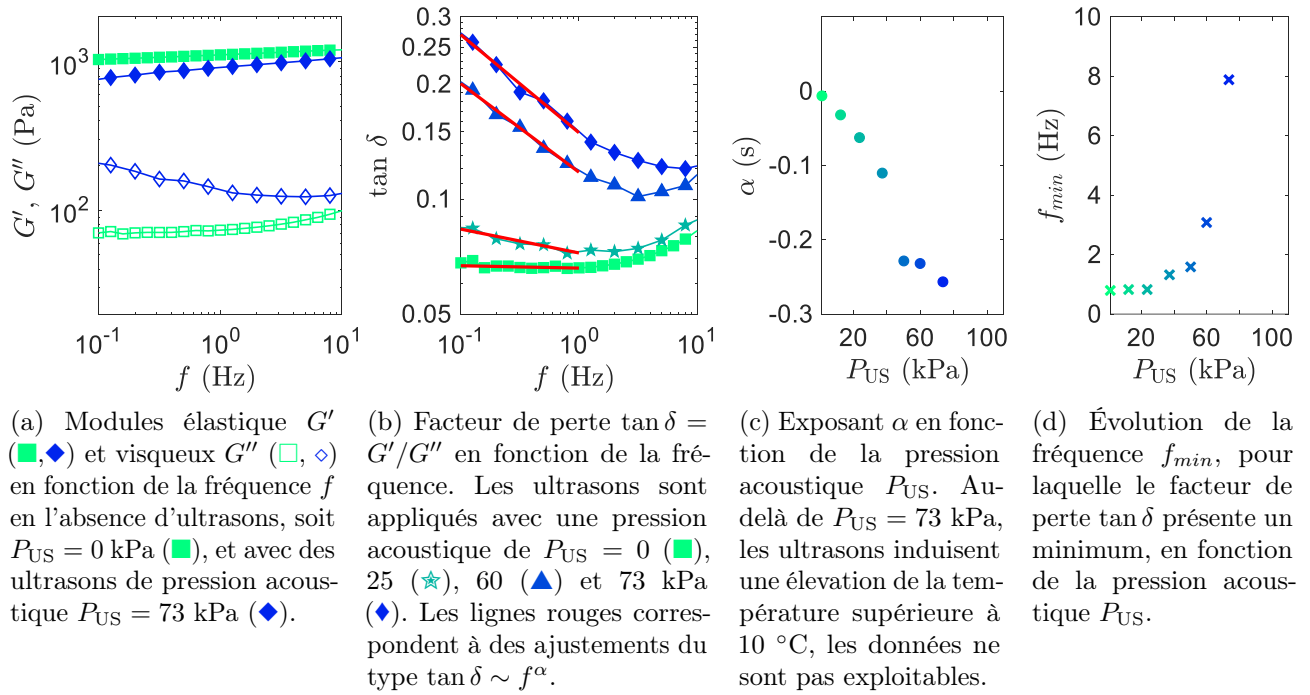
FIGURE 2.16 Influence des ultrasons de puissance sur le spectre viscoélastique du gel de noir de carbone (Cabot ® Vulcan XC72R) de concentration massique C = 6 %. Les mesures ont été réalisées à la déformation \gamma = 0.06 % avec deux cycles par point pour une durée totale du balayage en fréquence de 381 s avec une géométrie plane en plexiglas sablé de diamètre 50 mm.
