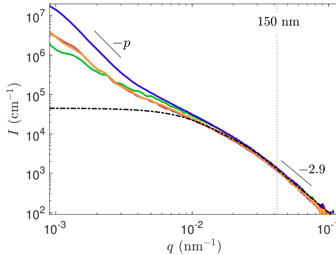
FIGURE 2.27 Spectres d'intensité I(q) pour le gel de noir de carbone au repos (orange), sous un écoulement \bar{\gamma} = 0.4 \text{ s}^{-1} (rouge), pendant l'application des ultrasons avec une pression acoustique P_{US} = 240 \text{ kPa} (bleu) et après les ultrasons (vert). Les pointillés noirs correspondent au facteur de forme des particules primaires de dimension fractale 2.9. Les instants correspondant à chacun des spectres sont indiqués par des symboles colorés sur la Figure 2.28(a).
