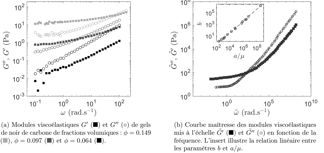
FIGURE 2.7 Comportement du spectre viscoélastique du gel de noir de carbone. Données extraites de [67].
