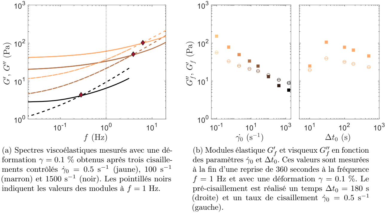
FIGURE 2.11 Influence du pré-cisaillement sur le spectre viscoélastique d'un gel de noir de carbone (Cabot® Vulcan PF dans de l'huile minérale de viscosité \eta = 252.1\text{ Pa.s} à 25^\circ\text{C} ). Ces données sont issues d'expériences menées avec une géométrie cône-plan.
