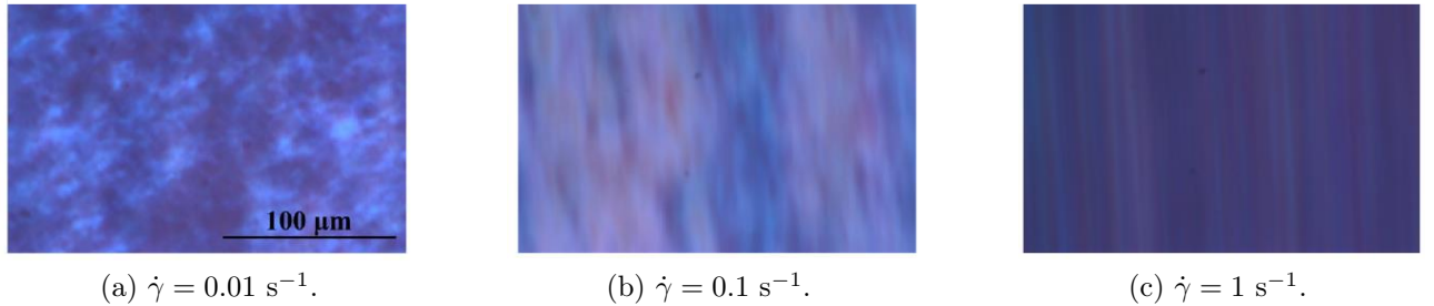
FIGURE 3.9 Effet du cisaillement d'un rhéomètre sur une suspension de nanocristaux de cellulose. Les images sont réalisées in situ entre polariseur et analyseur croisés. Les particules s'ordonnent en domaines alignés selon la direction de l'écoulement. Images extraites de [112].
