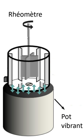
(a) Schéma du dispositif expérimental couplant la rhéologie à l'application de vibrations de basse fréquence [49].
