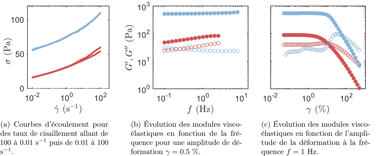
FIGURE 3.22 Viscoélasticité de la solution de nanocristaux de cellulose, fabriquée par l'Université du Maine à la concentration massique C = 12.2 %, avant (bleu) et après (rouge) une exposition aux ultrasons de puissance à la pression acoustique de 100 kPa pendant 180 s.
