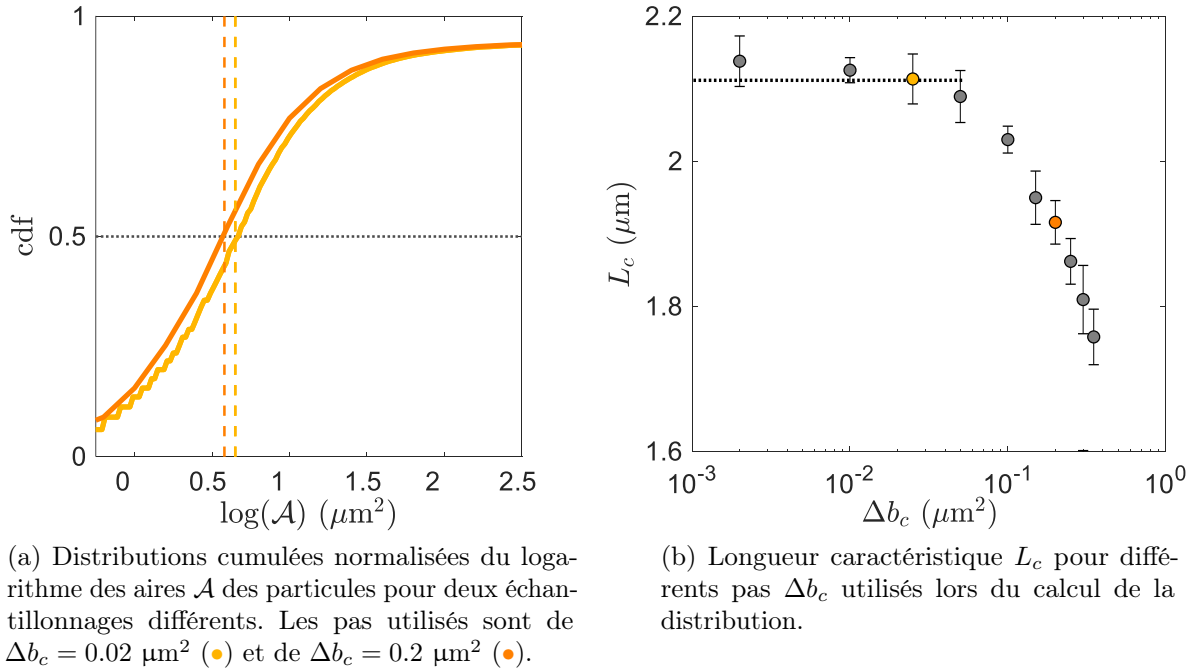
FIGURE 4.21 Définition de la longueur caractéristique L_c à partir de la distribution cumulée normalisée illustrée ici sur une solution ayant subi un cisaillement \dot{\gamma}_0 = 1 \text{ s}^{-1} pendant 300 s.
