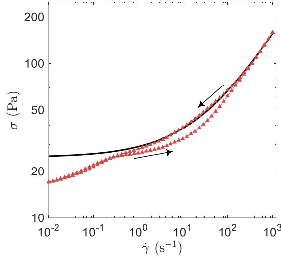
FIGURE 2.5 Courbe d'écoulement d'un gel de noir de carbone (Cabot® Vulcan XC72R dans de l'huile minérale de viscosité \eta = 0.025 Pa.s à 25^\circ\text{C} ) de concentration massique C = 6 %. La contrainte est mesurée pour des taux de cisaillement \dot{\gamma} décroissants puis croissants avec un temps d'attente par palier de 2 s. La courbe noire correspond à un ajustement de la contrainte par un modèle d'Herschel-Bulkley \sigma = \sigma_y + K\dot{\gamma}^n avec \sigma_y = 24.7 Pa, K = 4.24 SI et n = 0.50 .
