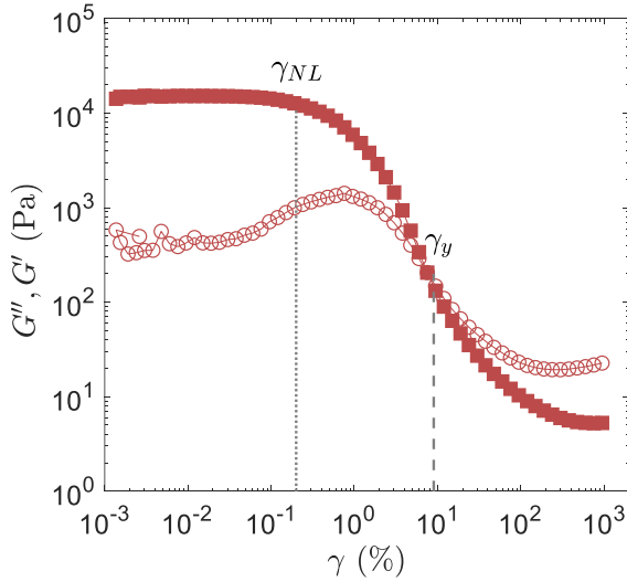
(a) Évolution des modules viscoélastiques G' et G'' en fonction de la déformation \gamma à une fréquence f = 1 Hz. Les pointillés mettent en évidence les déformations critiques \gamma_{NL} et \gamma_y .
