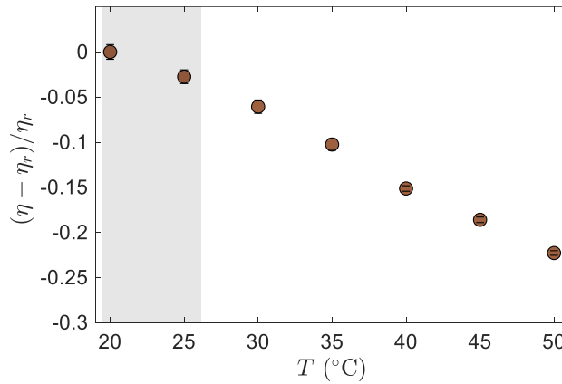
FIGURE 3.18 Évolution de la viscosité \eta avec la température T . Le rapport (\eta - \eta_r)/\eta_r permet d'évaluer la chute de viscosité suite à une augmentation de température, \eta_r étant la viscosité à 20 °C. La zone grisée correspond à la gamme de températures utilisées durant les expériences de ce manuscrit.
