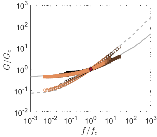
(a) Mise à l'échelle des spectres viscoélastiques à partir des paramètres G_c et f_c définis par G'(f_c) = G''(f_c) = G_c . Les données de V. Trappe et collaborateurs ont été ajoutées en traits gris [67].
