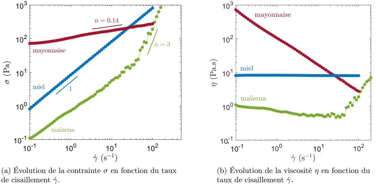
FIGURE 7 Écoulement du miel (Miel liquide d’acacia, Casino ® ) (•), de la mayonnaise (Amora ® ) (•) et d’une solution de maïzena (•) soumis à un taux de cisaillement \dot{\gamma} . L’obtention de ces mesures sera détaillée dans le chapitre 1.
