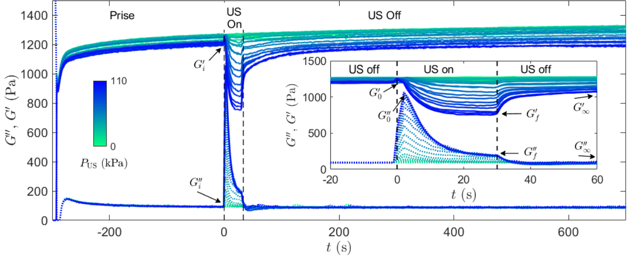
FIGURE 2.14 Effet des ultrasons de puissance sur les propriétés viscoélastiques d'un gel de noir de carbone (Cabot® Vulcan XC72R dans de l'huile minérale de viscosité \eta = 0.025 Pa.s à 25°C) de concentration massique C = 6 %. Après un pré-cisaillement s'arrêtant à t = -300 s, les modules élastique G' (—) et visqueux G'' (---) sont mesurés en fonction du temps dans le régime linéaire avec une amplitude de déformation \gamma = 0.06 % à la fréquence f = 1 Hz. Après 300 secondes, le gel possède des modules G'_i \simeq 1200 Pa et G''_i \simeq 100 Pa. Les ultrasons sont allumés à t = 0 s et éteints à t = 30 s avec une pression acoustique P_{US} allant de 0 kPa (vert) à 110 kPa (bleu). En insert, est représenté un zoom sur la période d'application des ultrasons. Les notations suivantes sont utilisées : G'_0 = G'(t = 1 s), G'_f = G'(t = 30 s), G'_\infty = G'(t = 700 s), G''_0 = G''(t = 3 s), G''_f = G''(t = 30 s) et G''_\infty = G''(t = 700 s). Ces mesures ont été effectuées dans une géométrie plane en plexiglas sablé de diamètre 50 mm.
