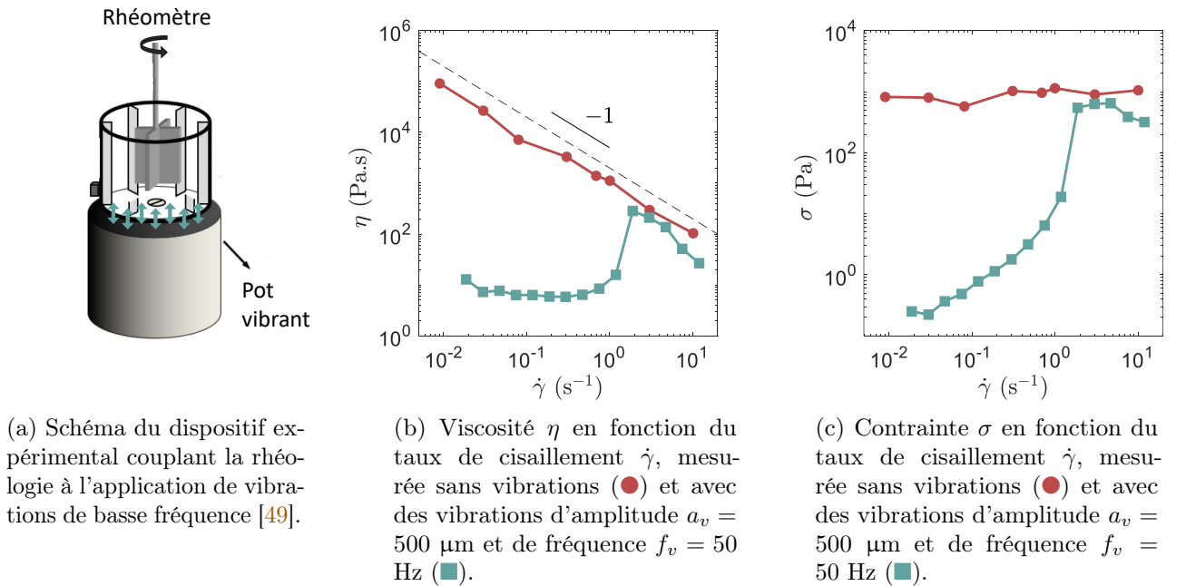
FIGURE 4.6 Effet des vibrations de basse fréquence sur l'écoulement de la suspension de silice de fraction massique \phi = 29 %.
