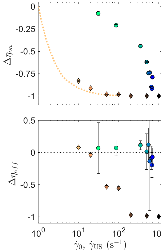
FIGURE 4.17 Comparaison de l'effet du changement de taux de cisaillement et de l'effet des ultrasons de puissance sur les variations de la viscosité de la suspension de silice.
