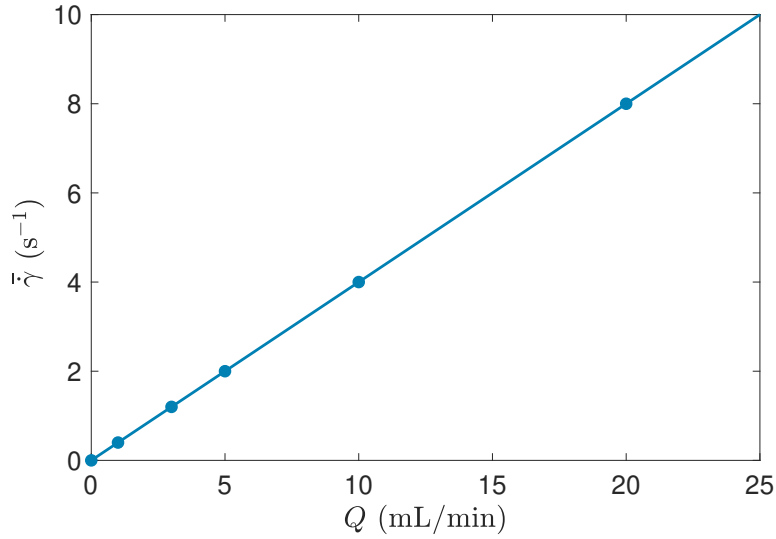
FIGURE 1.16 Taux de cisaillement \dot{\gamma} en fonction du débit imposé par le pousse seringue. (○) Débits imposés lors des expériences réalisées au cours de cette thèse.
