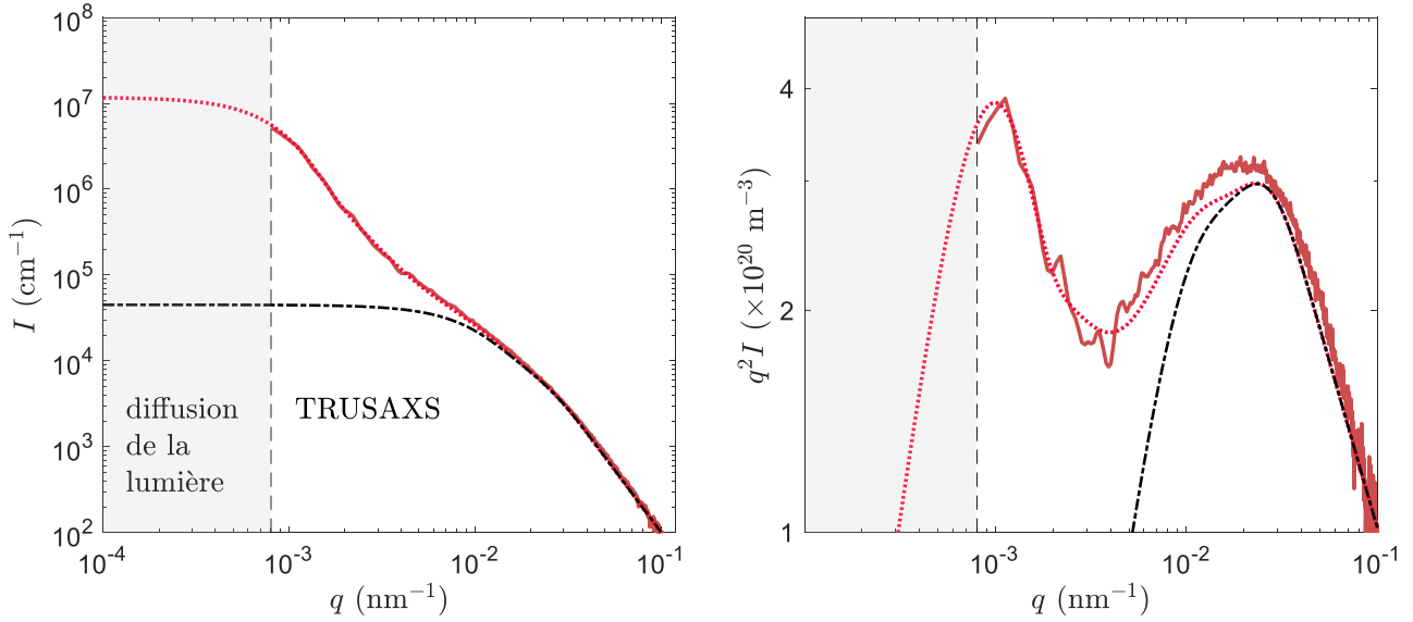
(a) Intensité diffusée par un gel noir de carbone au repos et son ajustement par un modèle de Beucage à deux niveaux ( \cdots ). Le facteur de forme des particules primaires, issue de cette modélisation, a été ajouté en pointillés noirs ( \cdot - \cdot ).
