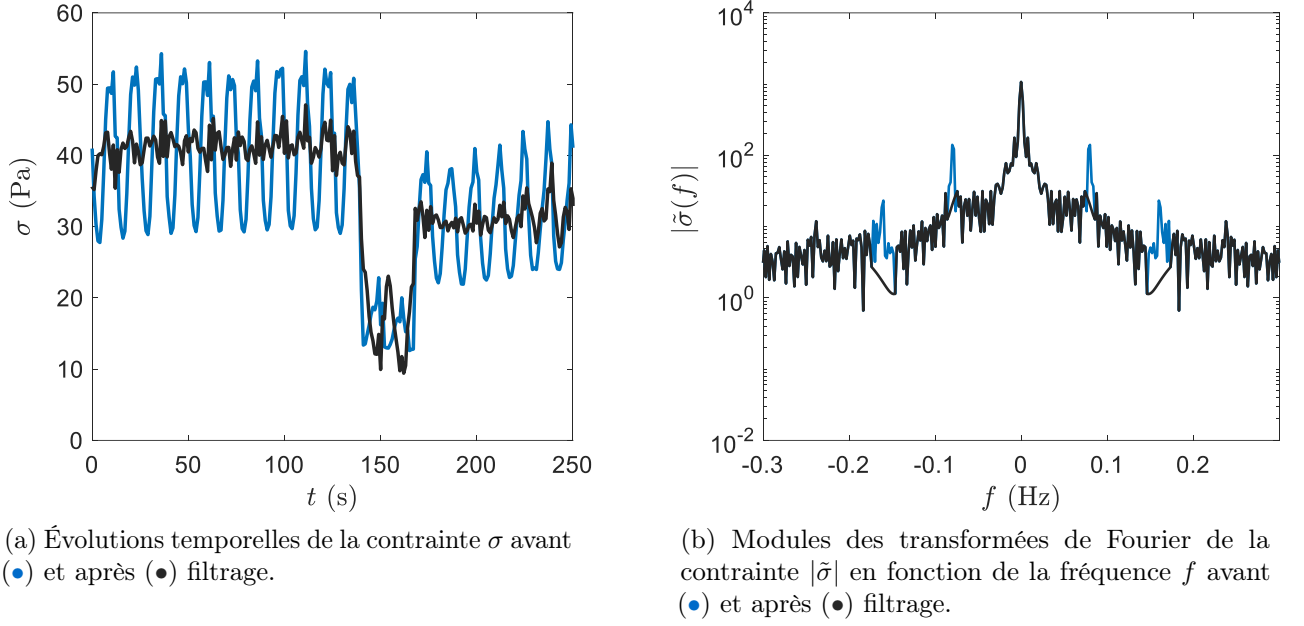
FIGURE 1.7 Exemple de filtrage d'un signal temporel de la contrainte mesurée avec un taux de cisaillement \dot{\gamma} = 10 \text{ s}^{-1} sur une suspension de silice de fraction massique \phi = 29 \% . La géométrie utilisée possède un rayon R = 20 \text{ mm} et un entrefer h = 1 \text{ mm} . La fréquence des oscillations est de f_a \sim 0.08 \text{ s}^{-1} .
