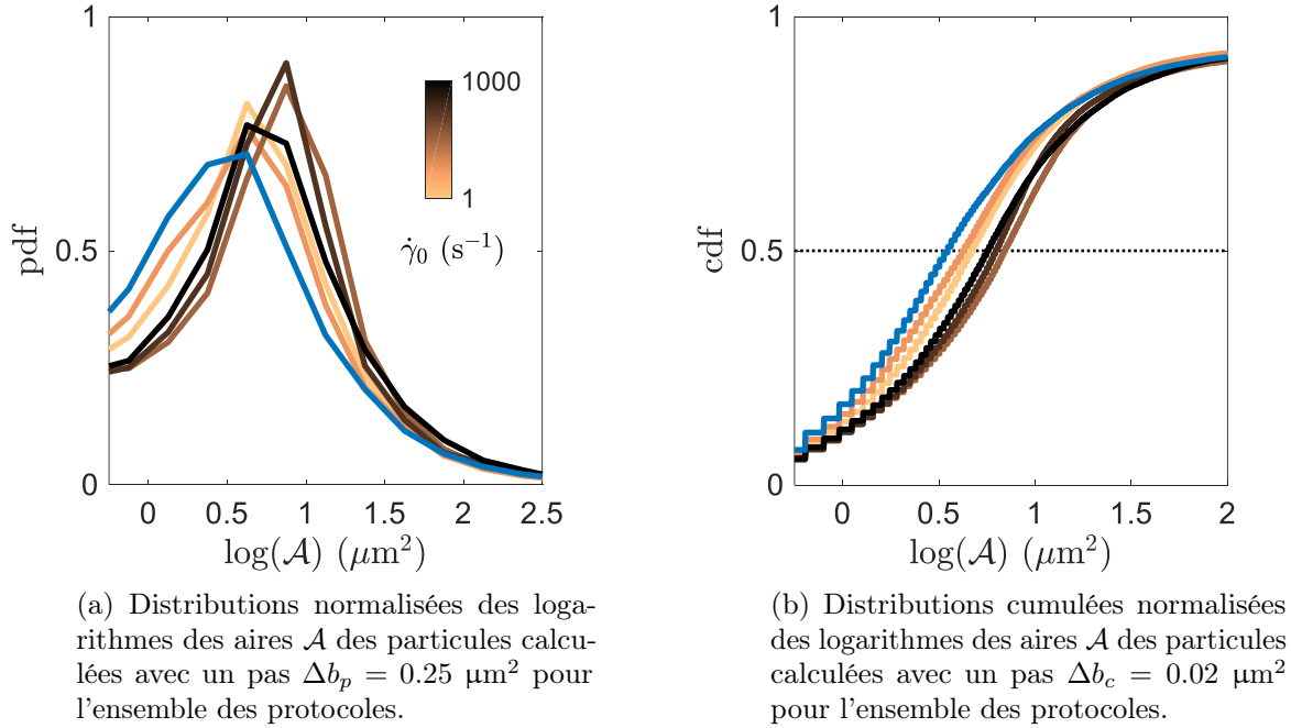
FIGURE 4.23 Influence du protocole sur les distributions normalisées du logarithme des aires \log(\mathcal{A}) des particules composant la suspension diluée de silice. La courbe bleue correspond à la solution cisailée avec un cisaillement \dot{\gamma}_m = 1 \text{ s}^{-1} et exposée à des ultrasons. Les autres courbes correspondent à des solutions uniquement cisillées : le dégradé de couleur du jaune au noir indique l'amplitude du cisaillement \dot{\gamma}_0 .
