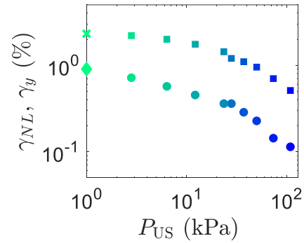
(b) Déformations caractéristiques \gamma_{NL} (●) et \gamma_y (■) en fonction de la pression acoustique P_{US} . La croix et le diamant représentent respectivement les déformations \gamma_{NL} et \gamma_y mesurées en l'absence d'ultrasons, soit P_{US} = 0 kPa.
