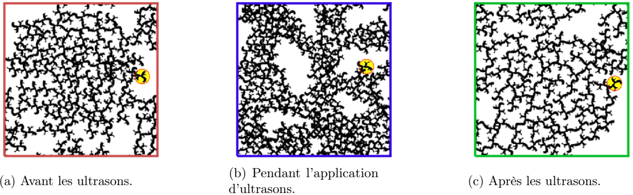
FIGURE 2.30 Mécanisme microscopique proposé pour expliquer les effets des ultrasons de puissance sur le gel de noir de carbone. Le disque jaune indique le rayon de giration d'un agrégat primaire de l'ordre de 150 nm.
