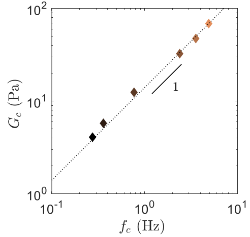
(b) Module de croisement G_c en fonction de la fréquence de croisement f_c . Les pointillés indiquent une loi de puissance du type G_c \propto f_c .
