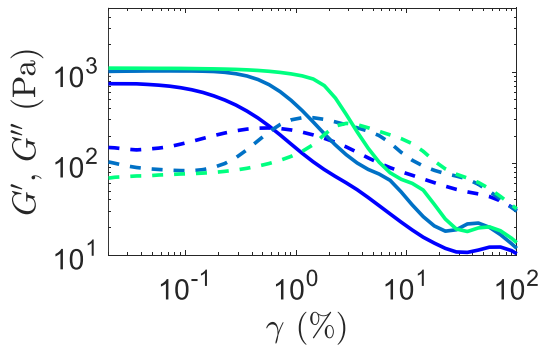
(a) Modules élastique G' (—) et visqueux G'' (---) en fonction de la déformation \gamma pour différentes pressions acoustiques : P_{US} = 0 (vert), 30 (turquoise) et 110 kPa (bleu).
