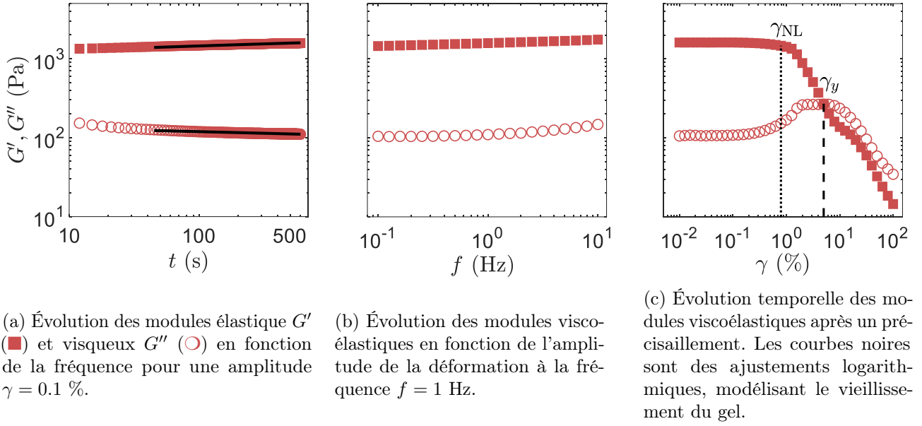
FIGURE 2.6 Propriétés viscoélastiques d'un gel de noir de carbone (Cabot® Vulcan XC72R dans de l'huile minérale de viscosité \eta = 0.025 Pa.s à 25^\circ\text{C} ) de concentration massique C = 6 %.
