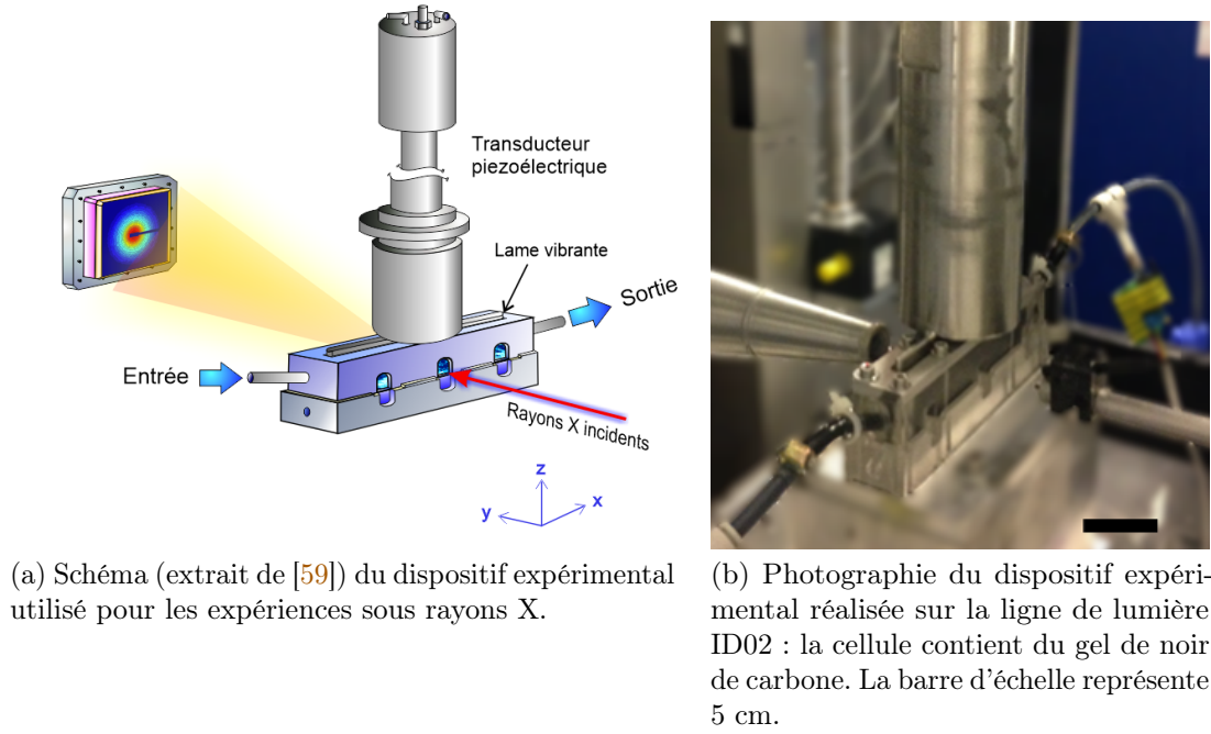
FIGURE 1.14 Système expérimental couplant la diffusion des rayons X avec l'application d'ultrasons de puissance.
