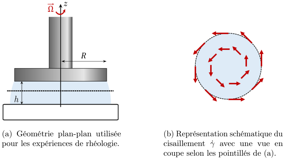
FIGURE 1.1 Rhéomètre en géométrie plan-plan.
