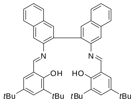
Figure 3.7 : Structure de la base de Schiff utilisée pour la synthèse de carbonates cycliques
