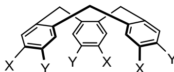
Figure 1.60 : Structure générique d'une unité cyclotrivratriylène (CTV)
