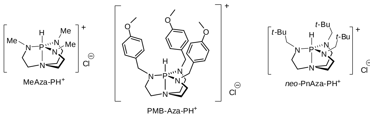
Figure 3.10 : Structures des trois catalyseurs utilisés pour l'étude de la réaction entre l'oxyde de styrène et le \text{CO}_2
