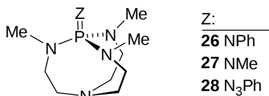
Figure 1.37 : Structure des iminophosphoranes et azidophosphoraneobtenus à partir des proazaphosphatranes
