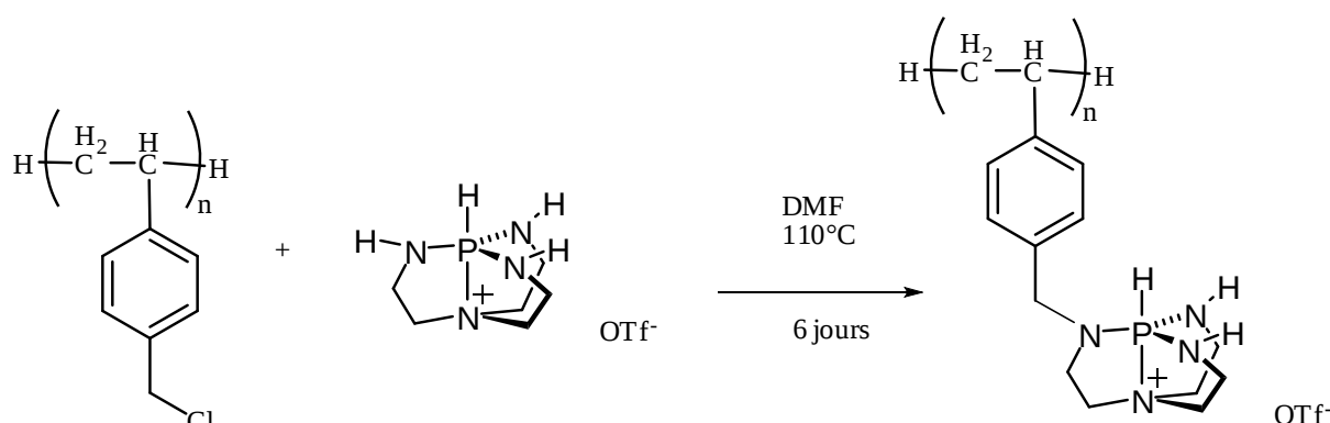
Figure 1.55 : Greffage d'un azaphosphatane sur résine de Merrifield
