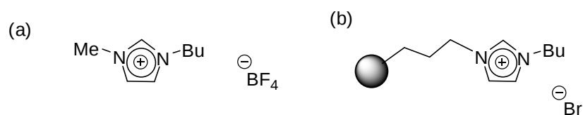
Figure 3.6 : Structures: (a) du sel de tétrafluoroborate et (b) du sel de bromure supporté sur silice
