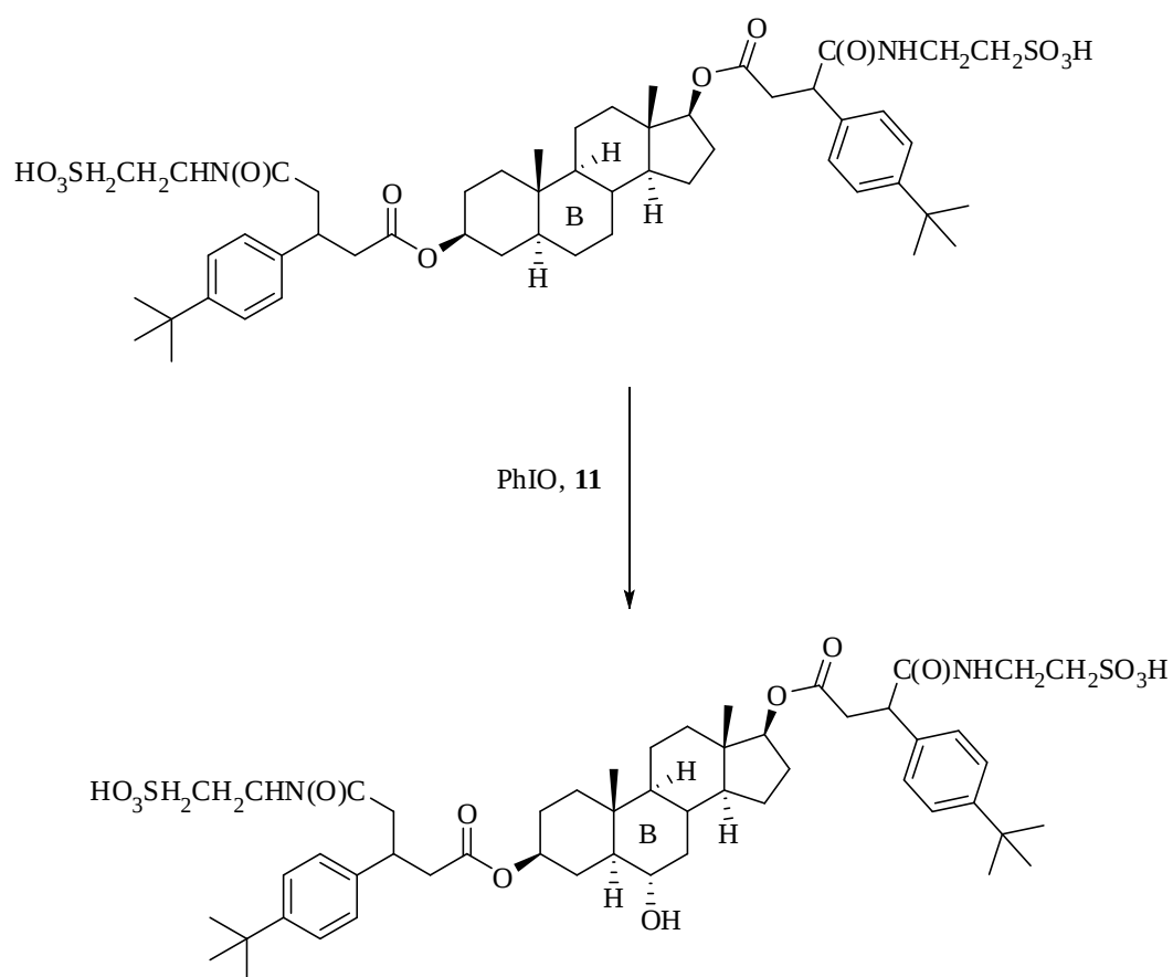
Figure 1.25 : : Structure du complexe manganèse-porphyrine comprenant quatre β-cyclodextrines et réaction sélective d'hydroxylation d'un dérivé de stéroïde
