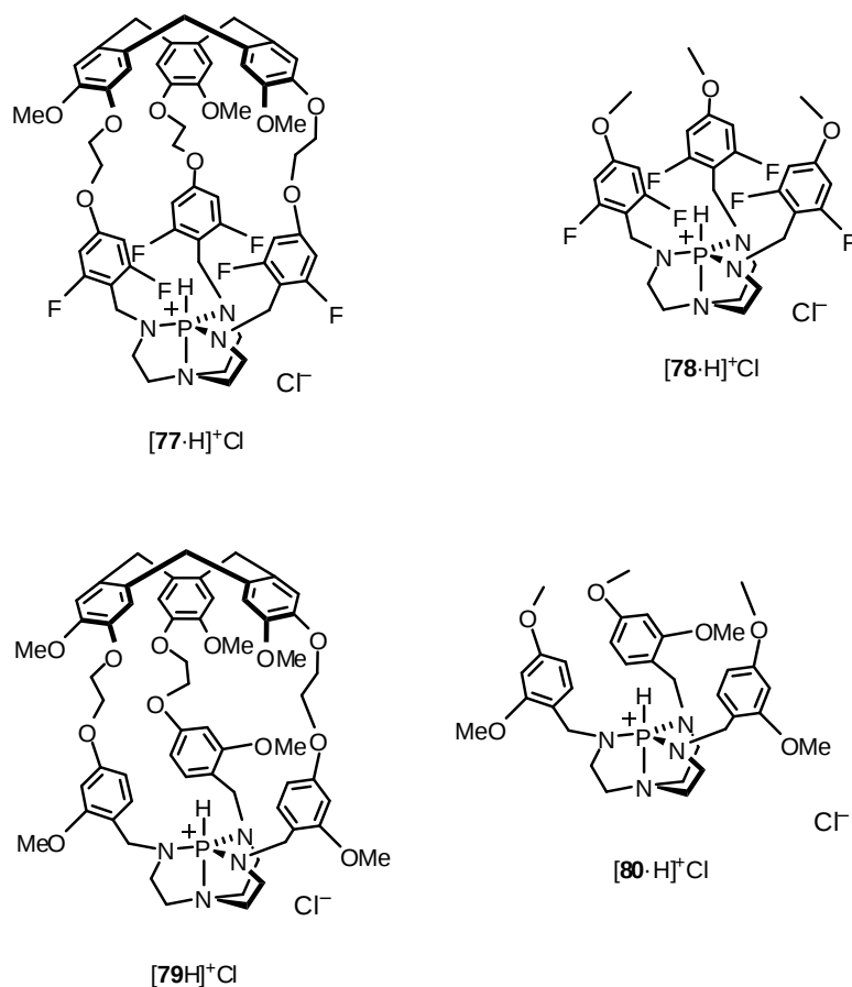
Figure 2.24 : Structures des azaphosphatranes supramoléculaires [77\cdot H]^+Cl^- et [78\cdot H]^+Cl^- et de leurs modèles [79\cdot H]^+Cl^- et [80\cdot H]^+Cl^-
