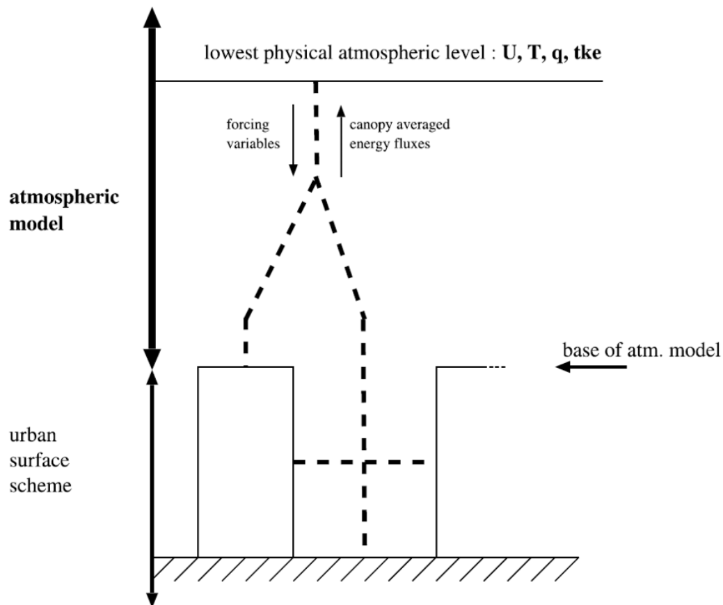
Figure 4 : Vue schématique de la configuration à couche unique du modèle TEB. Les lignes en pointillé représentent l'interaction des surfaces avec le modèle atmosphérique (Source : Masson, 2006).
