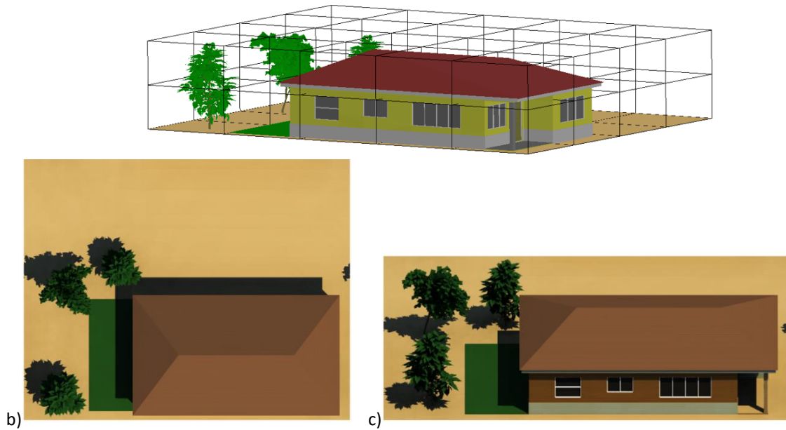
Figure 3.11 : Images DART de paysage schématique. a) Scène 3D DART, à la résolution spatiale 10mx10mx5m, comprenant 3 arbres et 1 bâtiment, simulés avec des surfaces triangulaires. b) Composition colorée DART au nadir. c) Composition colorée DART pour un angle zénithal de visée de 60°.
