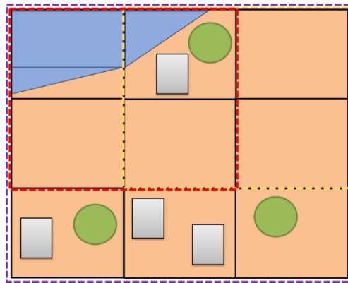
Figure 3.15 : Schéma présentant deux grilles d'analyse de mailles de 2x2 pixels et une grille de maille de 3x3 pixels. Les éléments présents sont le sol (beige), la végétation (vert), le toit (gris), et l'eau (bleu). Le premier groupe de pixel considéré est encadré en pointillés jaune, le deuxième en pointillés rouge, et le troisième en pointillés violets.
