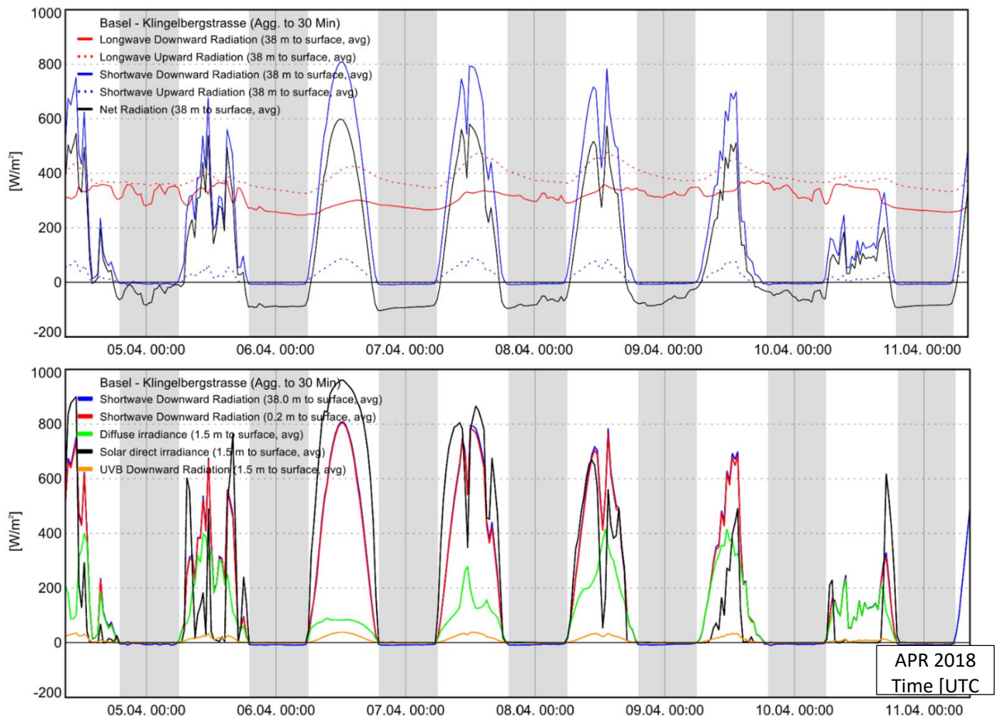
Figure 3.7 : Eclairage dans les grandes et courtes longueurs d'onde mesuré par une tour de flux à 38m au-dessus de la surface au centre de Bâle (Klingelbergstrasse). Haut : bilan radiatif ainsi qu' éclairage et exitance dans les courtes et grandes longueurs d'onde [ \text{W/m}^2 ]. Bas : éclairements solaires directs et diffus dans les courtes longueurs d'onde, à différentes altitudes [ \text{W/m}^2 ]. Les données sont agrégées à des intervalles de temps de 30 minutes, pour la semaine du 5 Avril au 11 Avril 2018. (Source : Université de Bâle - https://mcr.unibas.ch/dolueq2/ )
