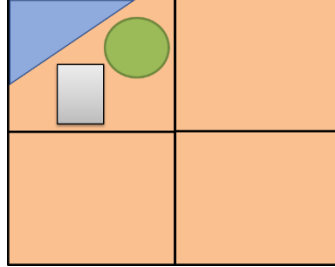
Figure 3.13 : Représentation de schématique de système insoluble pour l'algorithme d'inversion. Comme dans la Figure 3.12, quatre éléments sont présents : sol (beige), végétation (vert), toit (gris), et rivière (bleu).
