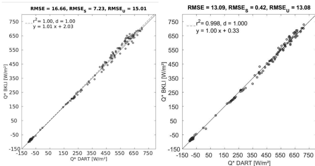
Figure 4.25 : Corrélogrammes de comparaison des valeurs de Q^* simulées et mesurées par la tour BKL de la ville de Bâle, pour la série MODIS-A (à gauche) et MODIS-T (à droite).
