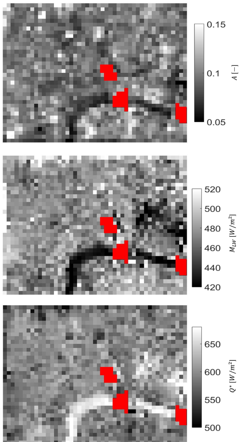
Figure 4.21 : Cartes d'albédo (haut), d'existance thermique (milieu), et de bilan radiatif (bas) de Londres, dérivées d'une image Landsat-8 du 08.07.2016 à 11h00, à 100m de résolution. Masques de nuages en rouge.
