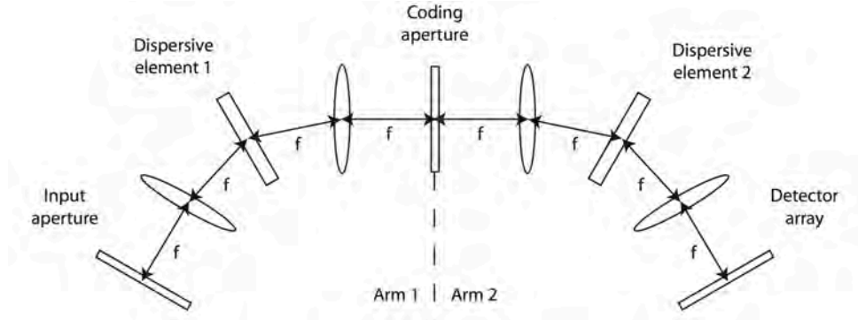
FIGURE 1.9 – Schéma du principe optique du concept Dual-Disperser CASSI (extrait de [GJB + 07])
