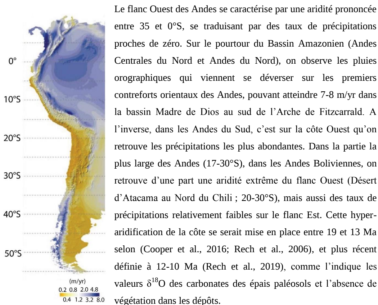
Figure I-13 : Précipitations moyennes annuelles (Montgomery et al., 2001)
