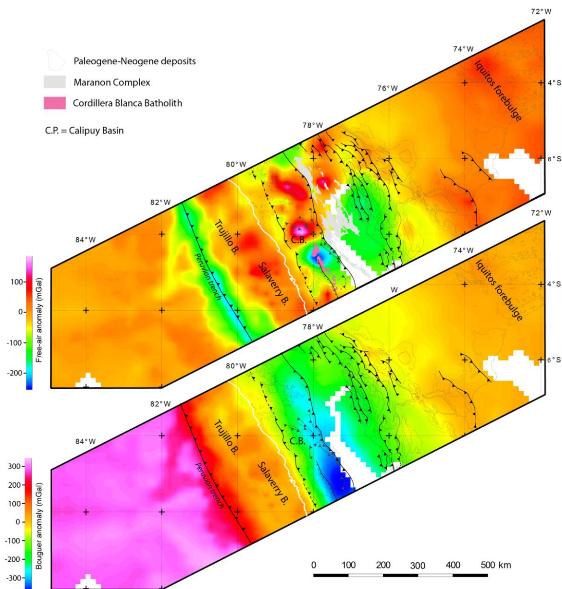
Figure III-6 : Cartes des anomalies à l'air libre (haut) et de Bouguer complète (bas), où sont localisées les failles principales, le batholite de la Cordillère Blanche, le complexe du Maraón et les contours des dépôts volcano-sédimentaires Néogène et Paléogène.
