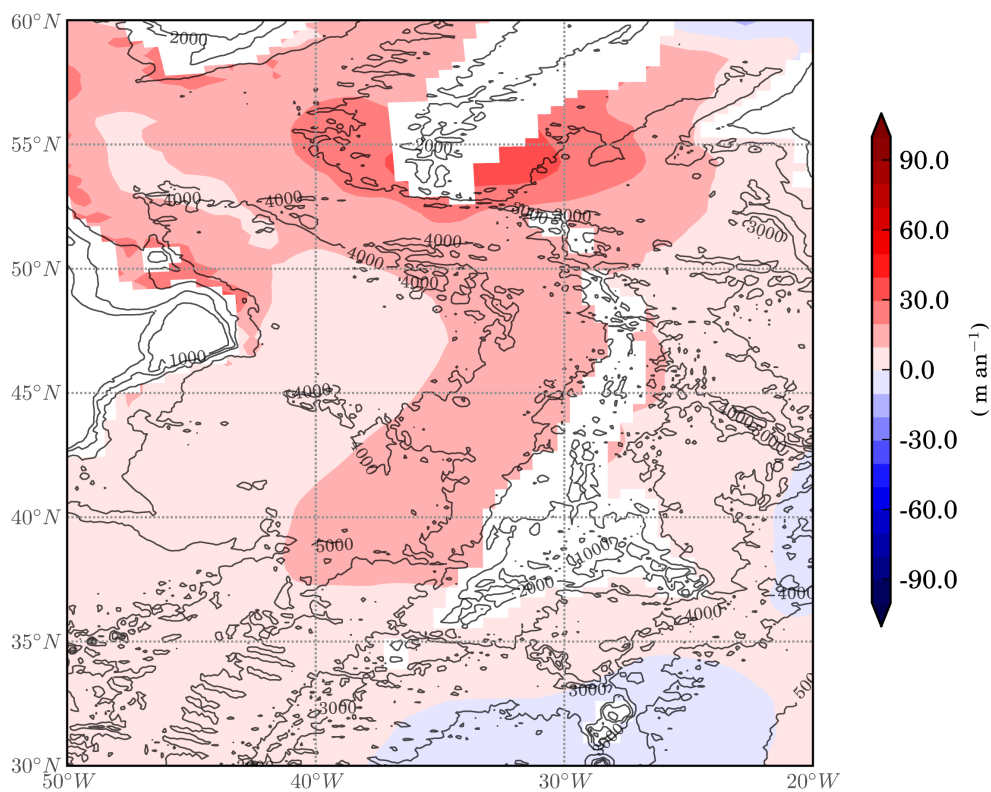
FIGURE 3.3 – Carte du taux de changement de la profondeur de l'isopycne 36.925 kg m -3 ( \partial z / \partial t ) entre 1990 et 2009 dans ORCA_REF.
