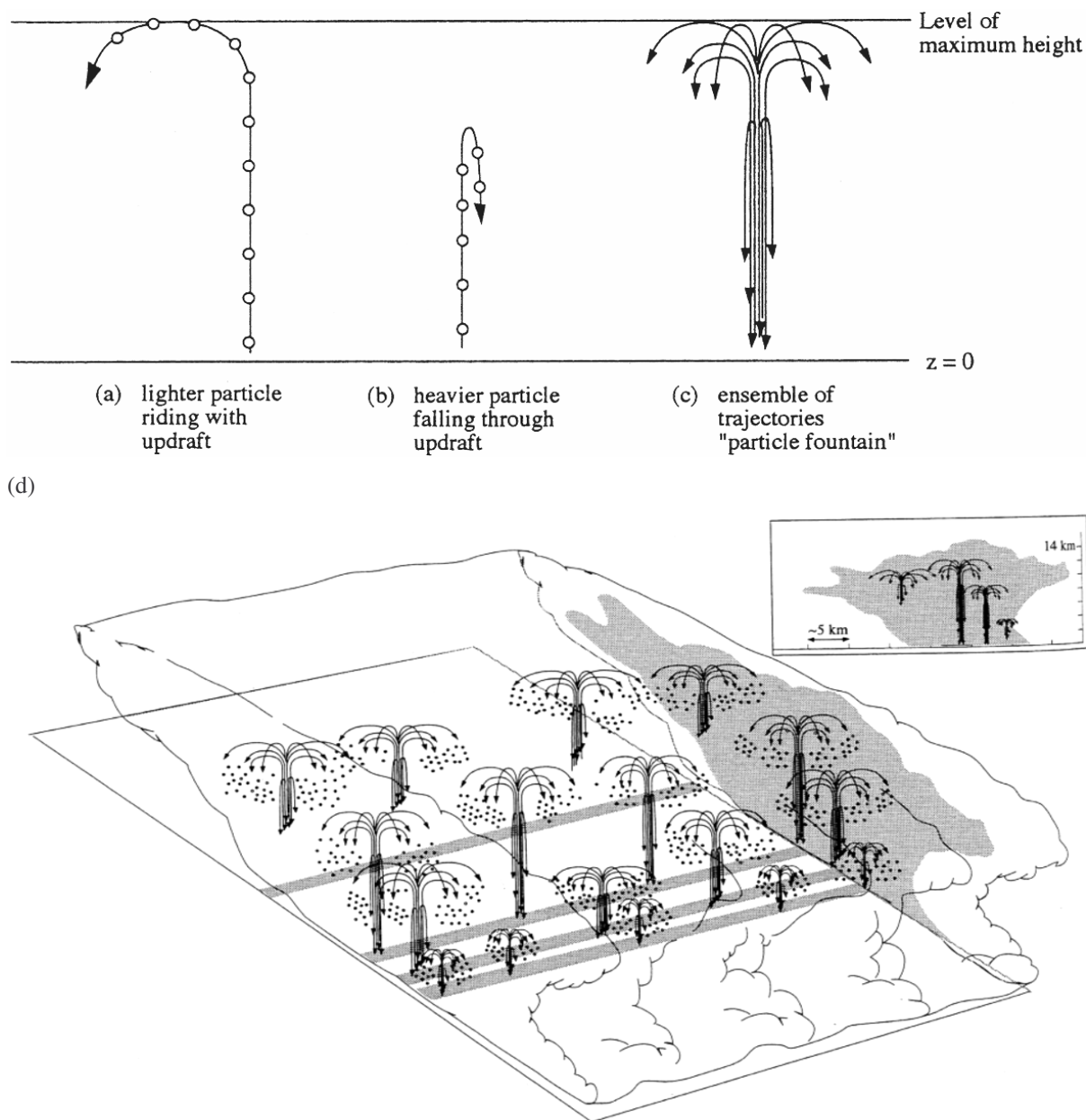
Fig. 10- Modèle de la fontaine de particules. (a) Trajectoire des particules les plus légères (cristaux de glace). (b) Trajectoire des particules les plus lourdes. (c) Une fontaine de particule. (d) Système multicellulaire composé d'un ensemble de fontaines de particules. D'après Yuter and Houze (1995).
