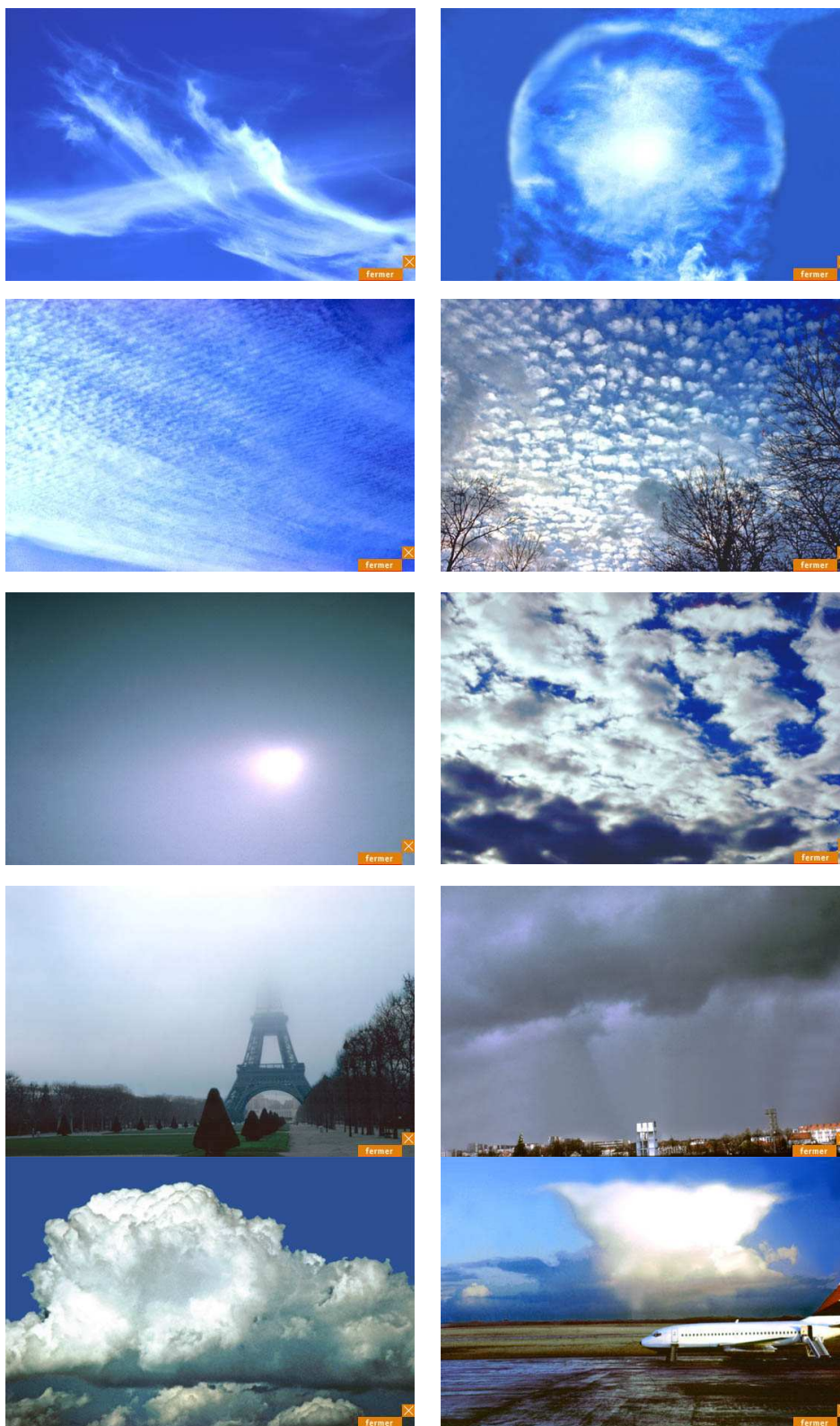
Photos des genres de nuages considérés par l'OMM. De gauche à droite et de haut en bas : Cirrus, Cirrostratus, Cirrocumulus, Altopumulus, Altostratus, Stratocumulus, Stratus, Nimbostratus, Cumulus et Cumulonimbus. D'après Météo-France ( http://www.meteo.fr ).
