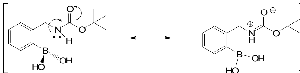
Figure 26: Délocalisation des électrons par résonance causée par l'ajout d'un groupement Boc.
