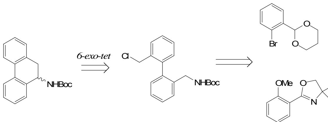
Figure 19 : Rétrosynthèse envisagée par Barberis pour la synthèse d'un composé modèle analogue à l'alcolchicine.
