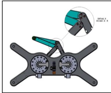
Figure 29 Contact entre les liens proximaux
