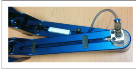
Figure 34 Passage du tuyau d'air
