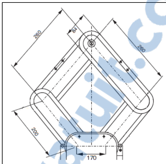
Figure 70 Dimensions du robot RP-5AH du Mitsubishi Electric Tirée de Mitsubishi (2012, http://www.mitsubishi-automation.fr/ )
