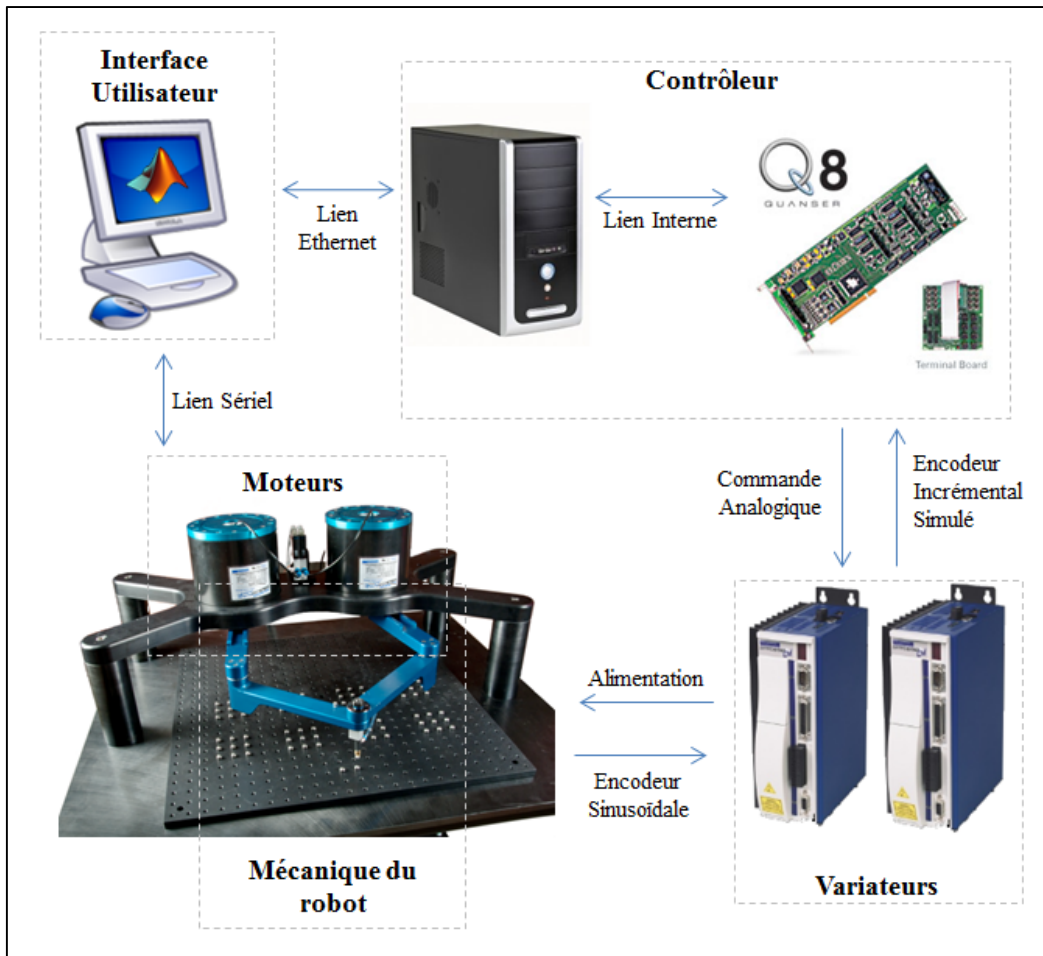
Figure 38 Composition du système
