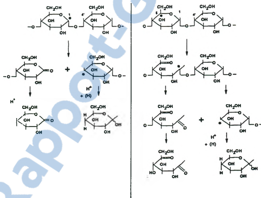
Figure III.11 b. Formation des radicaux libres des amidons irradiés par gamma (Sokhey et Hanna, 1993)
