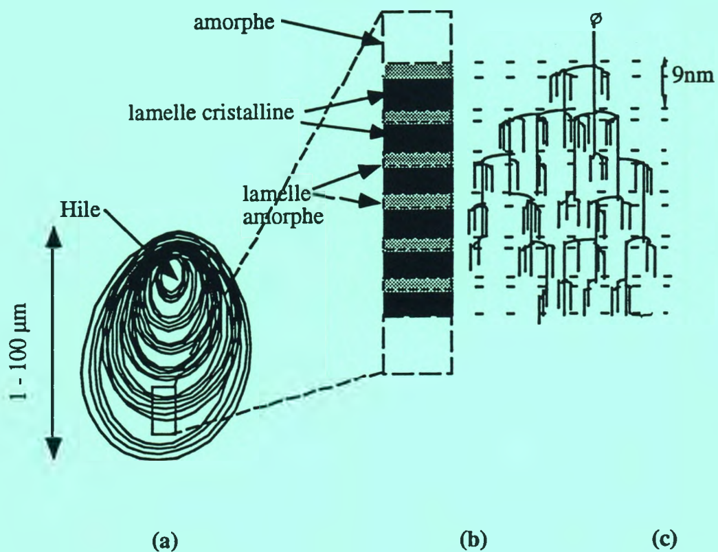
Figure I.1. Différents niveaux d'organisation dans un grain d'amidon.
