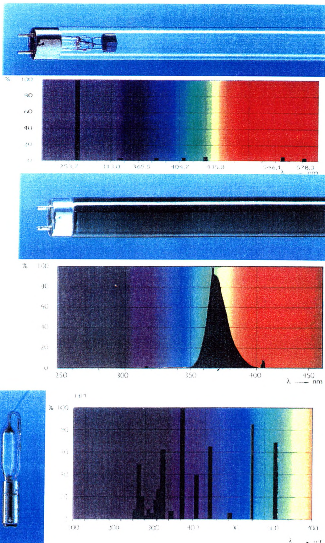
Annexe 2. Lampes utilisées pour l'irradiation de l'amidon avec leurs spectres respectifs d'émission (haut : \lambda_{max} 254 nm ; centre : \lambda_{max} 360 nm ; bas : \lambda ~200-600 nm).
