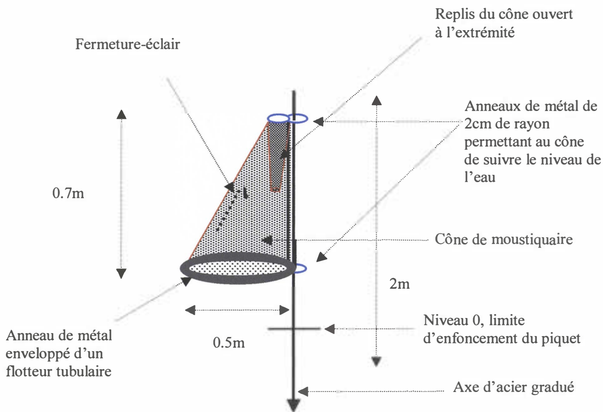
Fig 15) Piège à émergence utilisé dans l'étude de la fièvre de la vallée du Rift, Dakar, juin 2001
