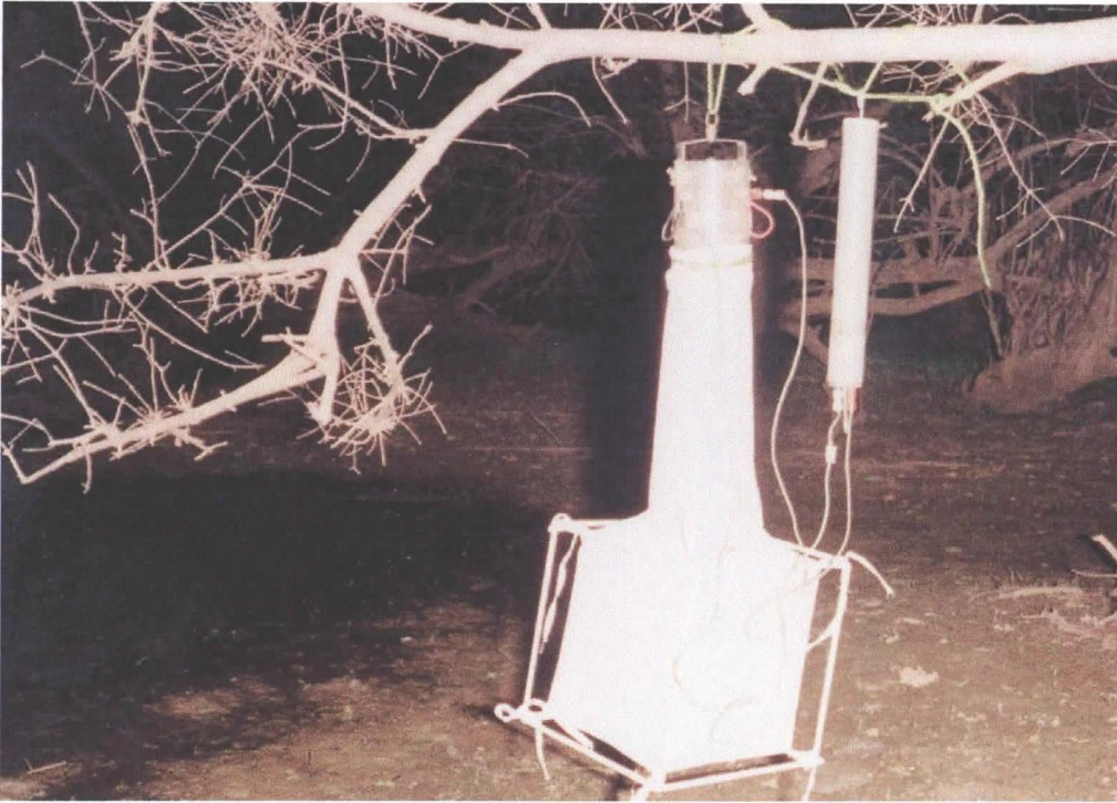
Fig 17) Pose d'un piège CDC au bord de la mare de Furdu
