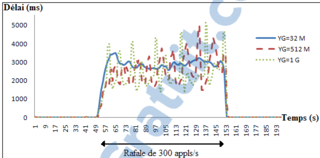
Figure 5.3 L'effet de l'YG sur les délais
