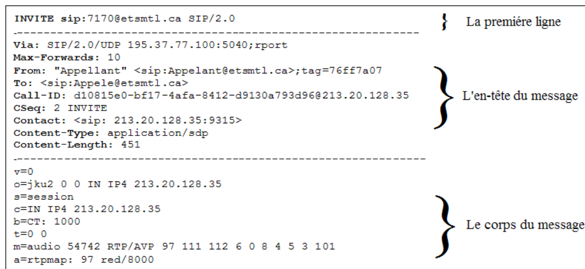
Figure 1.1 Le message 'Invite'
