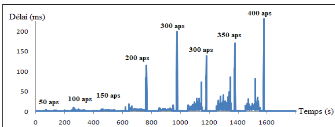
Figure 5.19 Le délai '200-Ack'
