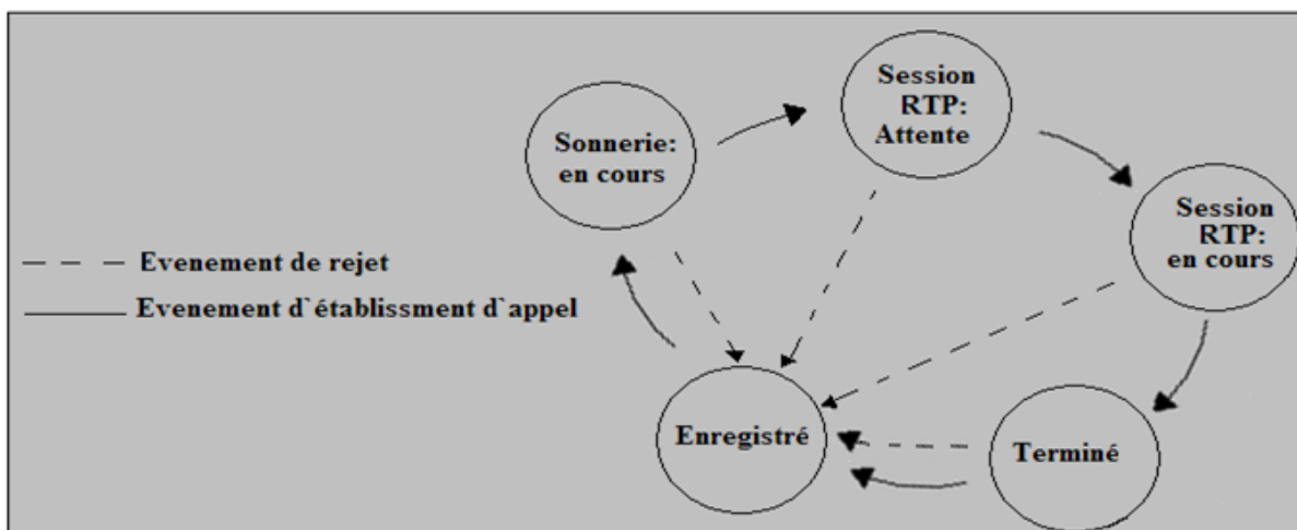
Figure 3.7 Le modèle UAS de Markov
