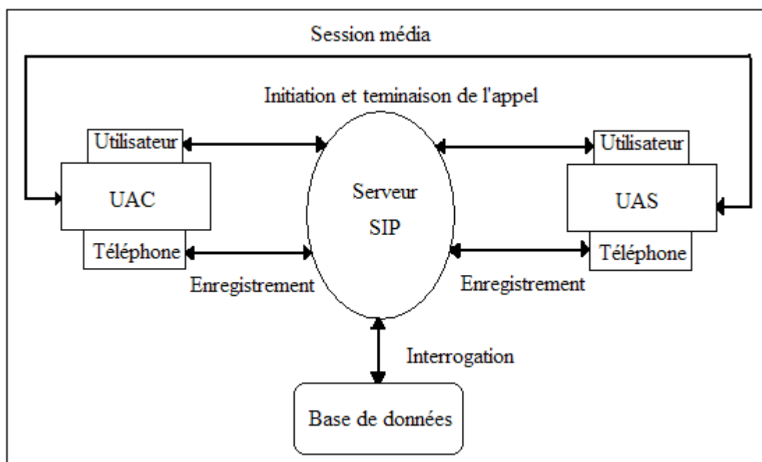
Figure 3.3 Un système standard d'évaluation SIP
