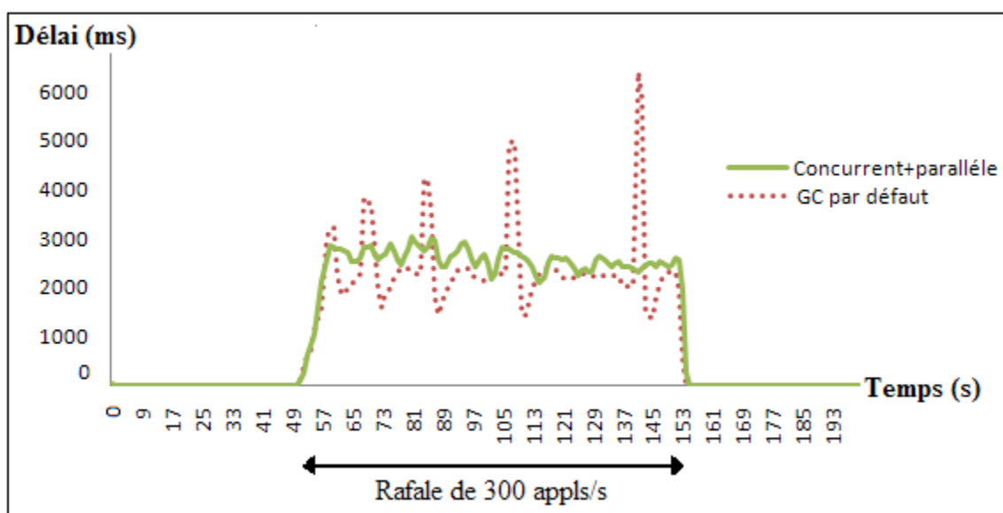
Figure 5.2 L'effet des algorithmes du GC sur le délai
