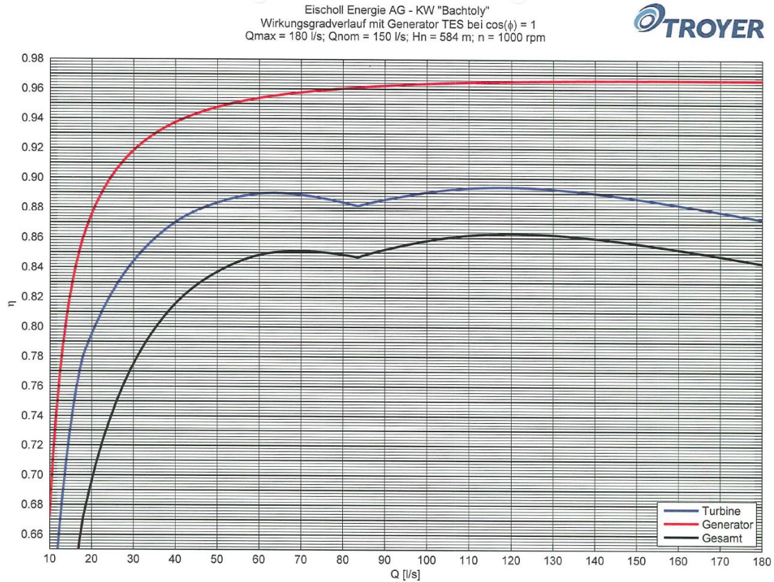
Graphique 6 Rendements de la turbine et du générateur en fonction du débit
