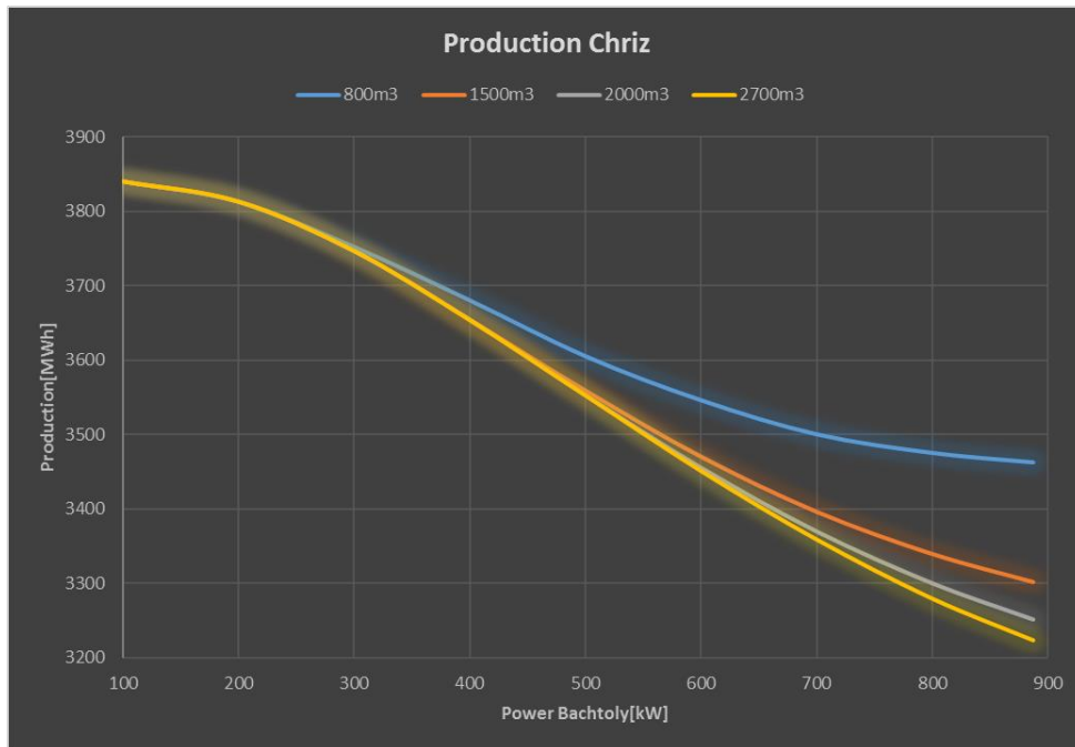
Graphique 17 Production de Chriz en fonction de la puissance de Bachtoly
