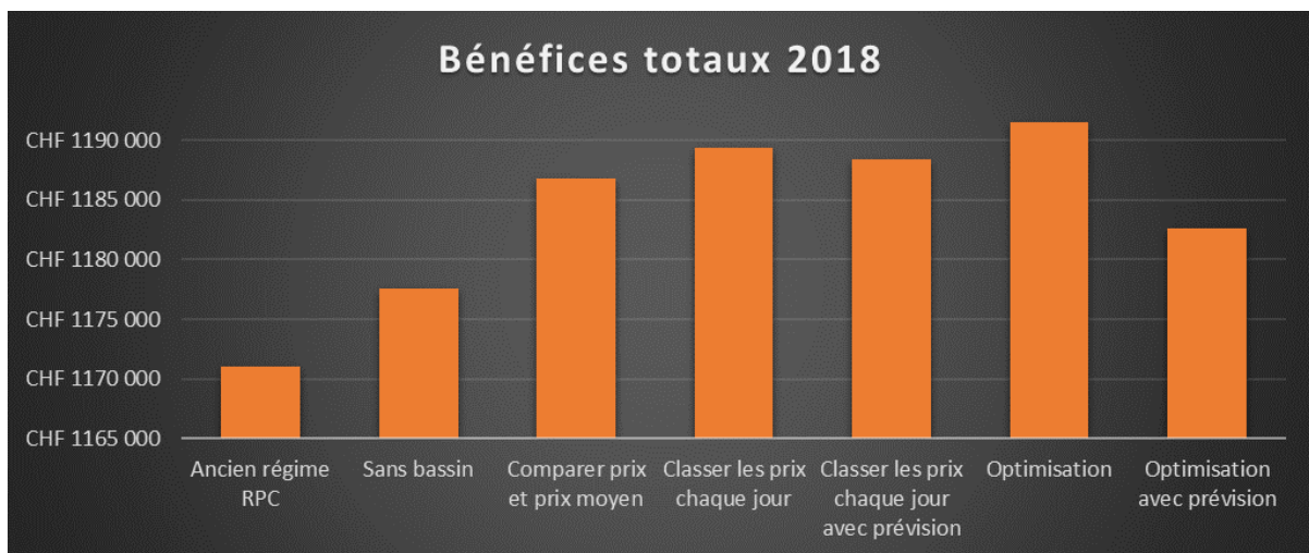
Graphique 19 résultats des simulations optimisées pour 2018 pour P = 200kW et V = 1500m 3
