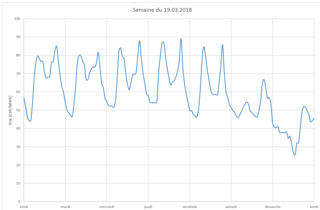
Graphique 4 évolution des prix durant une semaine
