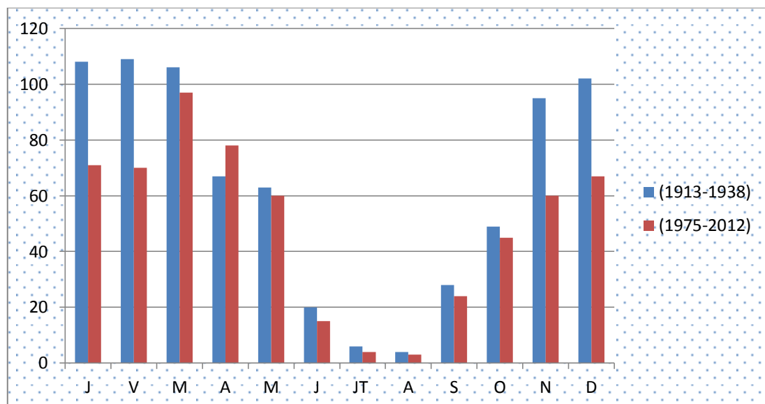
Figure 23 : Variation mensuelle des précipitations au niveau du massif Hafir-Zariffet pour les deux périodes de référence (ancienne et nouvelle).
