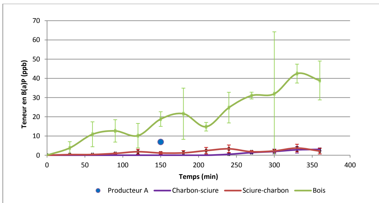
Figure 24 : Evolution de la teneur en B(a)P au cours du fumage
