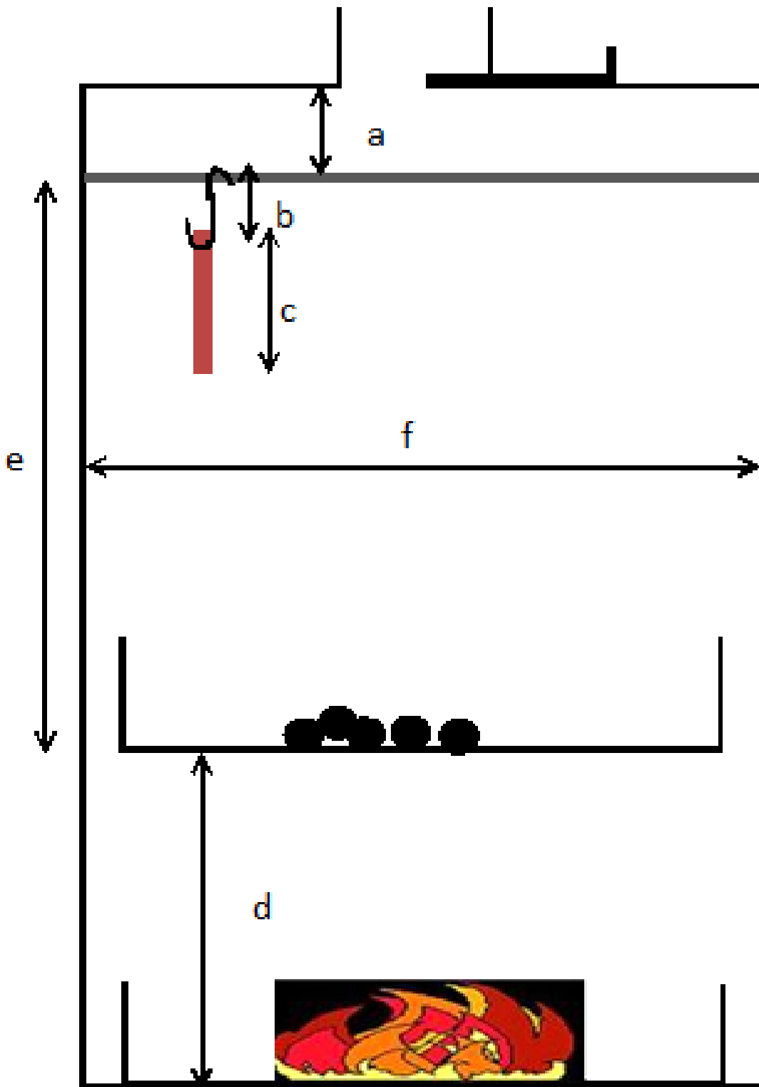
Figure 4 : Représentation schématique du four Capic 35
