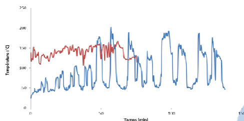
Evolution des températures d'attaque au cours du temps
