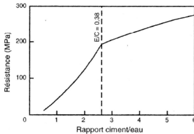
Figure I. 14: Relation entre la résistance calculée d'une pate pure de ciment et le rapport C/E [Nielsen, 1993]
