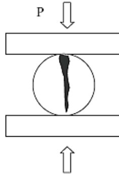
Figure I. 10: traction par fendage
