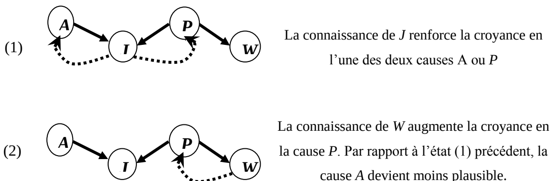
Figure 1-3 : L'information a circulé uniquement dans le sens effet \rightarrow cause . [24]
