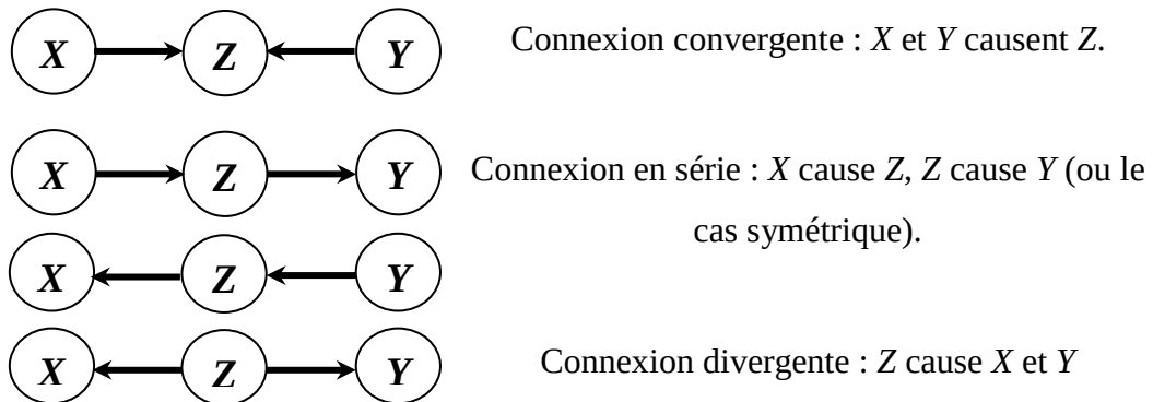
Figure 1-4 : la circulation de l'information dans un graphe causal [24]
