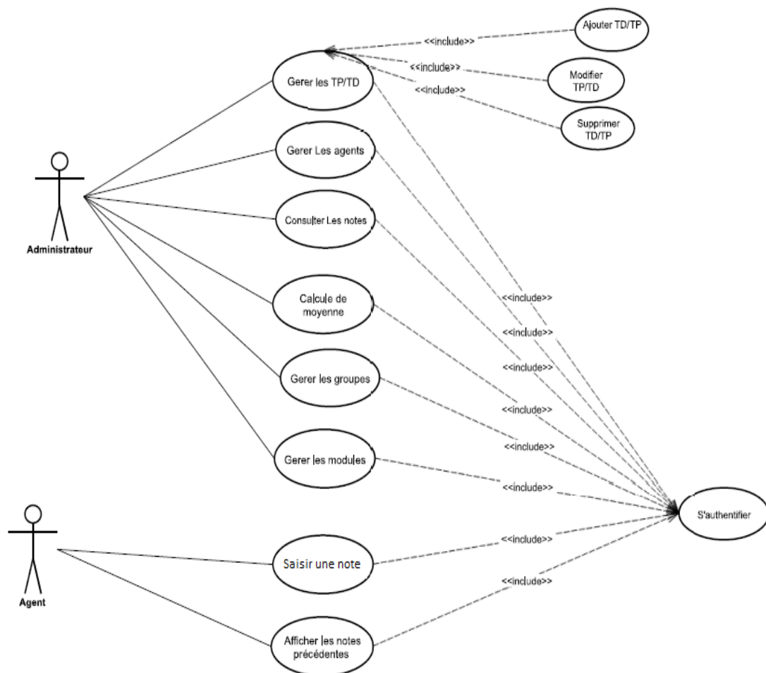
Figure 2 : Cas d'utilisation global
