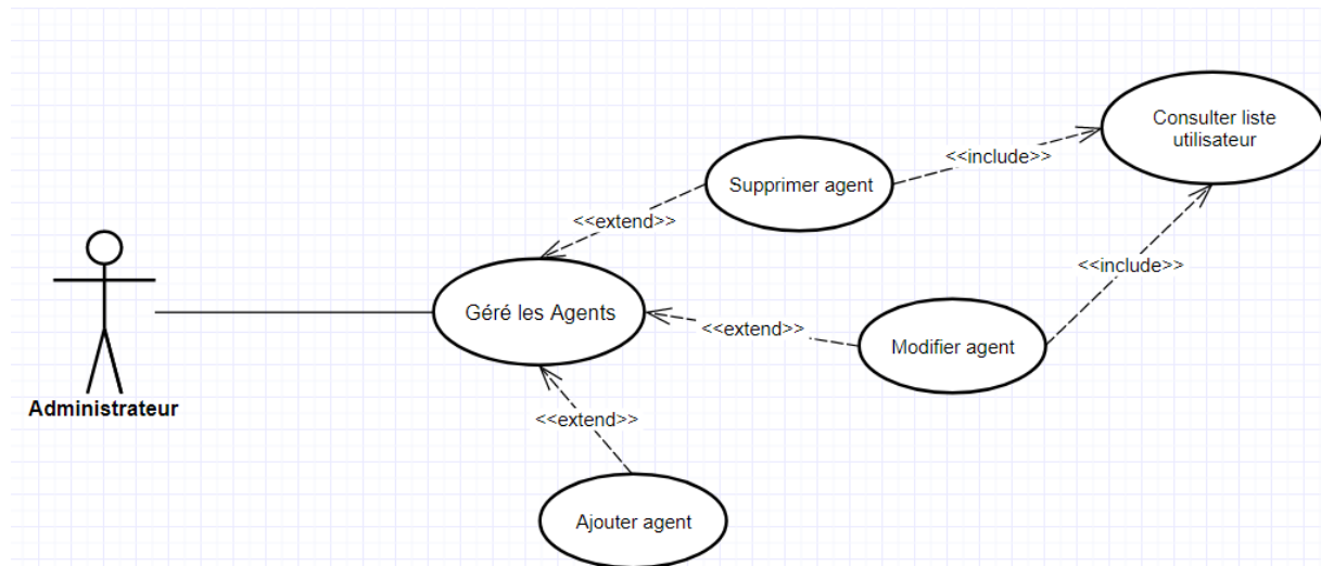
Figure 3: Gérer les Utilisateurs
