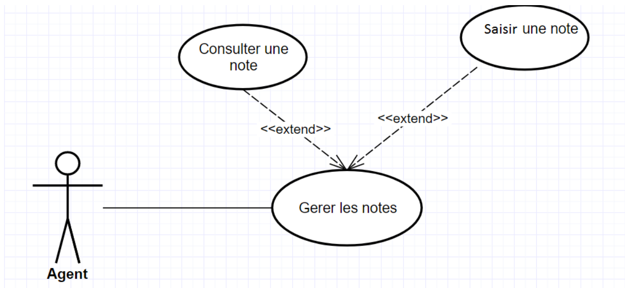
Figure 5 : Gérer les notes
