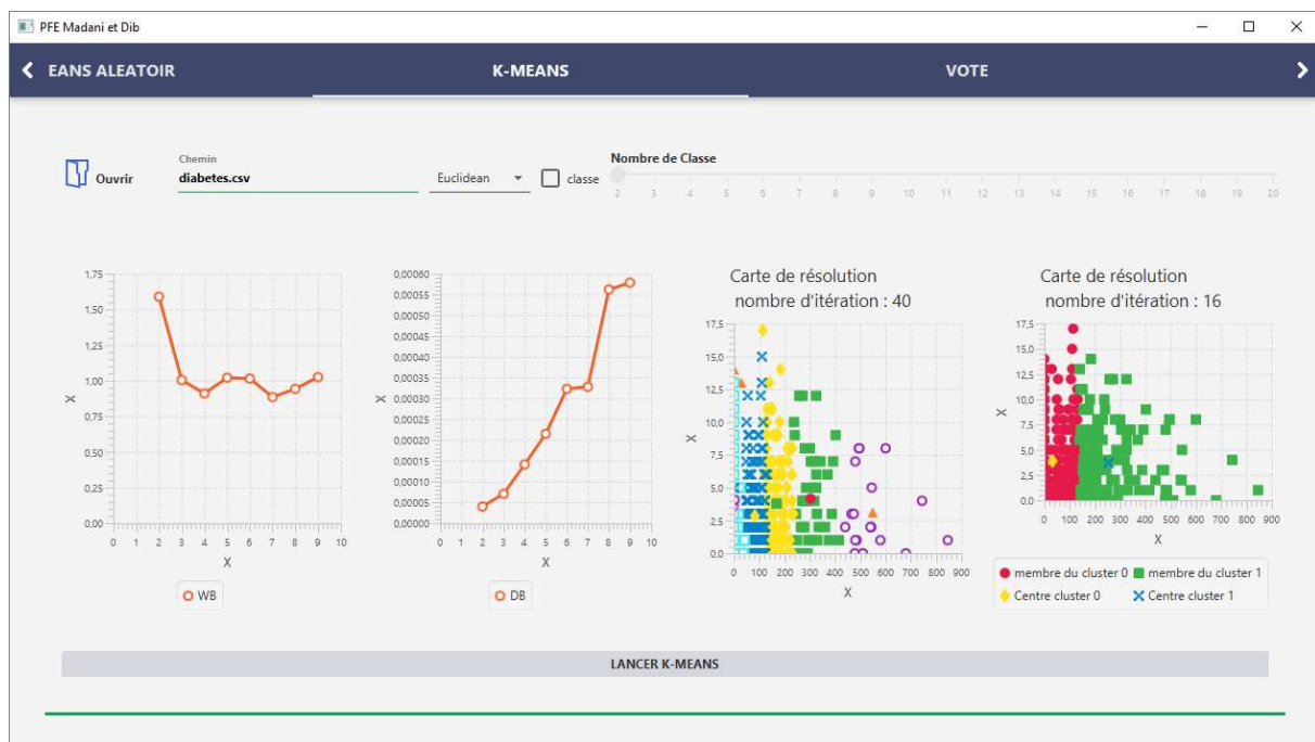
Figure III) 6- résultat du clustering kmeans avec distance euclidien, l'indice WB et DB. Cas K variantes
