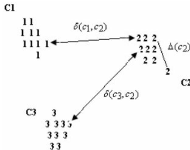
Figure I) 2-l'indice de Dunn
