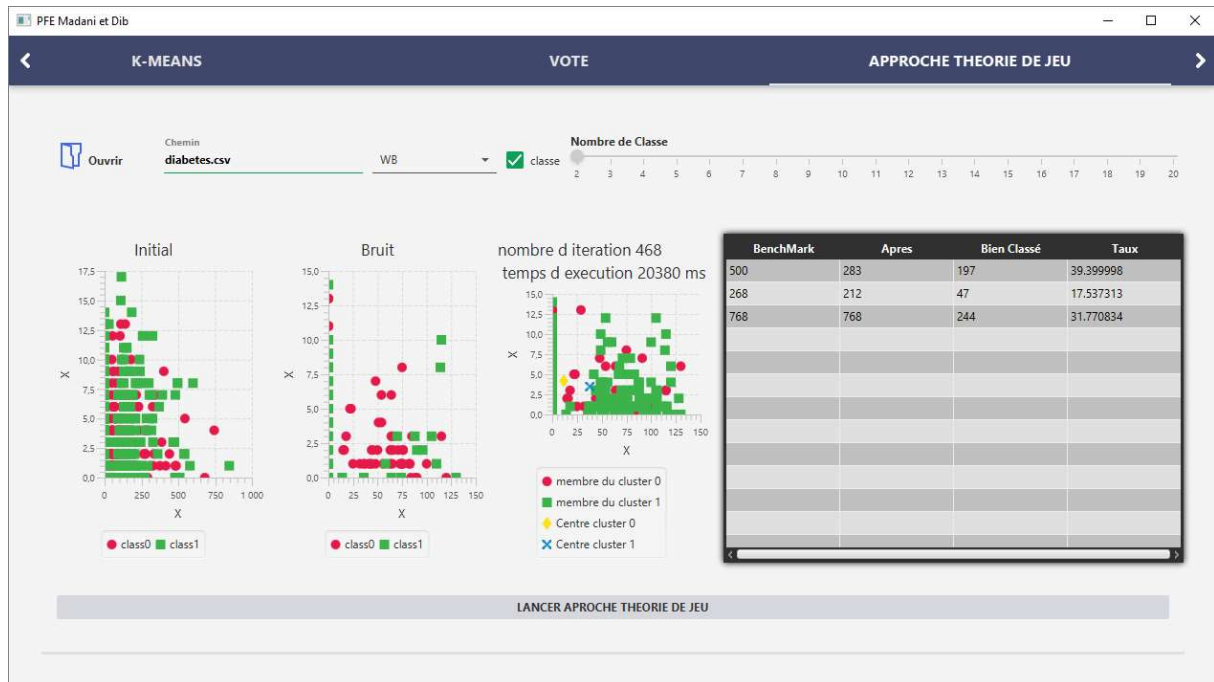
Figure III) 7- résultat du clustering THJ avec l'indice WB et k fixés a 2
