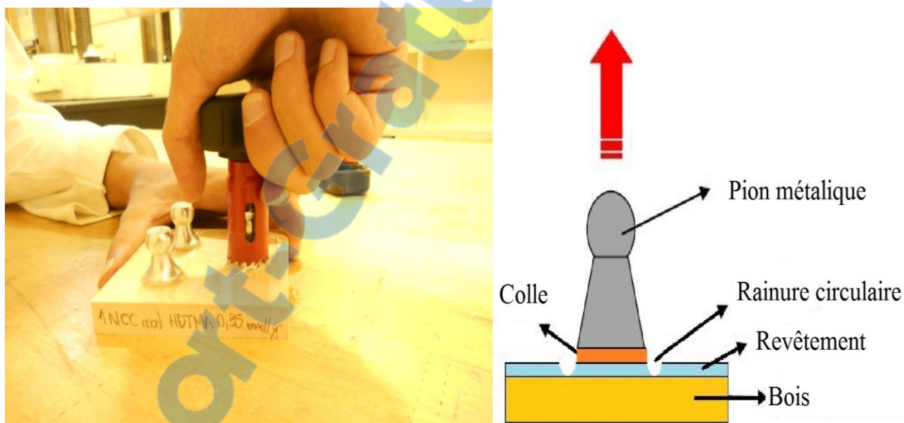
Figure 1.25. Schéma du principe de mesure de l'adhésion.
