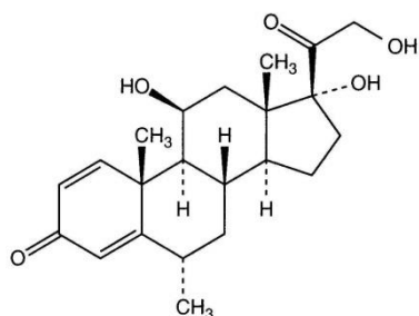
Figure 35 : Molécule de méthylprednisolone.
