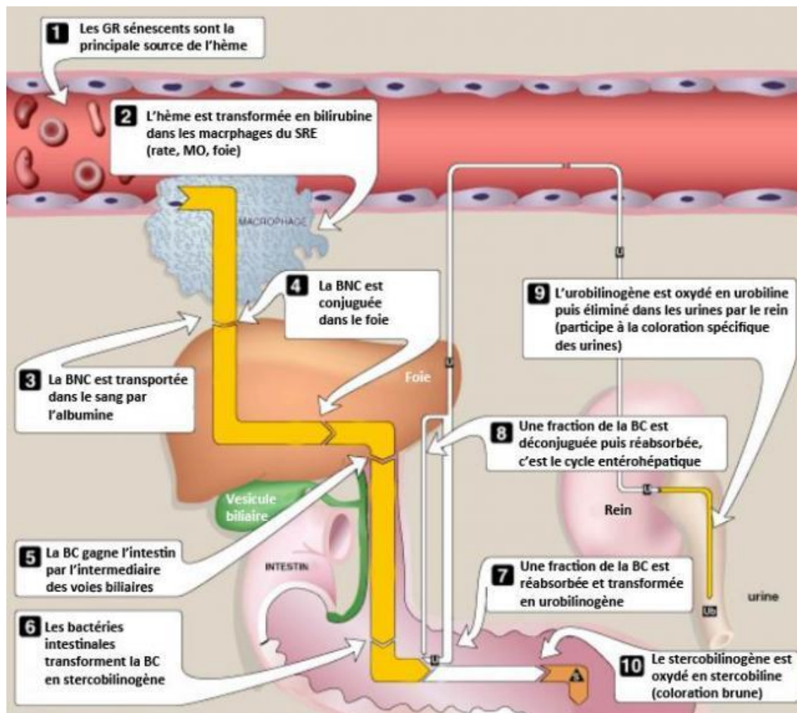
Figure 17 : Formation et transformation de la bilirubine. [24].
