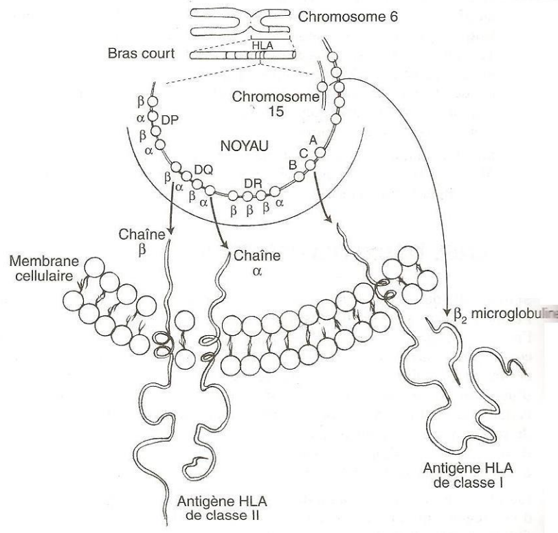
Figure 18 : Organisation du système HLA [4].
