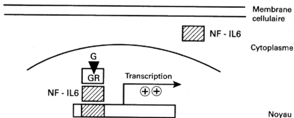
Figure 32 : Action transcriptionnelle indirecte : activation du facteur de transcription NF-IL6 [87].
