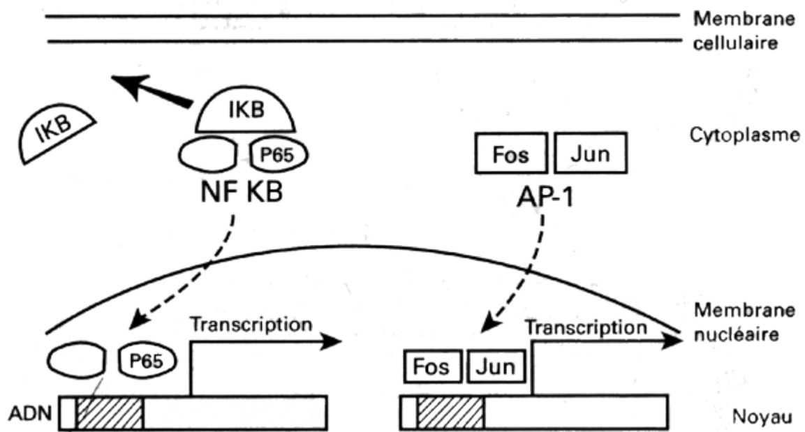
Figure 30 : Action transcriptionnelle indirecte : activation des facteurs de transcription NF-κB et AP-1 [87].
