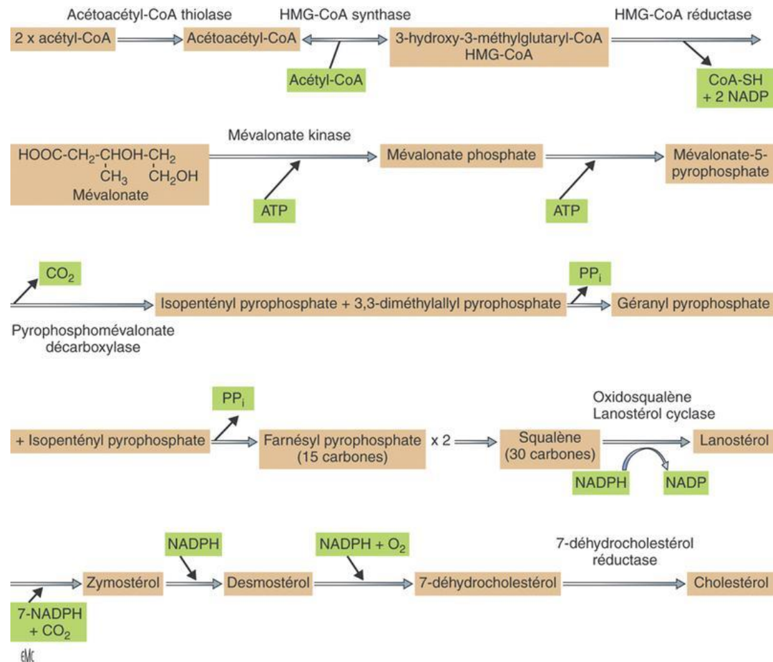
Figure 13 : Synthèse du cholestérol. [8].
