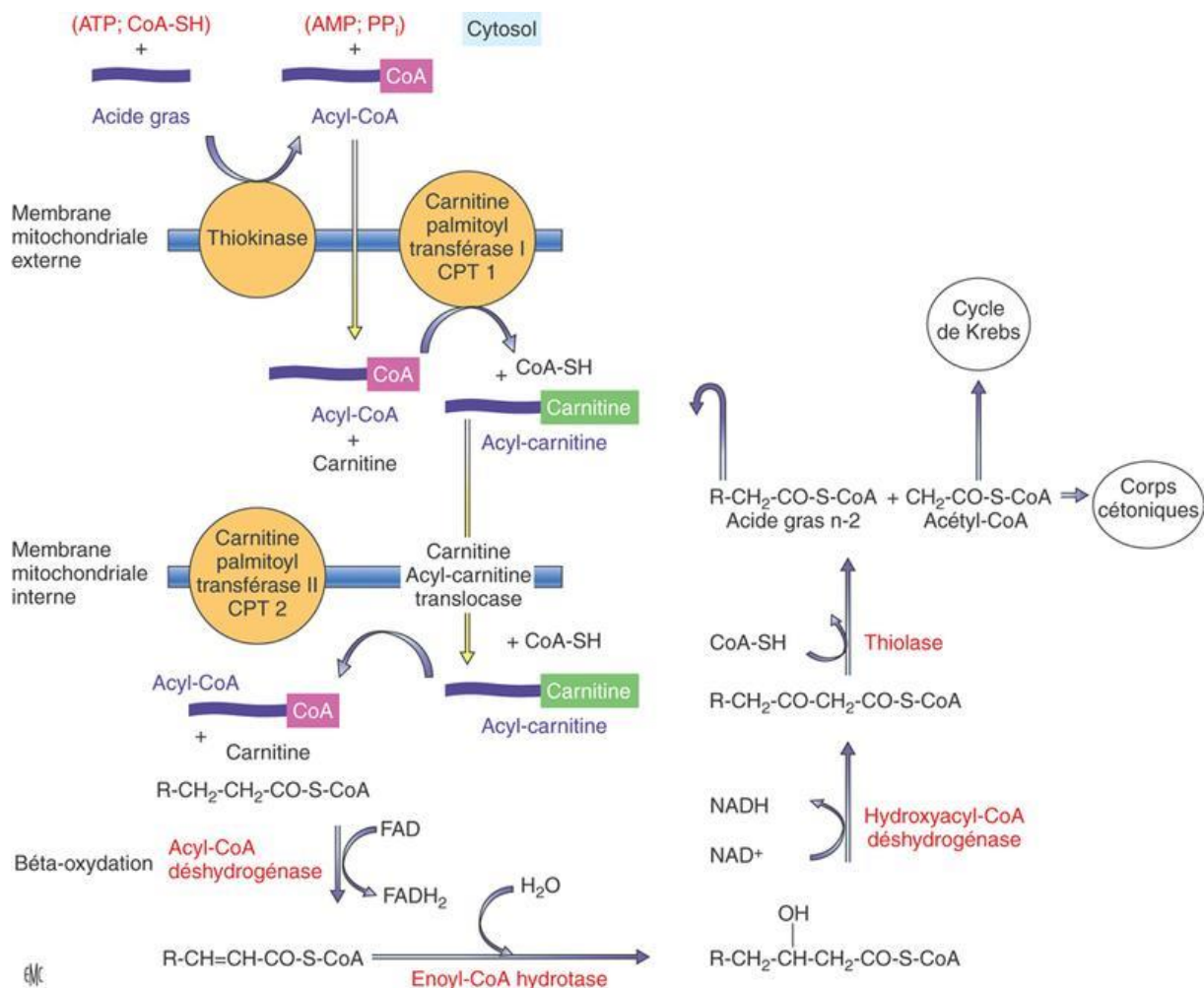
Figure 11 : Transport des acides gras dans la mitochondrie hépatique et \beta -oxydation [8].
