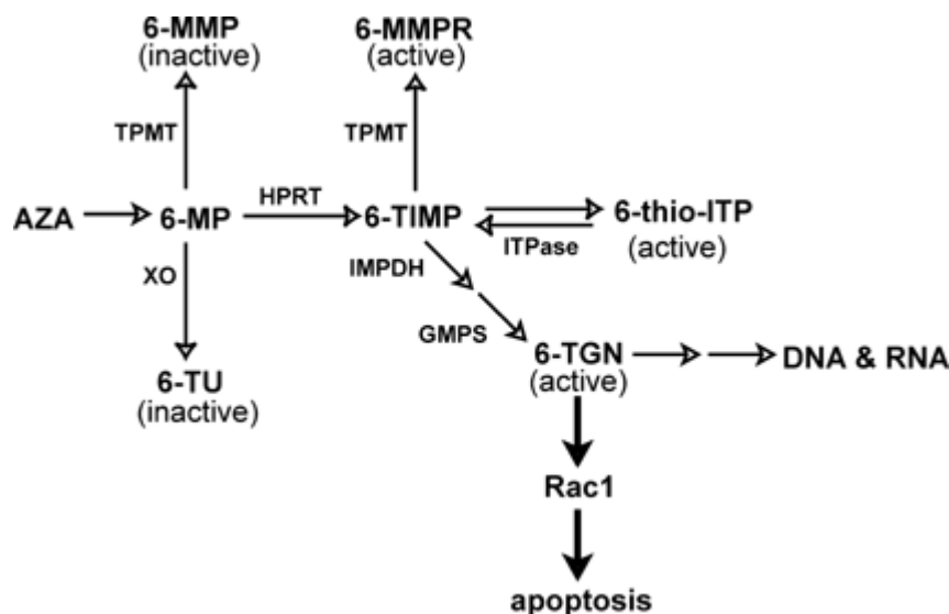
Figure 37 : Action des métabolites de l'azathioprine [92].
