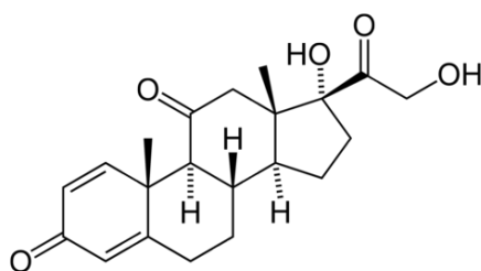
Figure 33 : Molécule de prednisone.
