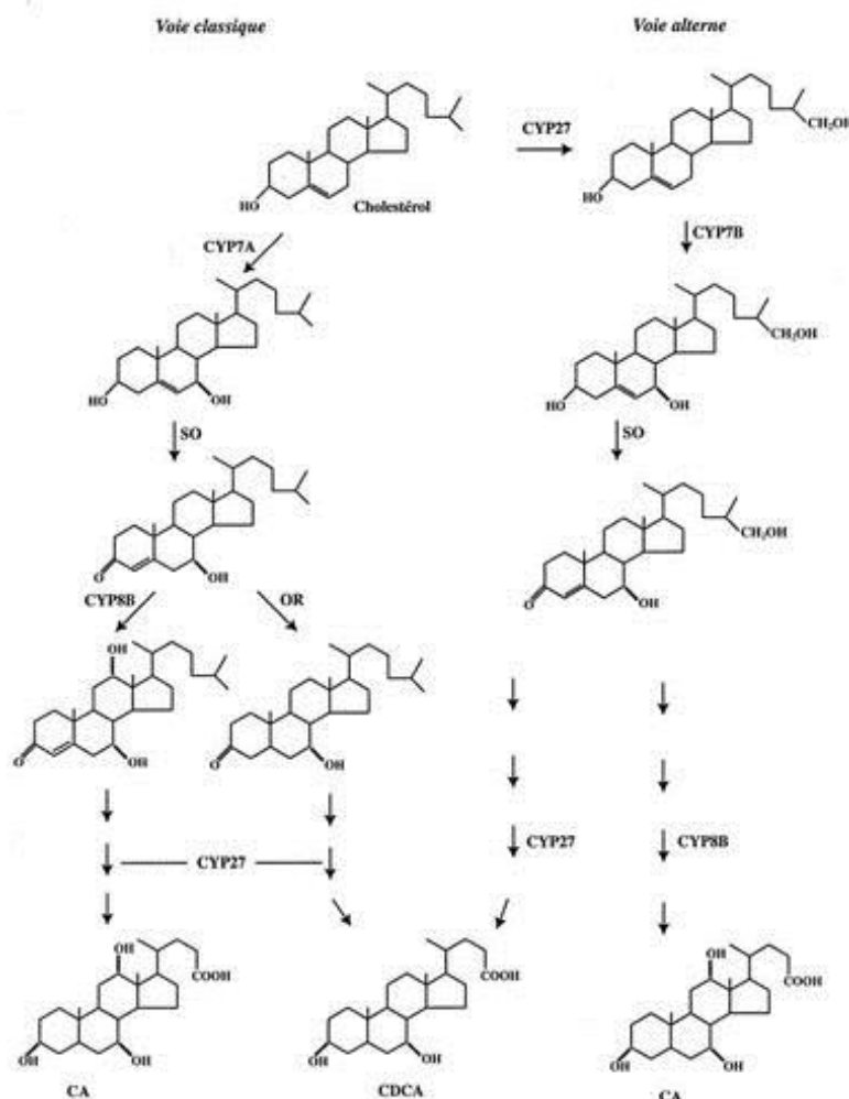
Figure 16 : Formation des acides biliaires à partir du cholestérol [21].
