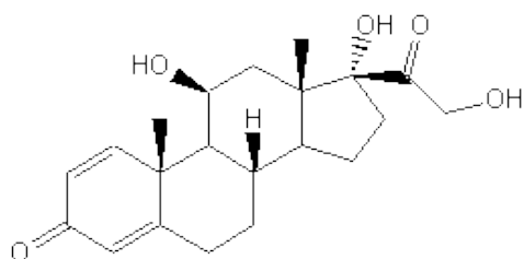
Figure 34 : Molécule de prednisolone.
