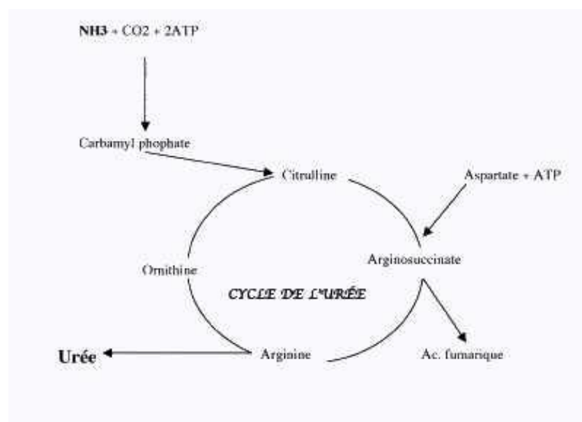
Figure 14 : Le cycle de l'urée [17].
