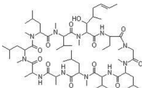
Figure 27 : Molécule de ciclosporine.
