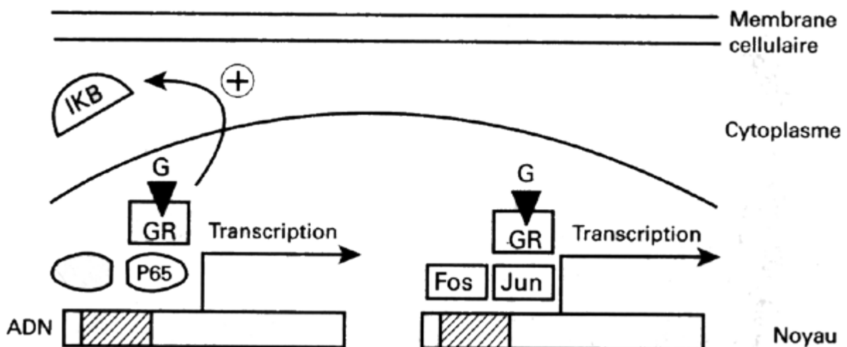
Figure 31 : Action transcriptionnelle indirecte : inhibition des facteurs de transcription NF-κB et AP-1 [87].
