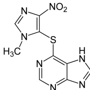
Figure 39 : Molécule d'azathioprine.
