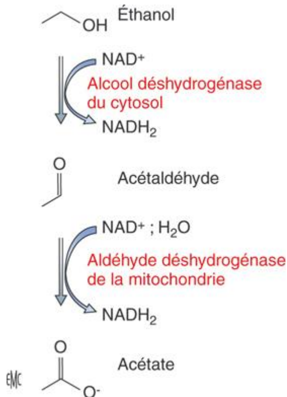
Figure 15 : Oxydation de l'éthanol par le foie [8].
