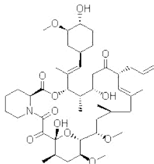
Figure 28 : Molécule de tacrolimus.
