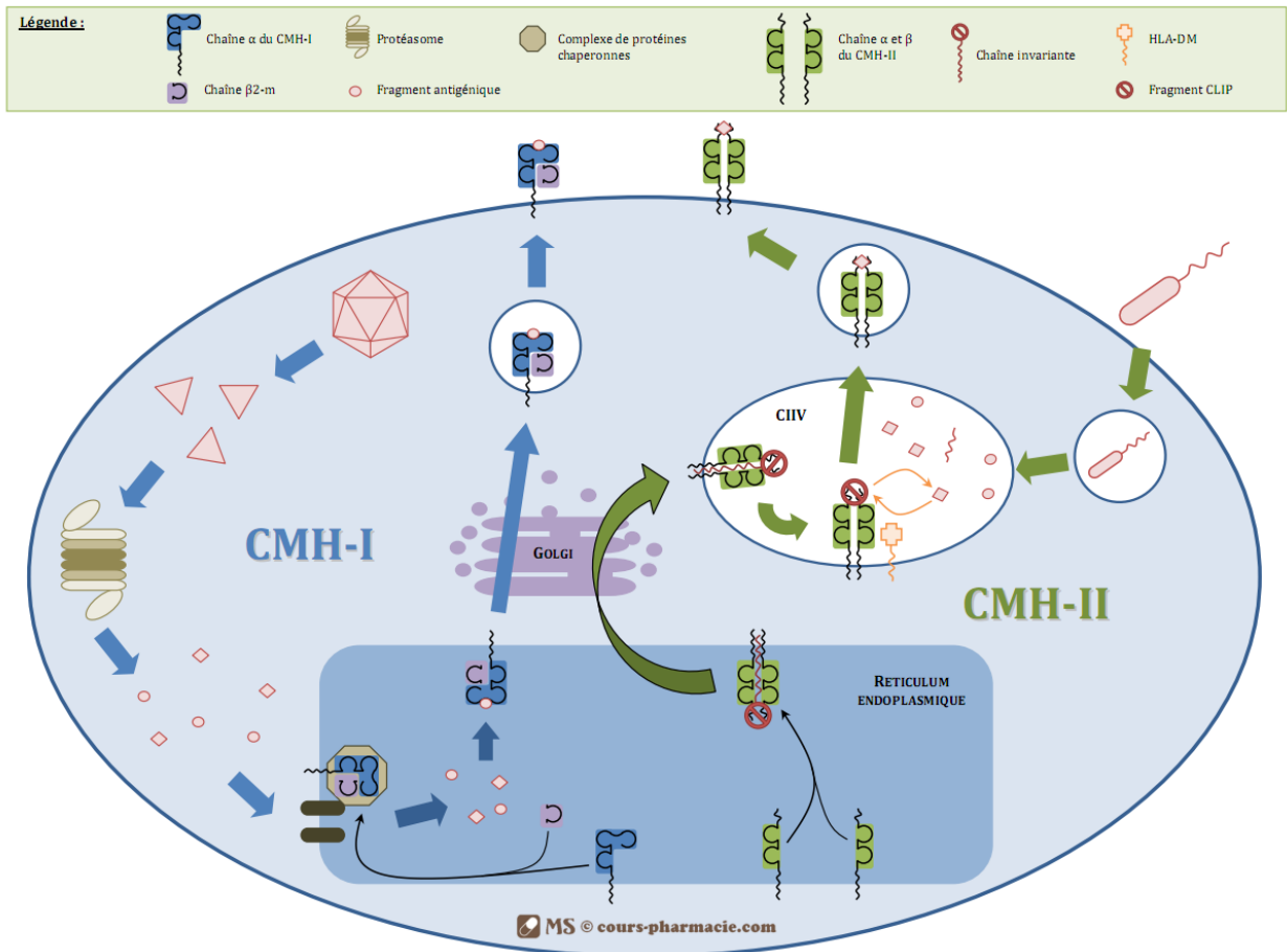
Figure 19 : Prise en charge et présentation des peptides antigéniques par les molécules HLA de classe I et II [52].
