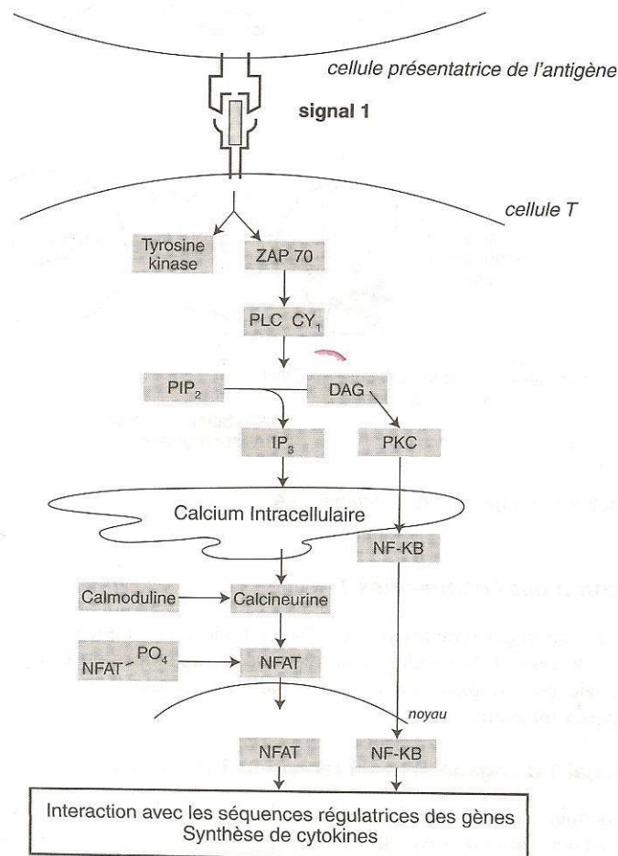
Figure 20 : Signal 1 d'activation du lymphocyte T [4].
