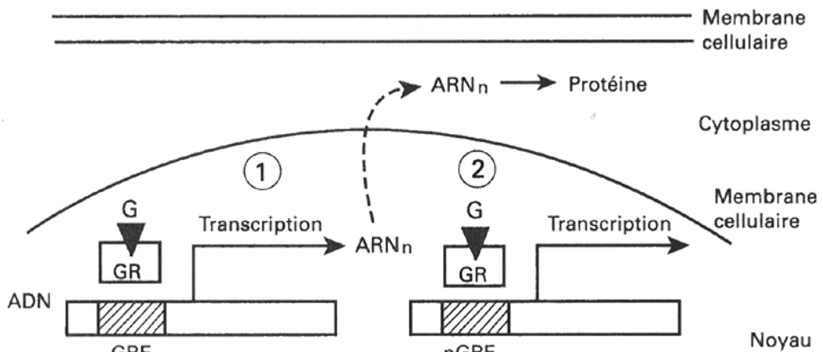
Figure 29 : Action transcriptionnelle directe : effet positif ou négatif [87].
