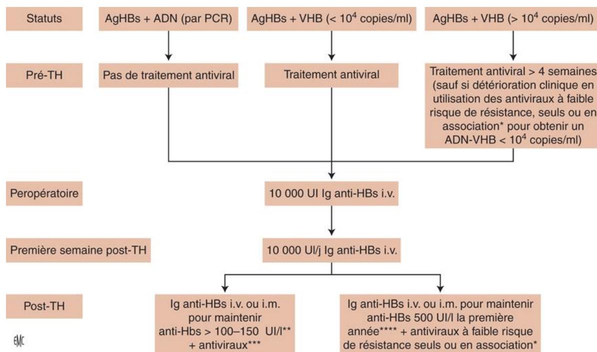
Figure 24 : Prévention de la récurrence virale B post-transplantation hépatique [57].
