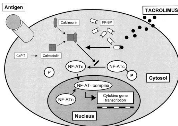
Figure 26 : Mécanismes d'action du tacrolimus [73].
