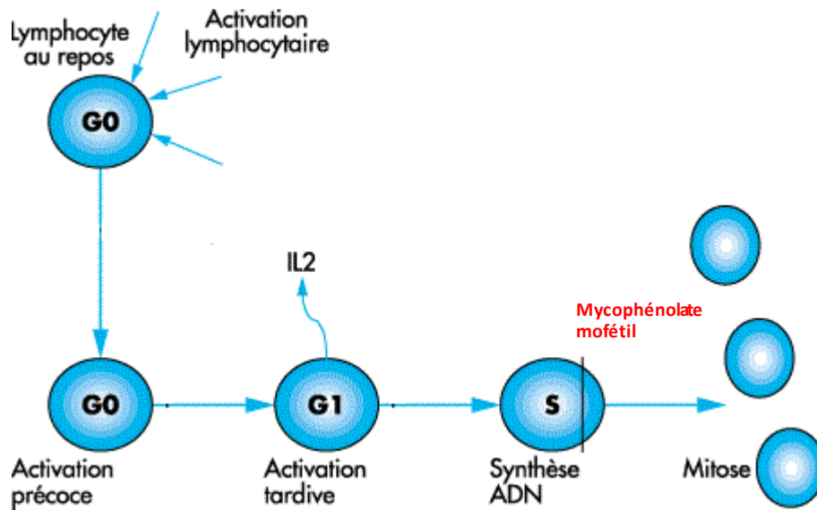
Figure 38 : Mécanisme d'action du mycophénolate mofétil [94].
