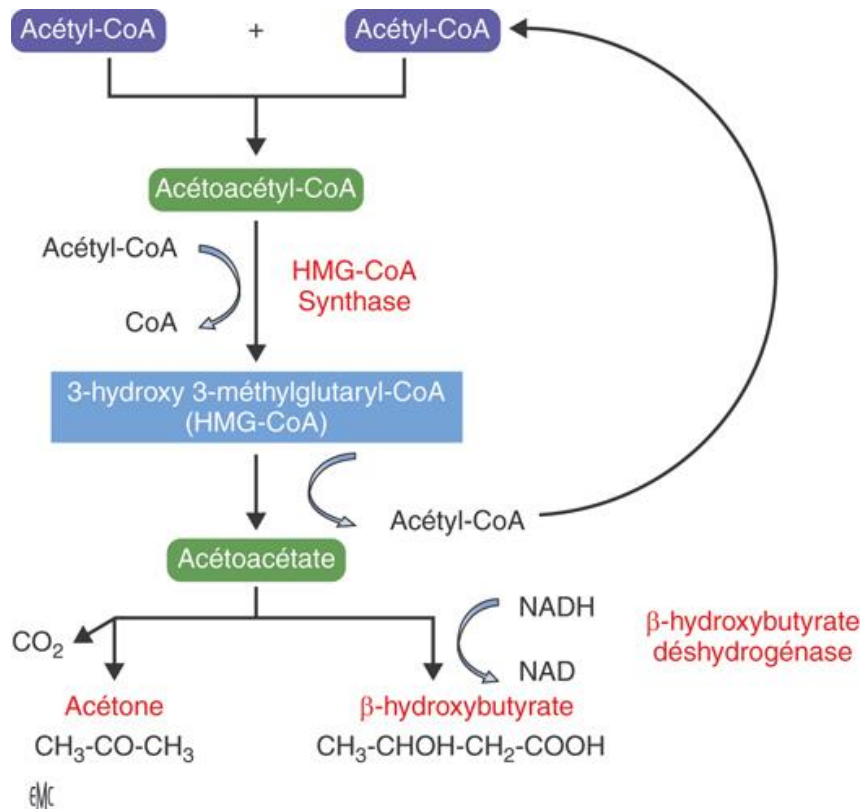
Figure 12 : Formation des corps cétoniques [8].
