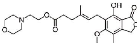
Figure 40 : Molécule de mycophénolate mofétil.
