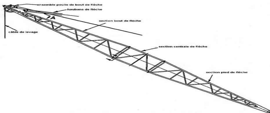
Figure 16 : La flèche
