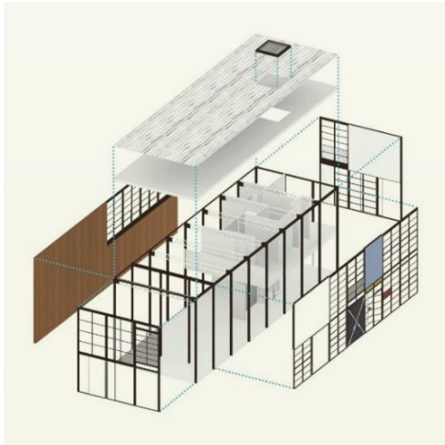
Figure 67 : Axonométrie éclatée_Eames House [Pin21?].
