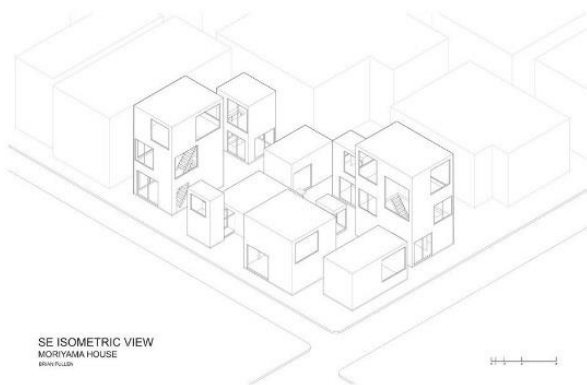
Figure 18 : Axonométrie_ Moriyama House [Pin21].
