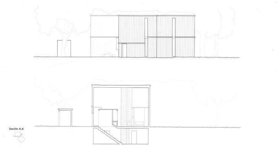
Figure 75 : Coupes et élévations_Fisher House [Gal21].
