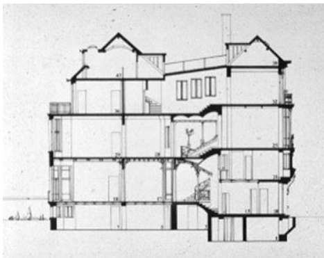
Figure 54 : Coupe_ Hôtel Tassel [Coh19].
