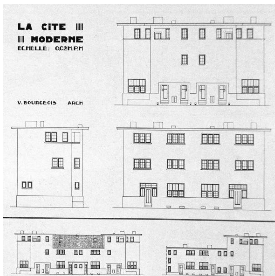
Figure 7 : Elévations_ La Cité Moderne [Coh19].
