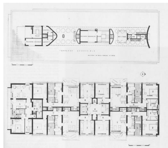
Figure 87 : Plan_Cité de Droixhe_[Coh19].
