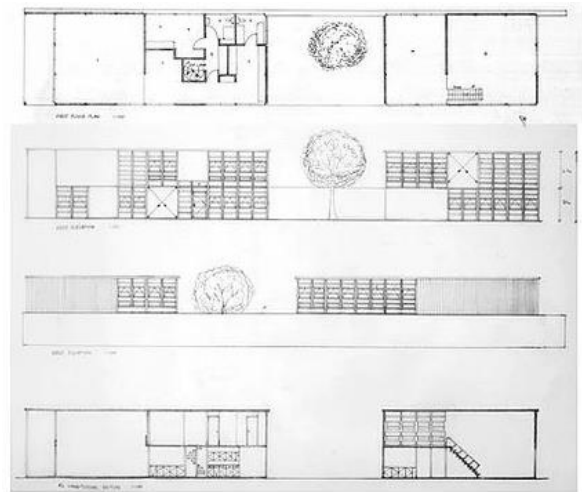
Figure 68 : Plan, coupes et élévations_Eames House [Min21].
