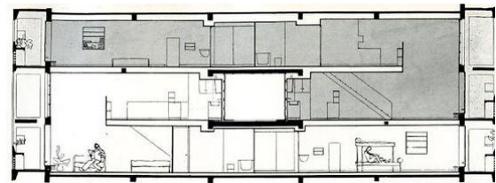
Figure 83 : Coupe_ La Cité Radieuse [Pin21].
