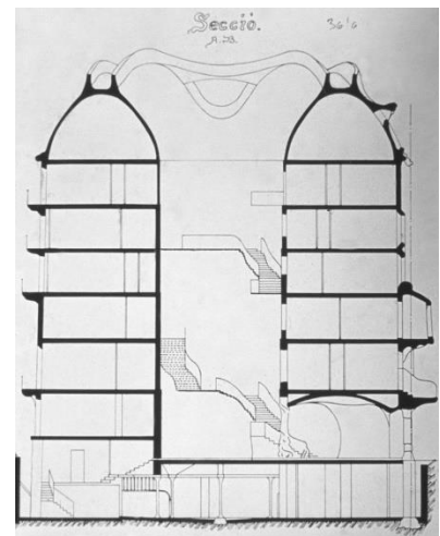
Figure 60 : Coupe_ Casa Milà [Ker21].
