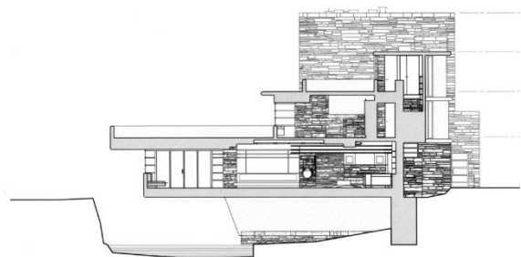
Figure 64 : Coupe_Fallingwater [BP19].
