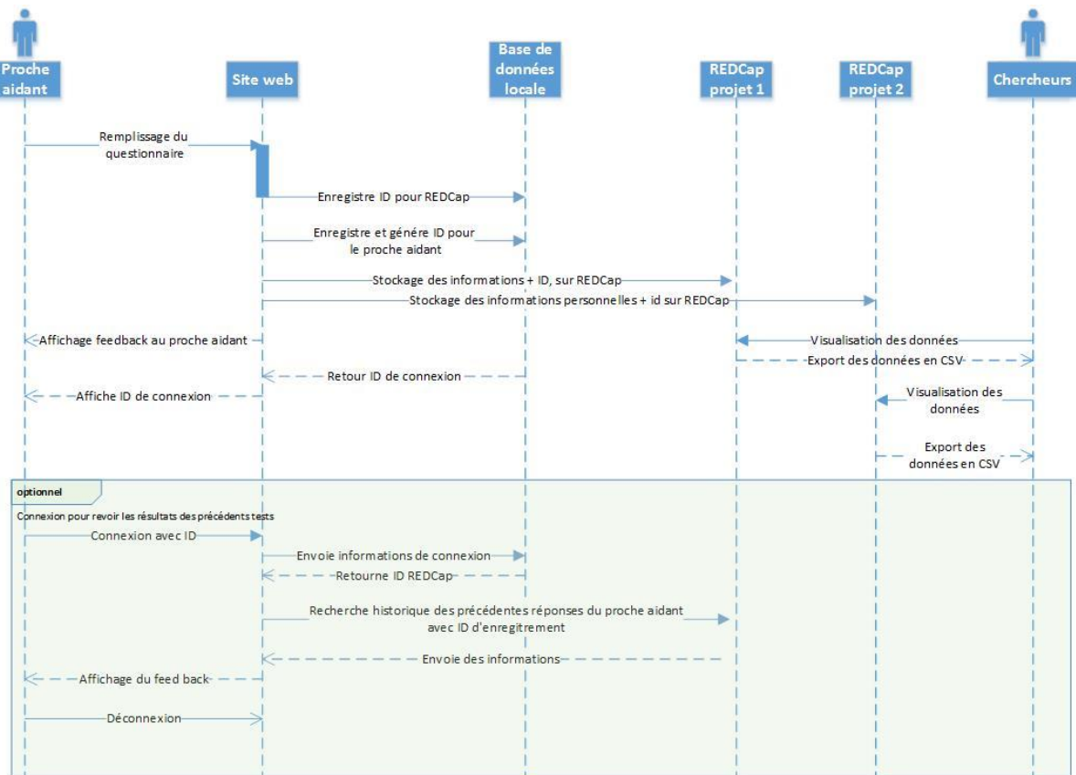
Figure 14 Diagramme de séquence après rencontre avec Fabien (Source : auteur)
