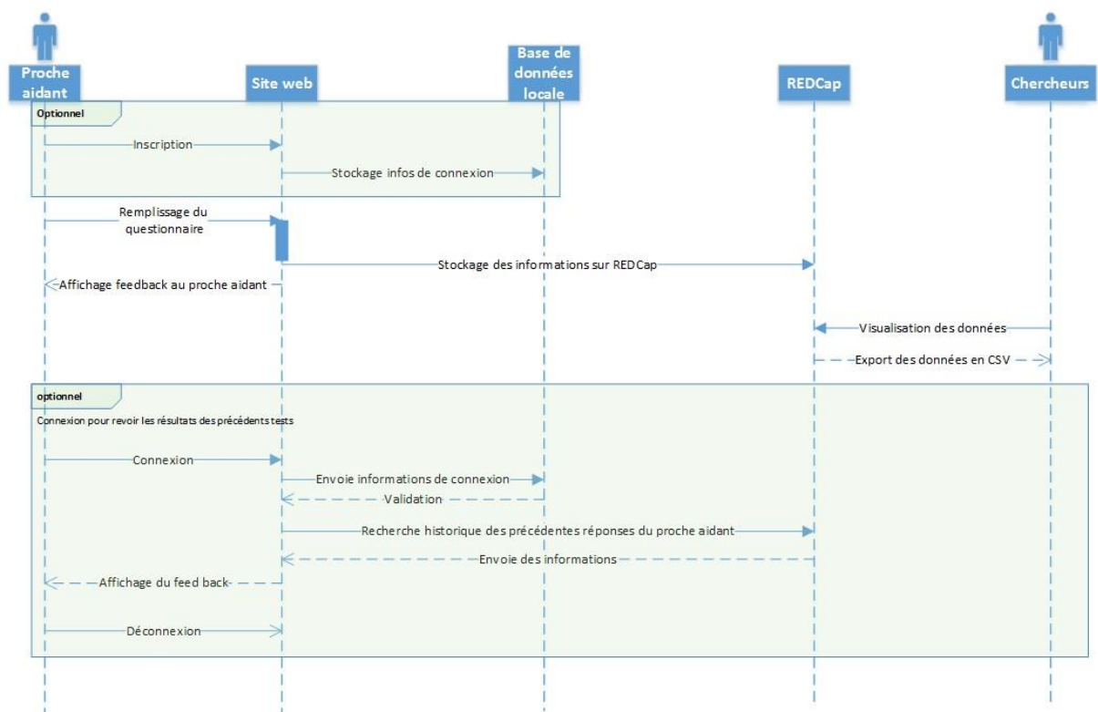
Figure 10 Premier diagramme de séquence. Accès libre au site (Source : auteur).
