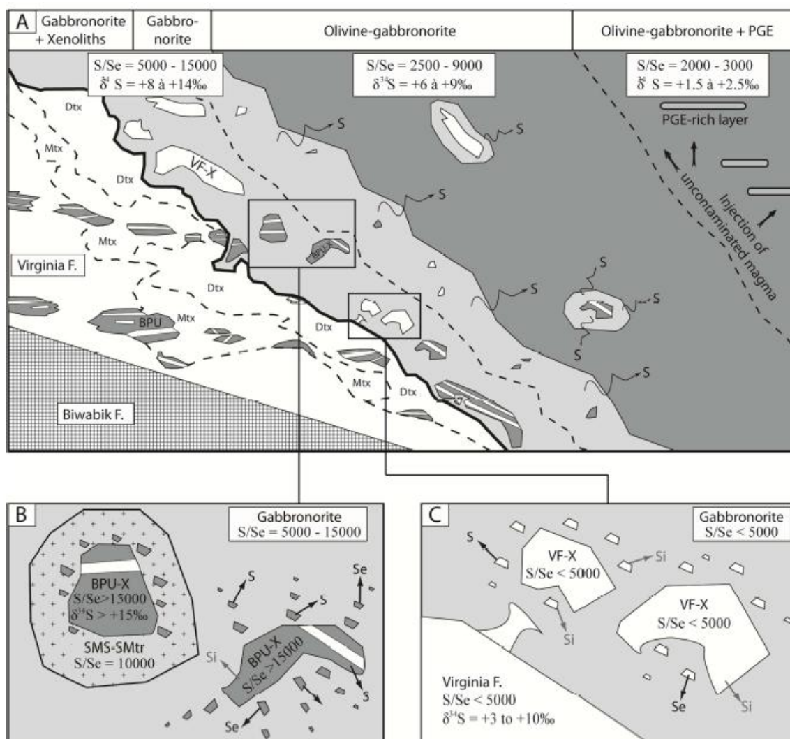
Figure 1.4: Modèle de contamination en S du magma par assimilation in-situ de xénolithes de roches sédimentaires de la BPU (Bedded Pyrrhotite Unit) (Modifiée d'après Queffurus et Barnes, 2014). Abréviations : VF-X=Xénolithes de la Formation de Virginia non issus de la BPU; BPU-X=Xénolithes de la Bedded Pyrrhotite Unit; Mtx=Métatexites; Dtx=Diatexites; SMS-SMtr=Sulfures massifs et matriciels.
