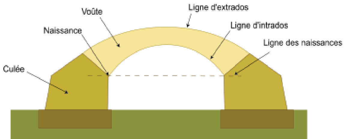
Figure 8 : Pont à voutes en maçonnerie
