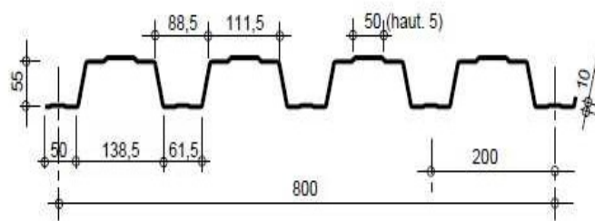
Figure IV. 1: Caractéristiques géométriques de la tôle HI Bond 55-800
