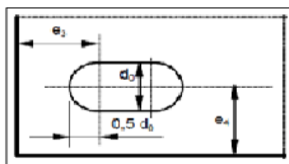
Figure 2.5. Pince longitudinale et pince transversale pour trous oblongs
