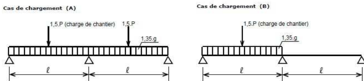
Figure IV. 3: Représentations des Cas de charge
