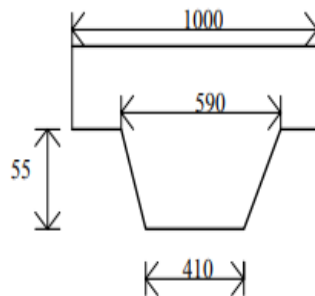
Profil HI BOND 55-750
