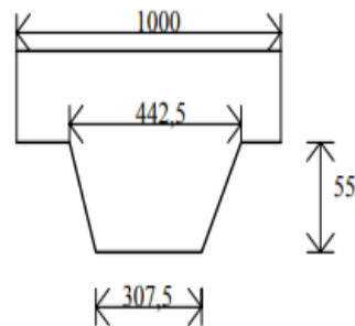
Profil HI BOND 55-800
