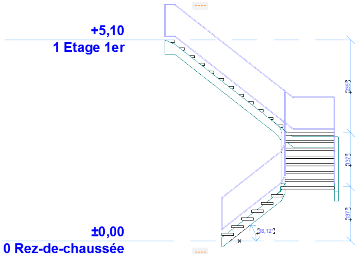
Figure VI.6: le choix des dimension d'escaliers entre étage.
