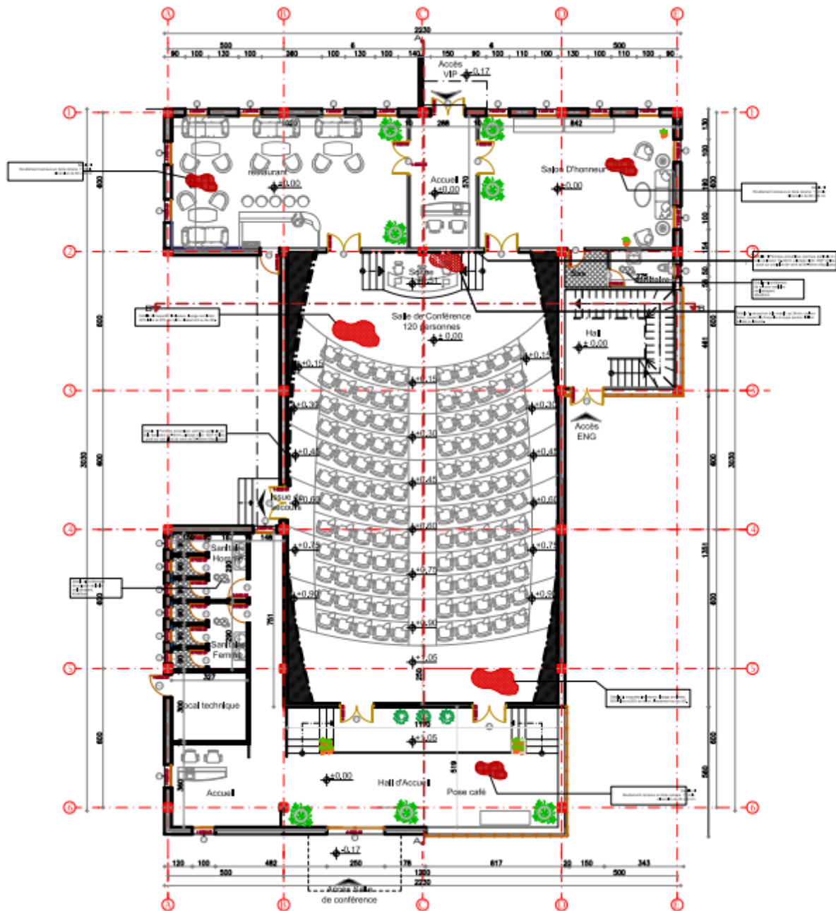
Figure I.9: Plan du RDC.
