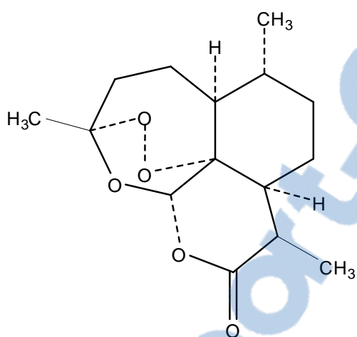
ARTEMISININ
