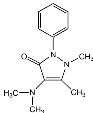
Pyramidon
