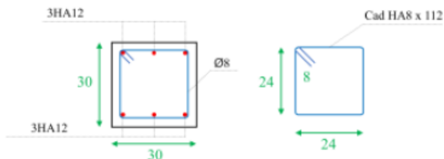
Figure V-3: Ferrailage longitudinal et transversal des poteaux
