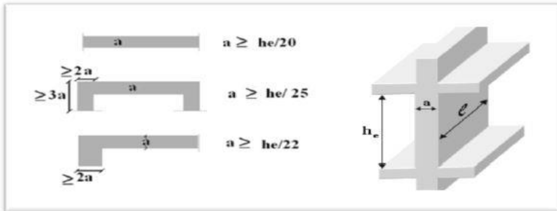
Figure III-2: Section réduite du voile
