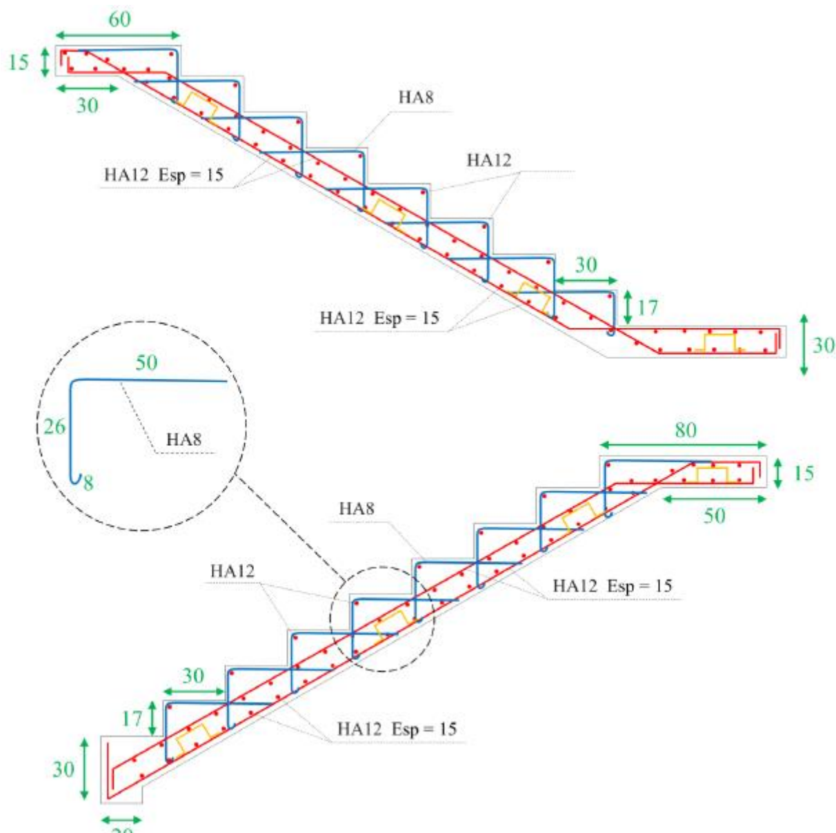
Figure V-12: Ferrailages longitudinal et transversal des escaliers
