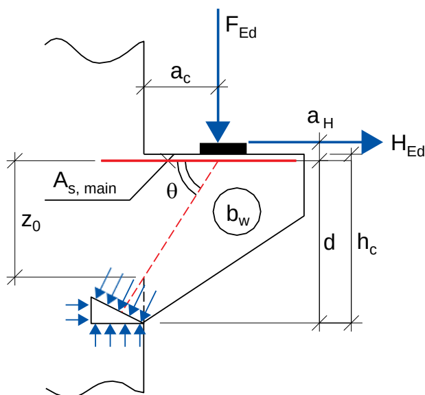
Figure V-4: Résultante des forces agissantes sur le corbeau
