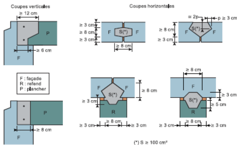
Figure I-2: liaisons continues bétonnées sans armature en attente
