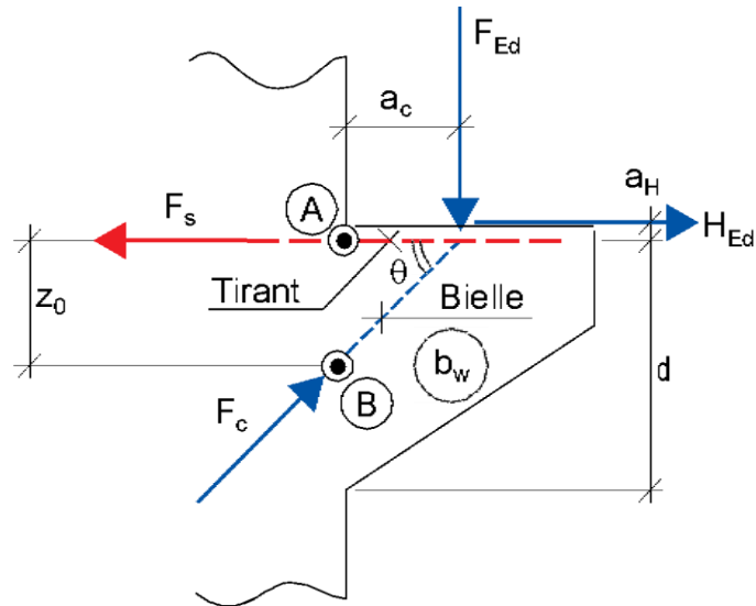
Figure II-2: Résultante des forces appliquées sur le corbeau
