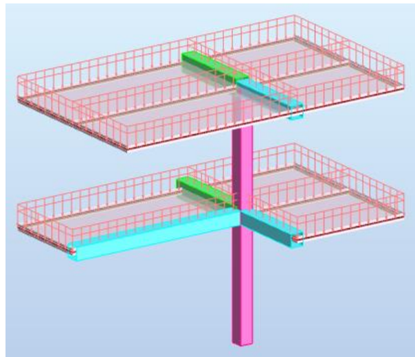
Figure III-1: Poteau le plus sollicité
