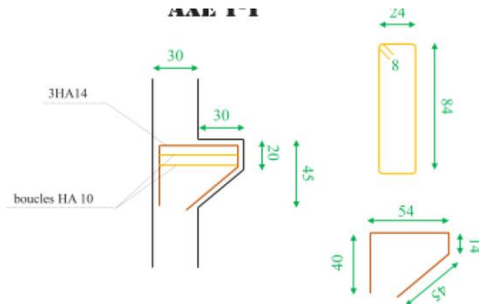
Figure V-6: Ferrailages longitudinal et transversal des corbeaux PT01
