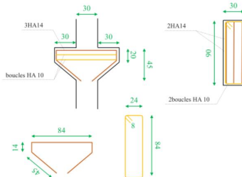
Figure V-6: Ferrailages longitudinal et transversal des corbeaux PT01
