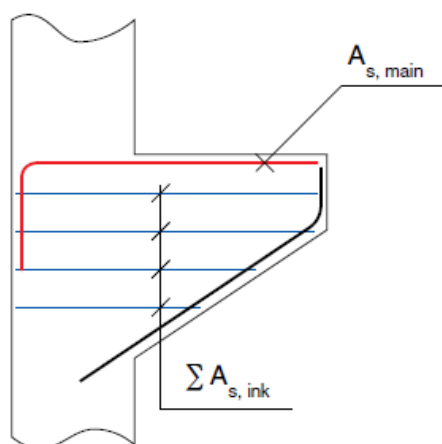
Figure V-5 : Répartition des armatures sur le corbeau
