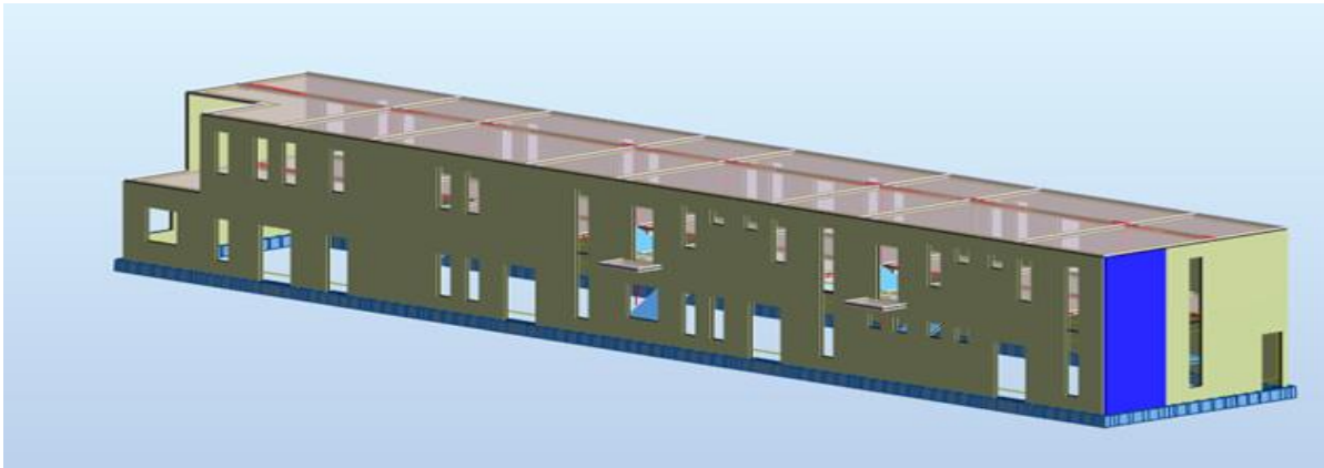
Figure V-8: Exemple de voile calculé
