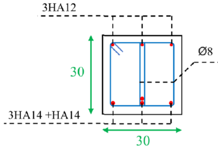
Figure V-1: Ferrailages longitudinal et transversal des poutres PO01/PO03
