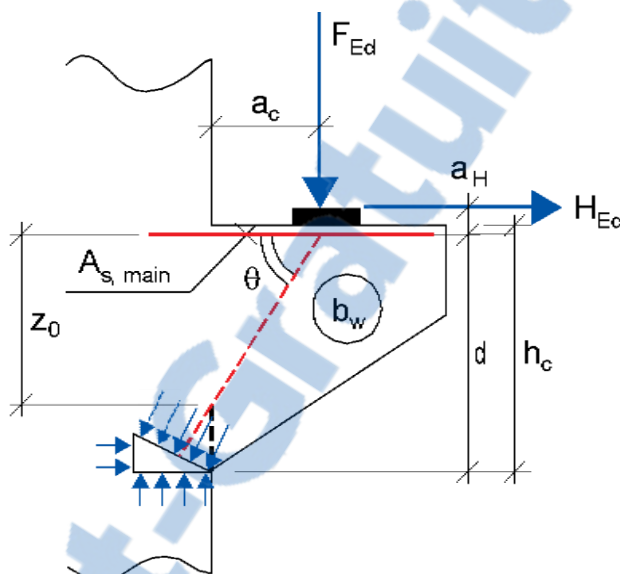
Figure II-1: Résultante des forces appliquées sur le corbeau
