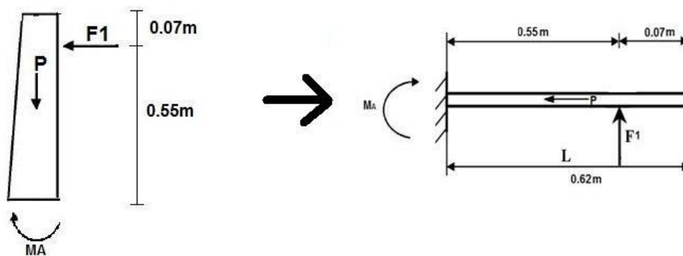
Figure II-5: Forces et moments agissants sur le fut d'encuvement
