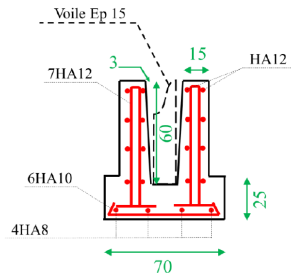
Figure VI-4 : Dessin de ferrailage de semelle filante et le fût d'encuvement
