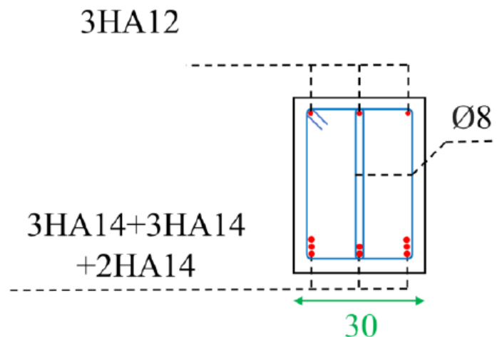
Figure V-2: Ferrailages longitudinal et transversal des poutres PO02/PO04
