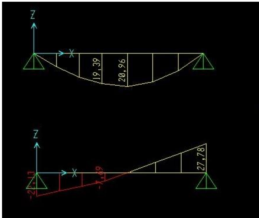
Figure V-10: Diagramme des sollicitations (ELU).
