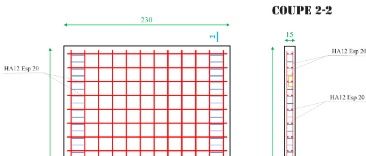
Figure V-9: Ferrailages longitudinal et transversal des voiles
