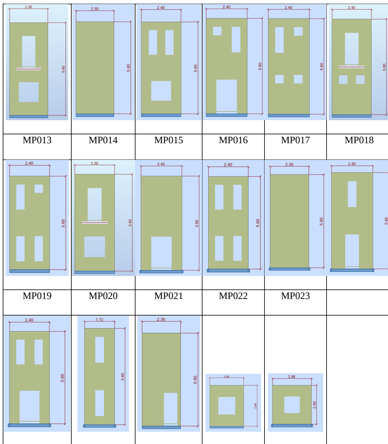
Figure III-4: types de voiles
