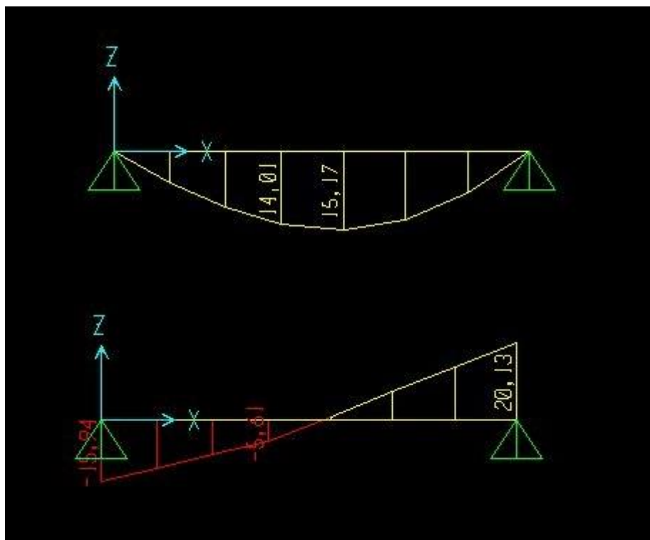
Figure V-11: : Diagramme des sollicitations (ELS).
