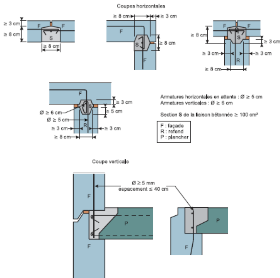
Figure I-3: liaisons continues bétonnées avec armatures en attente
