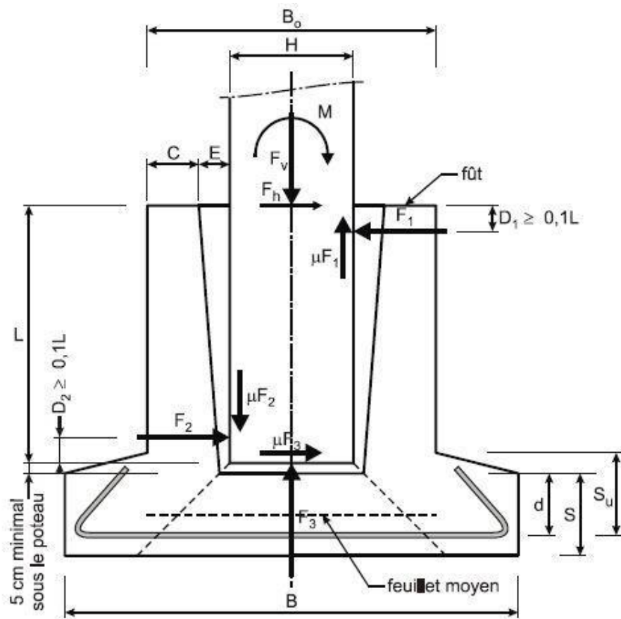
Figure VI-2 : Schéma descriptif du fut d'encuvement
