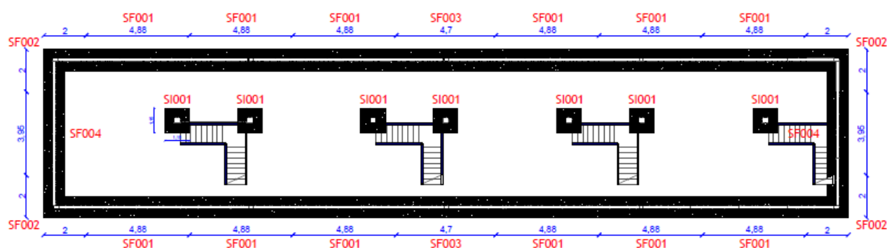
Figure VI-1 : Schéma descriptif des semelles
