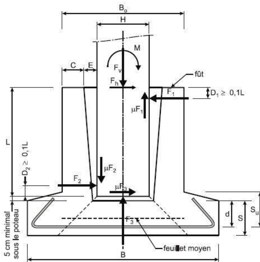
Figure II-4: Schéma descriptif du fût d'encuvement
