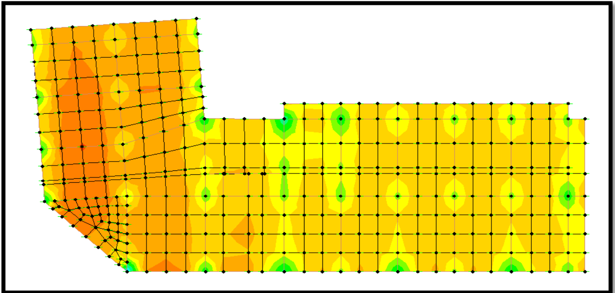
Figure.7.1 Moments M11 a l'ELU.
