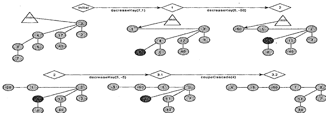
Figure 40 : Opération Decrease-key
