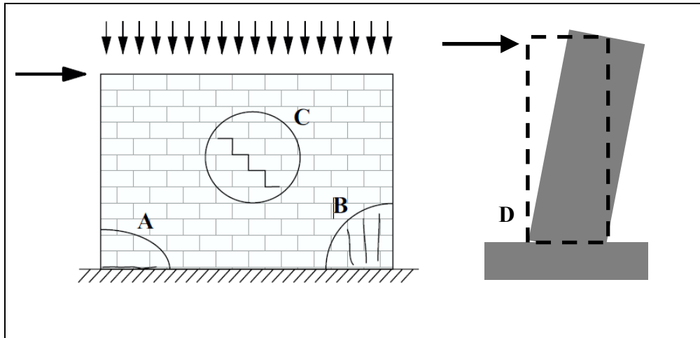
Figure 1.16 Différents modes de rupture des murs de maçonnerie, A : Rupture par glissement dans les joints, B : Rupture par écrasement du pied du mur, C : Rupture par traction diagonale, D : rupture par balancement Tirée de Lang (2002)
