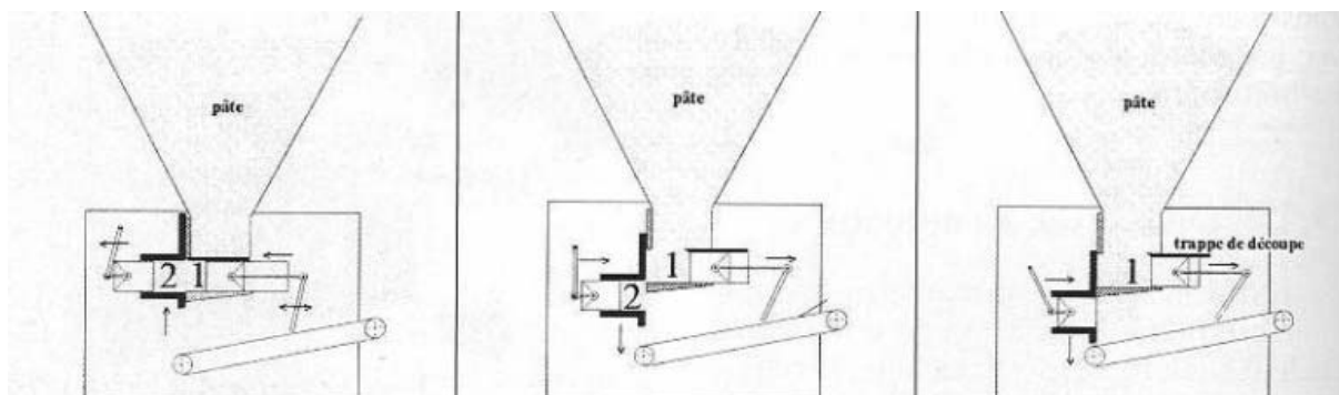
FIGURE 25 : FONCTIONNEMENT D'UNE DIVISEUSE A TIROIRS (d'après [6])
