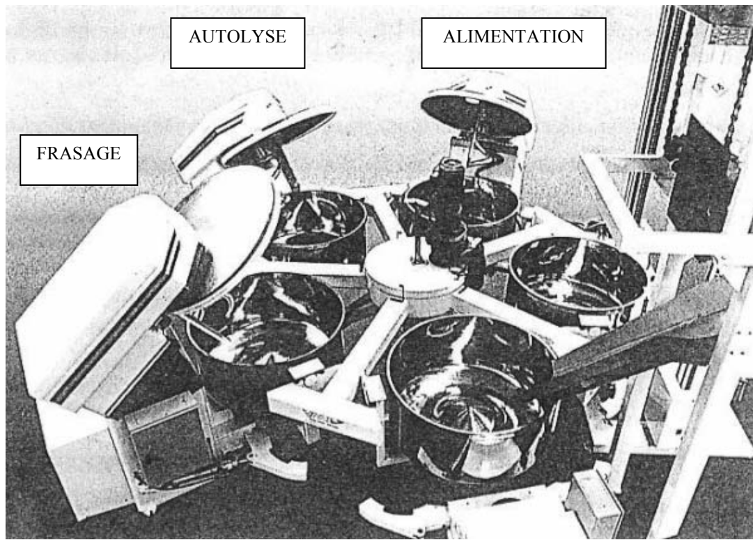
FIGURE 24 : FONCTIONNEMENT D'UN CARROUSEL DE 5 PETRINS (d'après [6])
