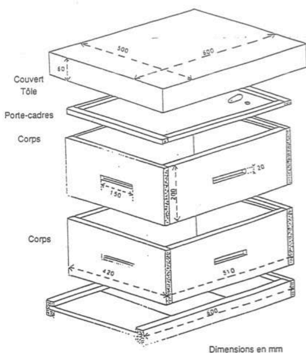
Figure 24 : Les dimensions de la ruche Bourbon (Megret, 1986)
