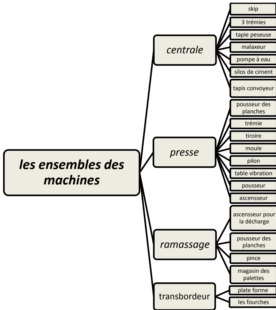
Schéma 4 : les ensembles et les sous-ensembles des machines
