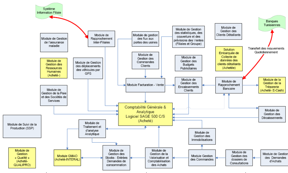
Figure 1.3 : Architecture du système d'information actuel
