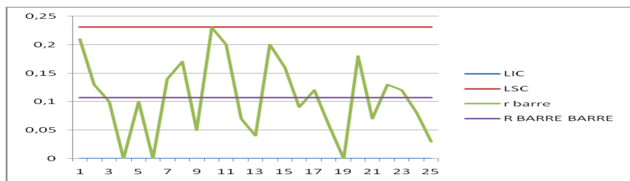
Figure 2 illustrant la carte de contrôle pour l'étendue :
