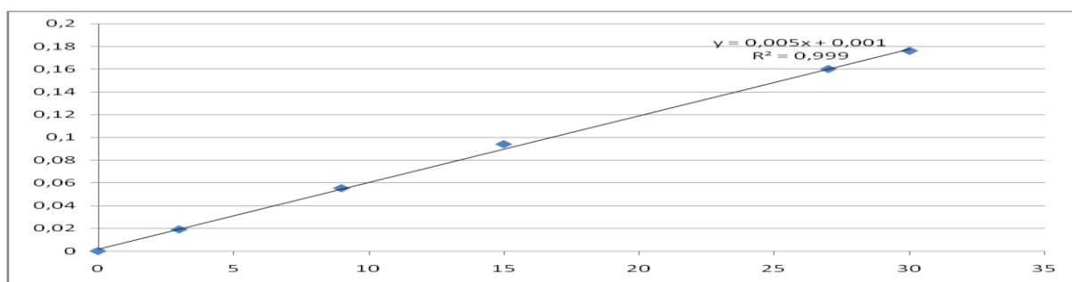
figure 2 : la courbe d'étalonnage en fonction de la densité optique et la concentration en (SO_4)^{2-}
