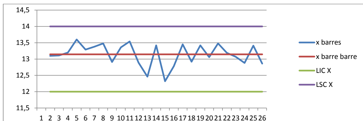
Figure 2 illustrant la carte de contrôle pour la moyenne :
