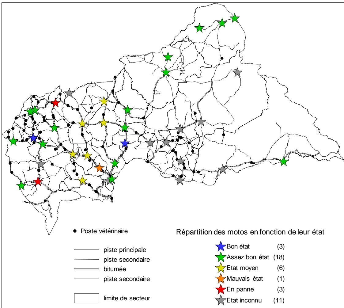
FIGURE 20 : RÉPARTITION DES MOTOCYCLETTES DU PARC ET ANALYSE DE LEUR ÉTAT DE FONCTIONNEMENT
