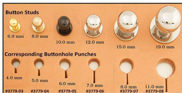
Figure 5.16. Différentes tailles de boutons de col avec la dimension du trou. ( www.stecksstore.com )
