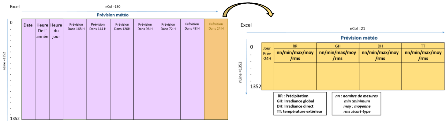
Figure 34: Structure des données de prévision météorologique
