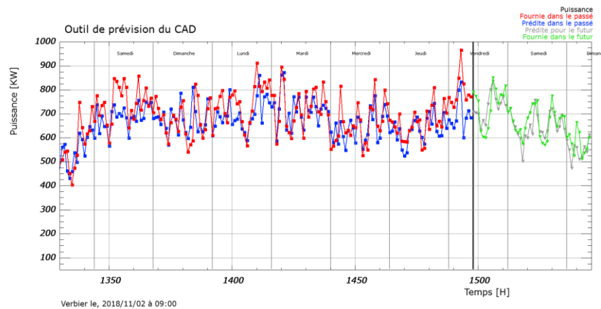
Figure 31: Modèle "météo réelle", h_{\text{Actuel}}=1498
