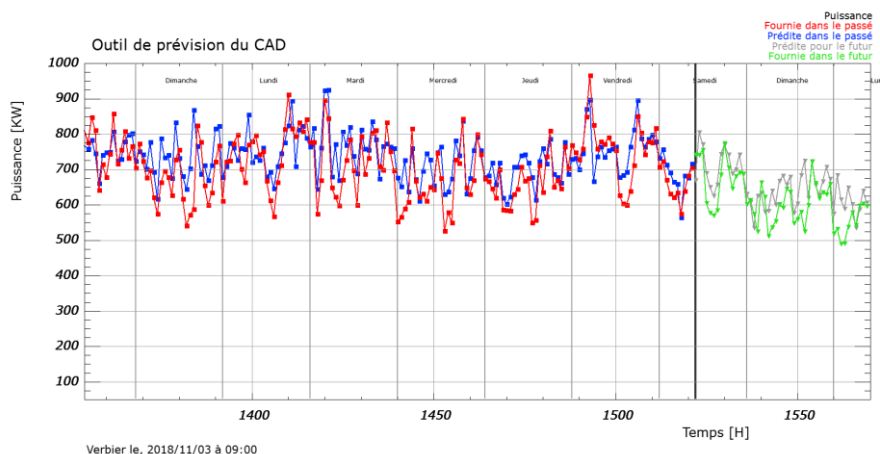
Figure 32: Modèle "météo réelle", h_{\text{Actuel}} = 1522
