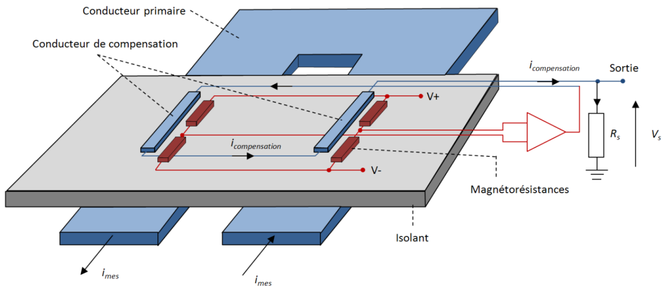
Figure II.12 : Schéma de principe d'un capteur magnéto résistif monté en pont de Wheatstone et opérant en boucle fermée.
