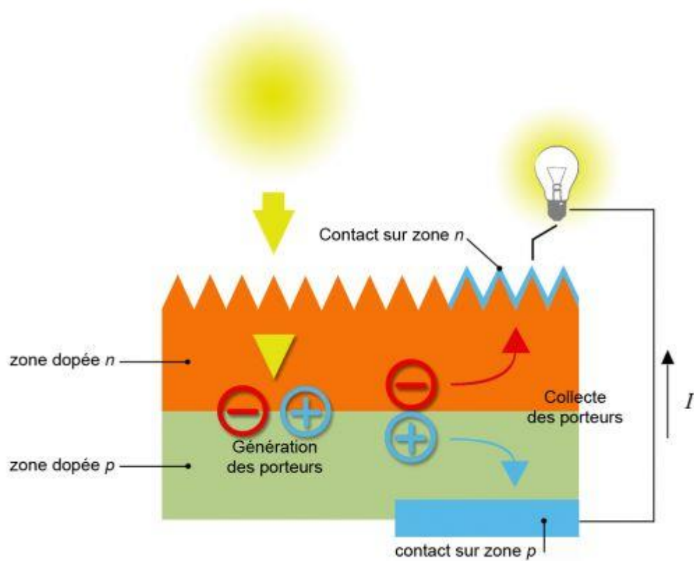
Figure I.6 Constitution d'une cellule photovoltaïque
