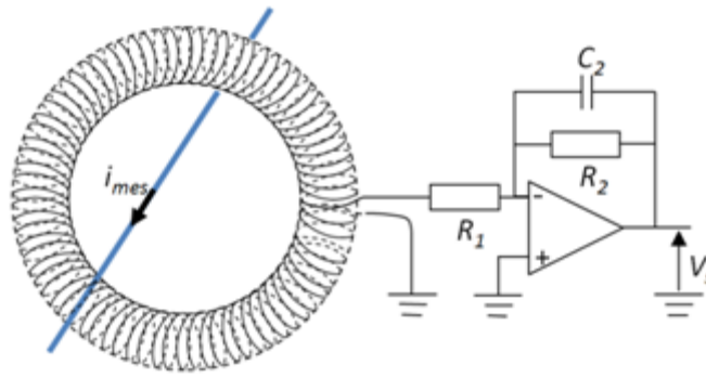
Figure II.9 : Schéma de principe d'une bobine de Rogowski munie d'un intégrateur
