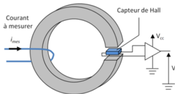
Figure II.10 : Schéma de principe d'un capteur de Hall
