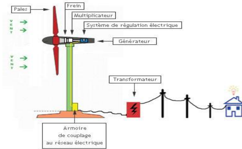
Figure I.5 parc éolienne
