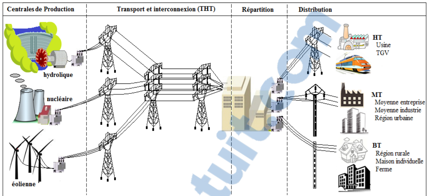
Figure I.7 transport et distribution de l'énergie électrique
