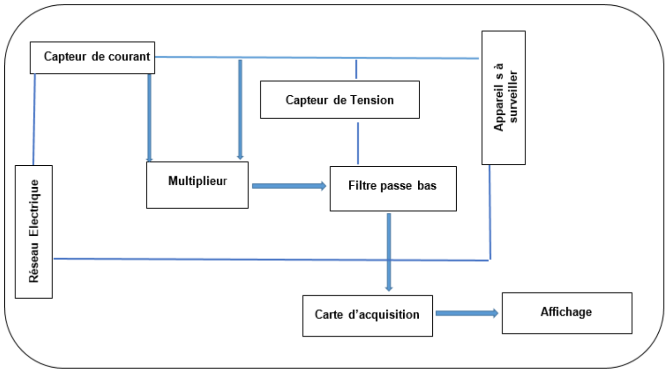
Figure II.6 : schéma synoptique d'un compteur d'energie
