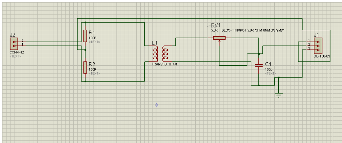
Figure III.4: schéma électrique de capteur de tension réaliser par Isis
