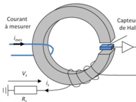
Figure II.11 : Schéma de principe d'un capteur de Hall en boucle fermée
