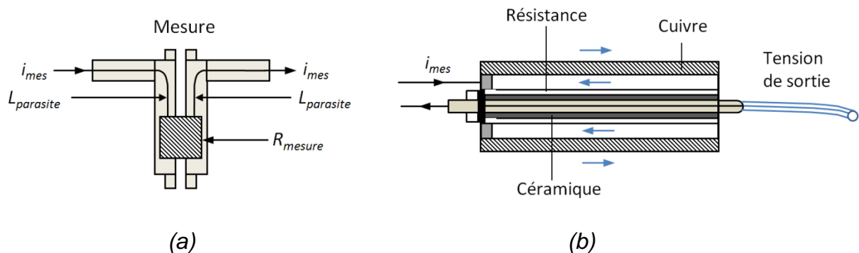
Figure II.7 : Schémas de principe (a) shunt en technologie couches épaisses et (b) shunt coaxial.
