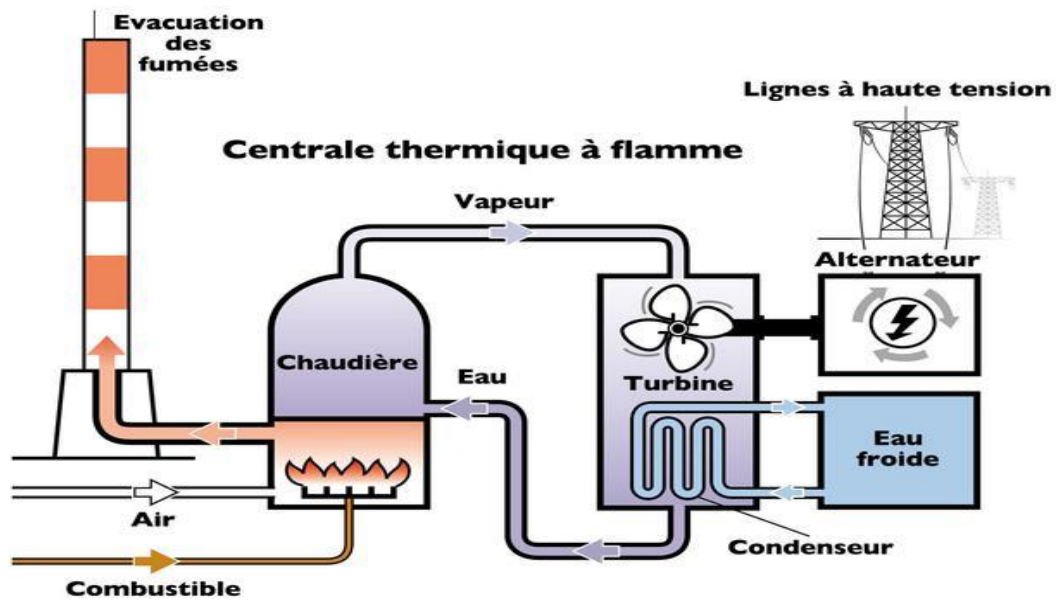
Figure I.3 centrale thermique
