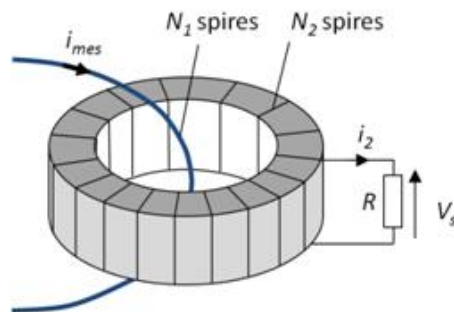
Figure II.8 : Schéma de principe d'un transformateur de courant.
