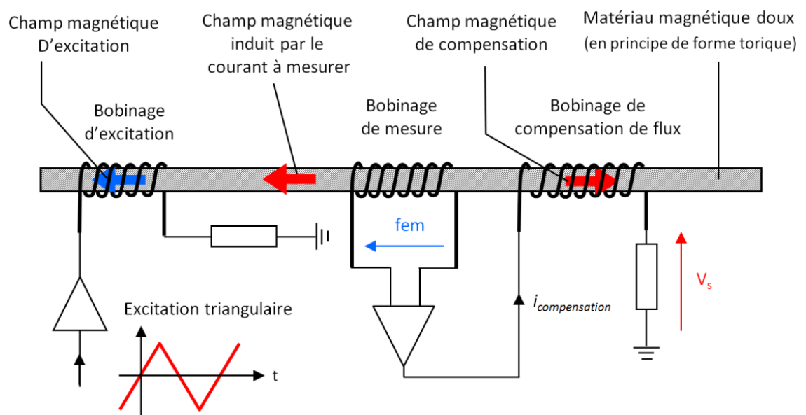
Figure II.13 : Schéma de principe d'un capteur fluxgate opérant à flux nul (boucle fermée)
