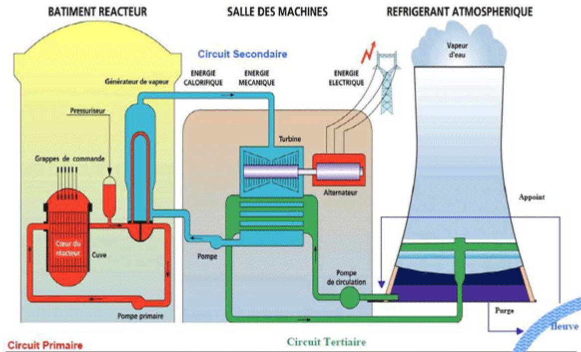
FigureI.4 centrale nucléaire
