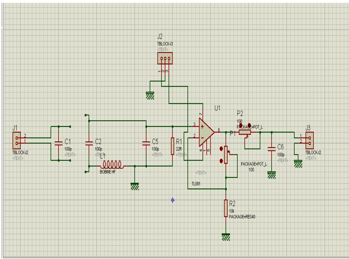
Figure III.1: schéma électrique d'un capteur de courant réaliser par Isis
