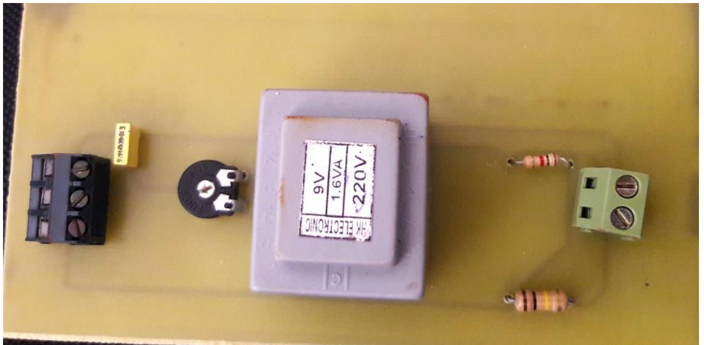
Figure III.6: circuit électrique de capteur de tension
