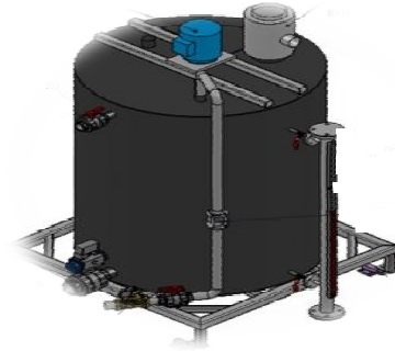
Figure n°7 : Bac de préparation des sels
